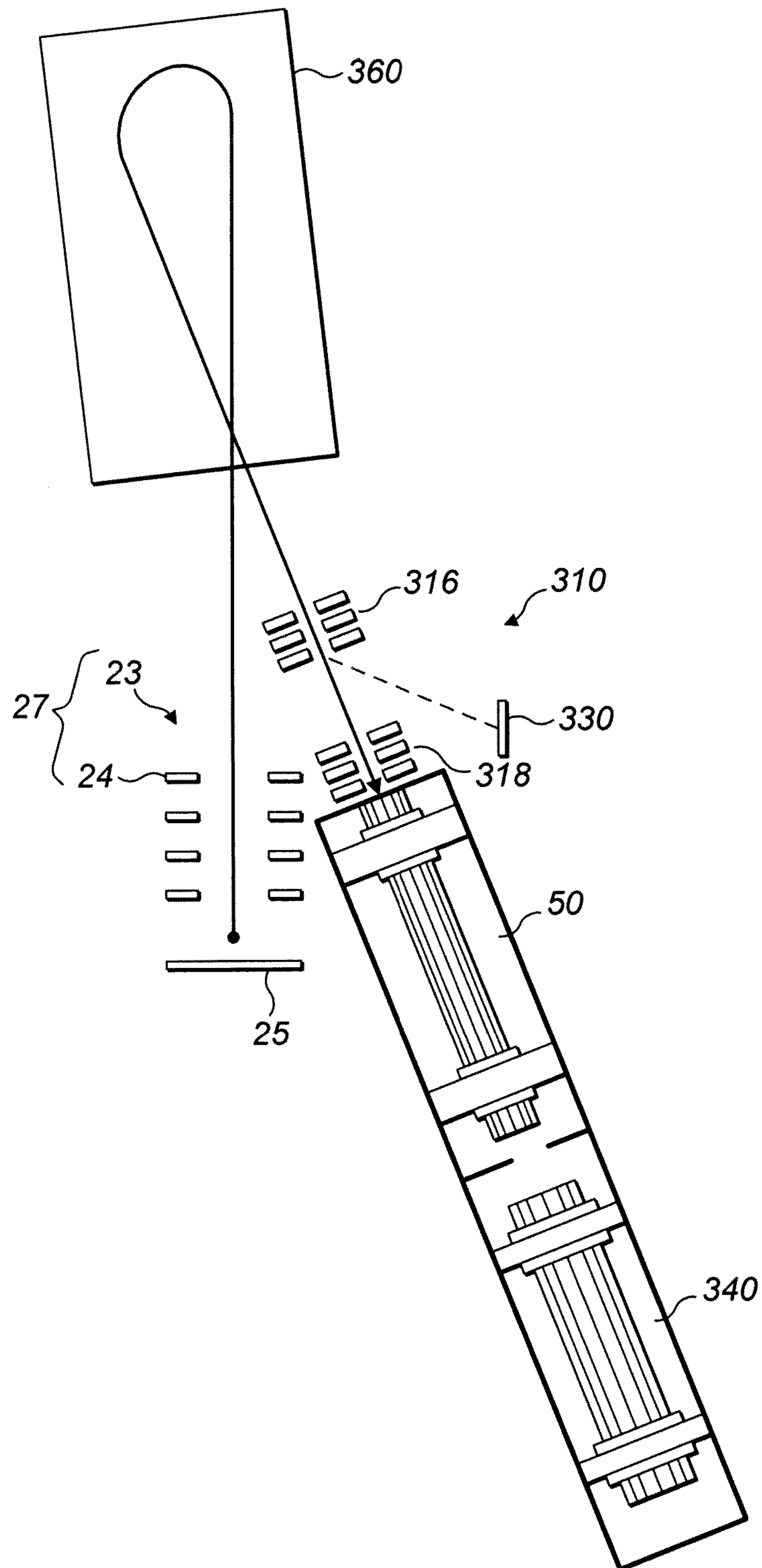
FIG. 7b
