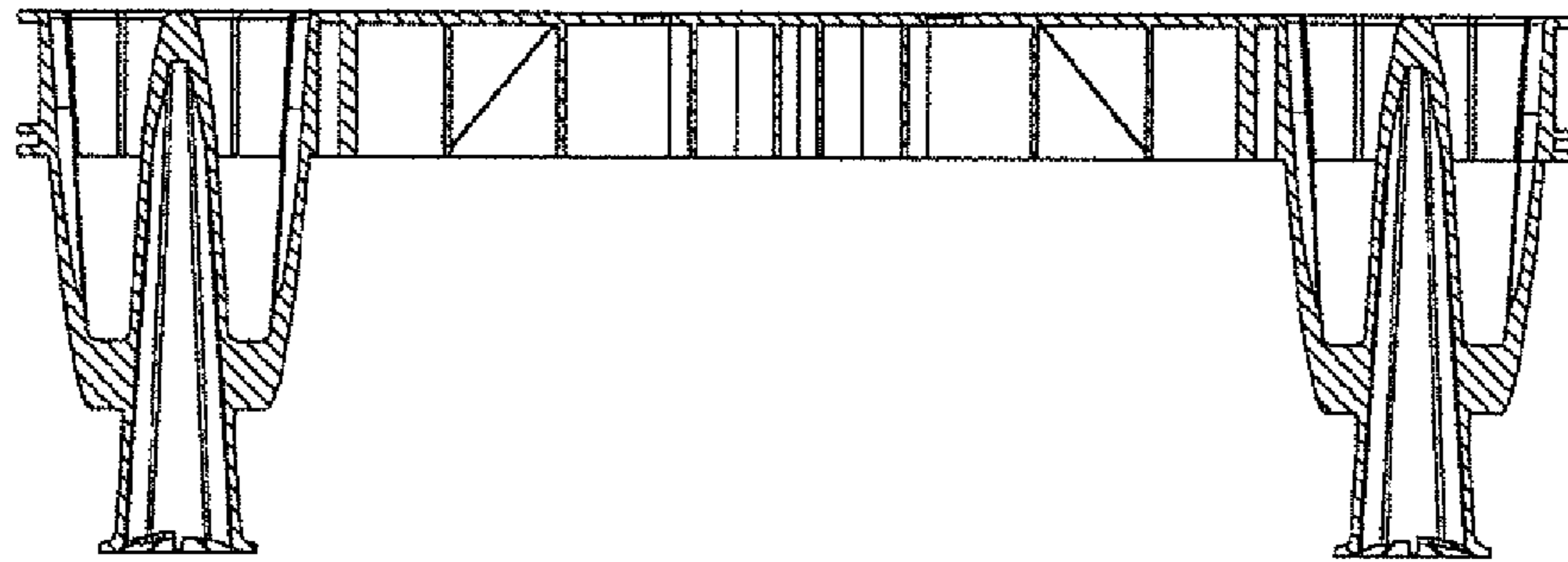
Fig. 80 Section A-A
