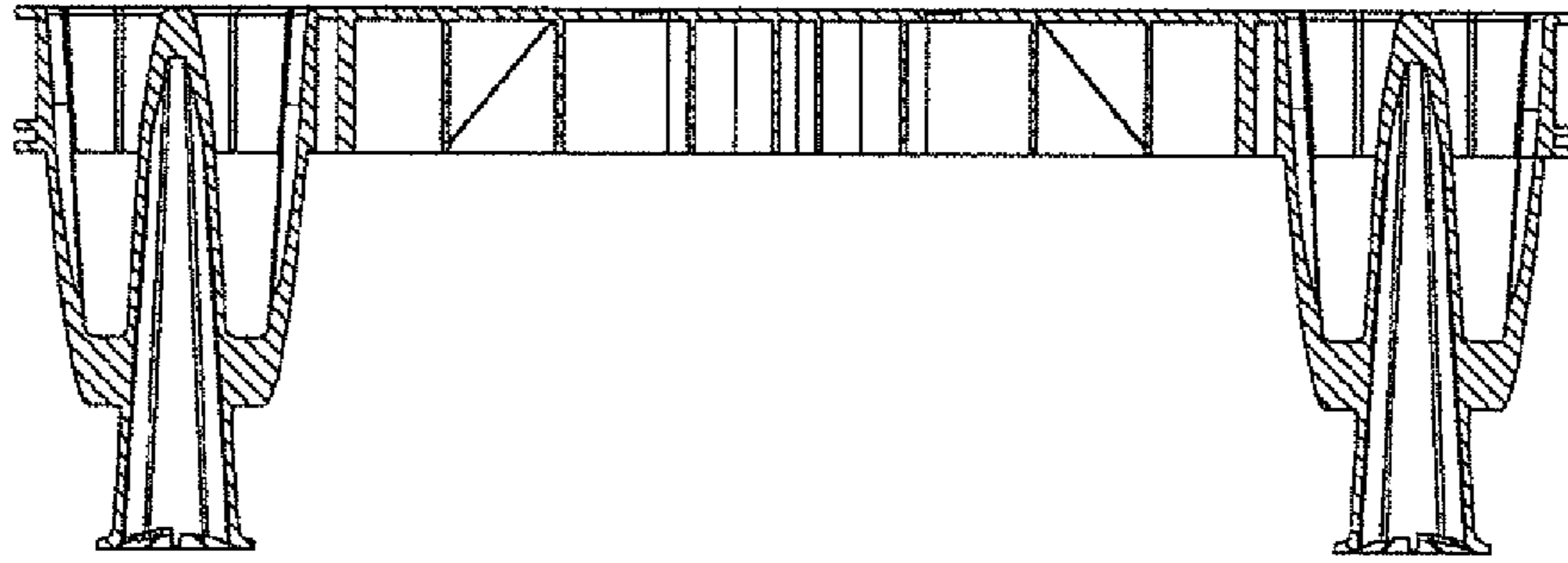
Fig. 80 Section A-A
