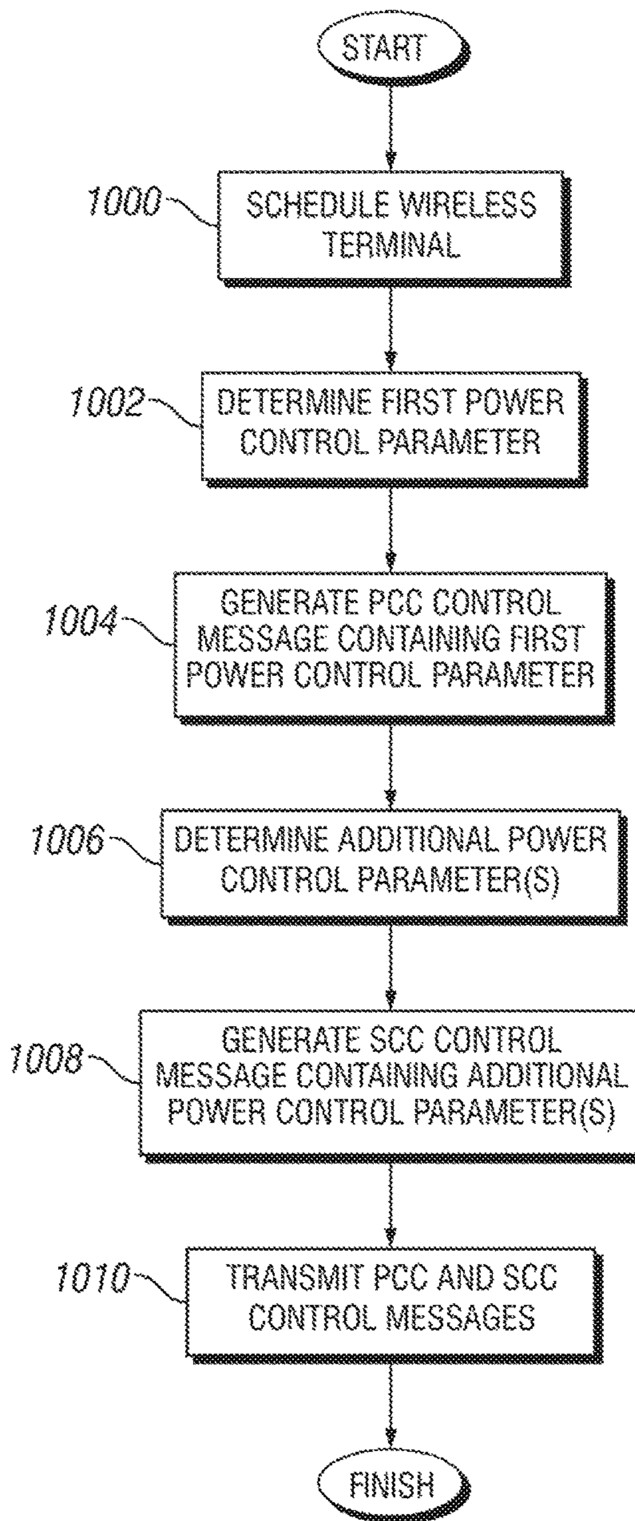
FIG. 10
