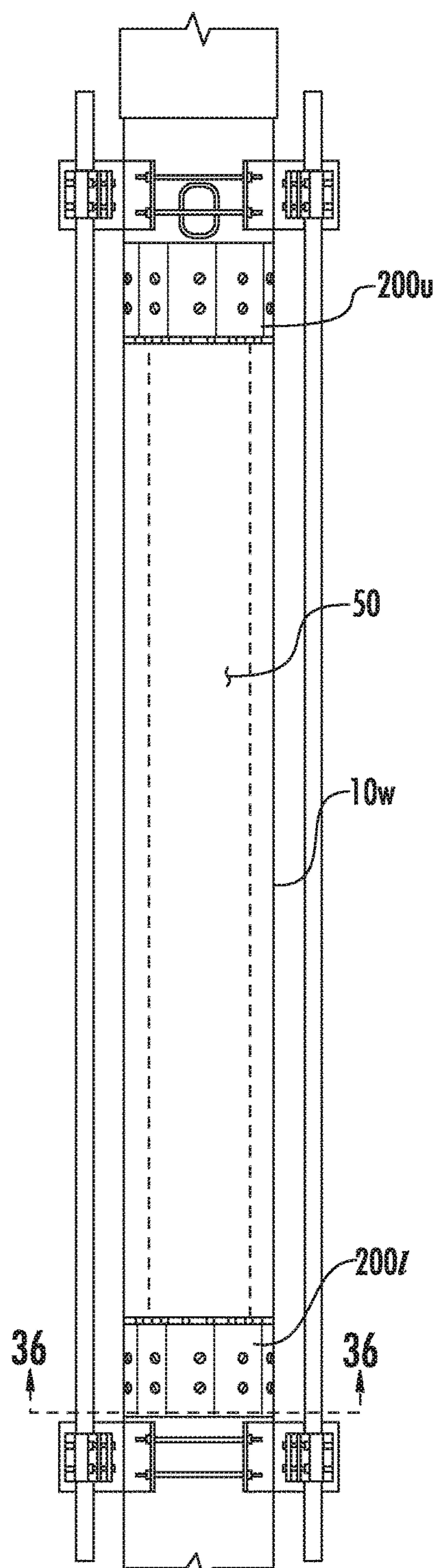
BOTTOM INSTALL STEP 4 FIG. 34
