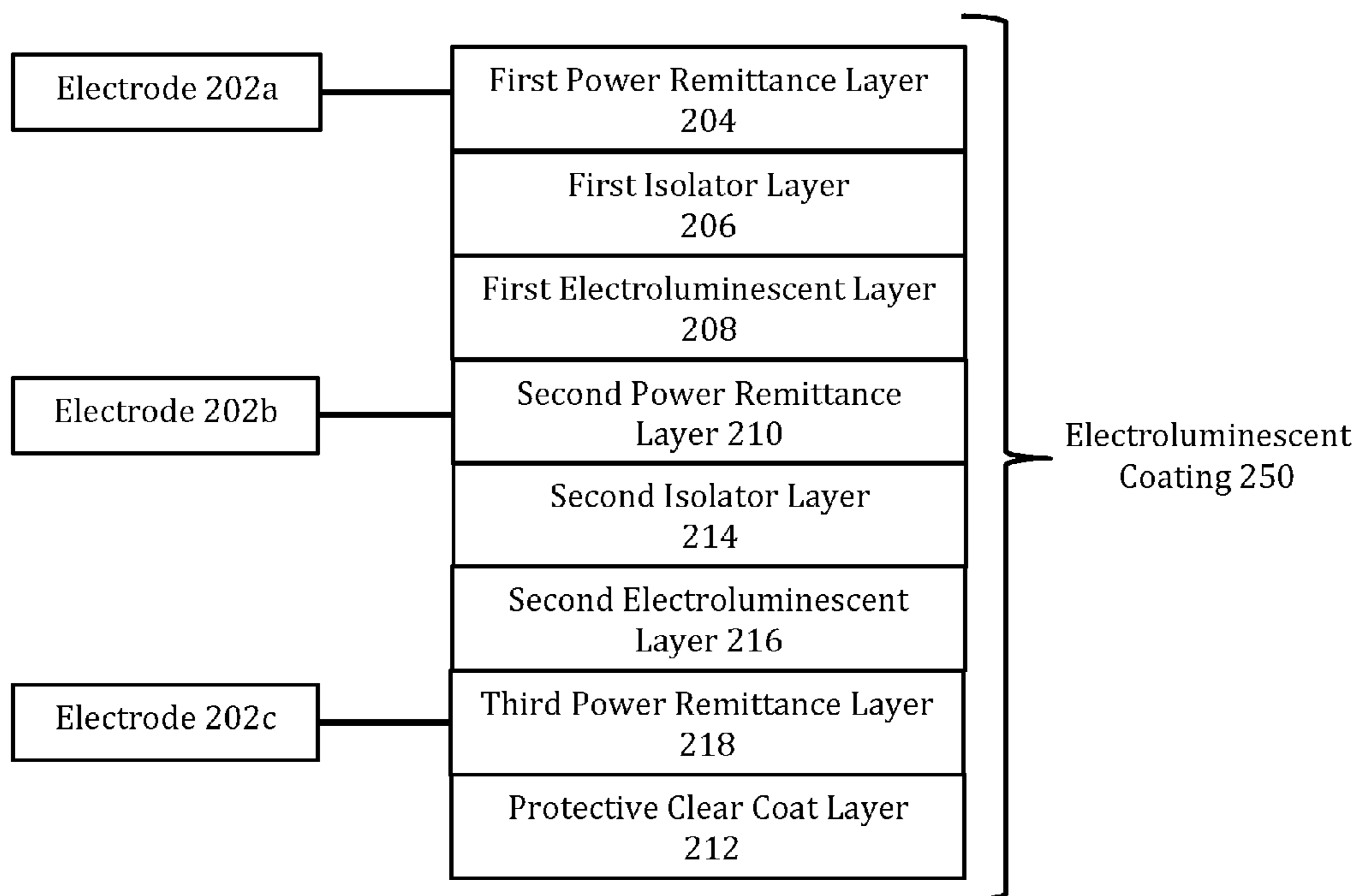
FIG. 2B
