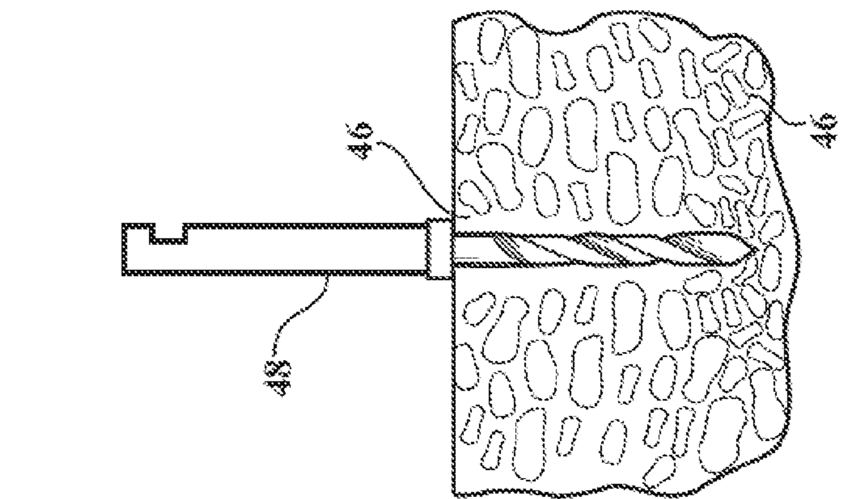
FIG. 24D
