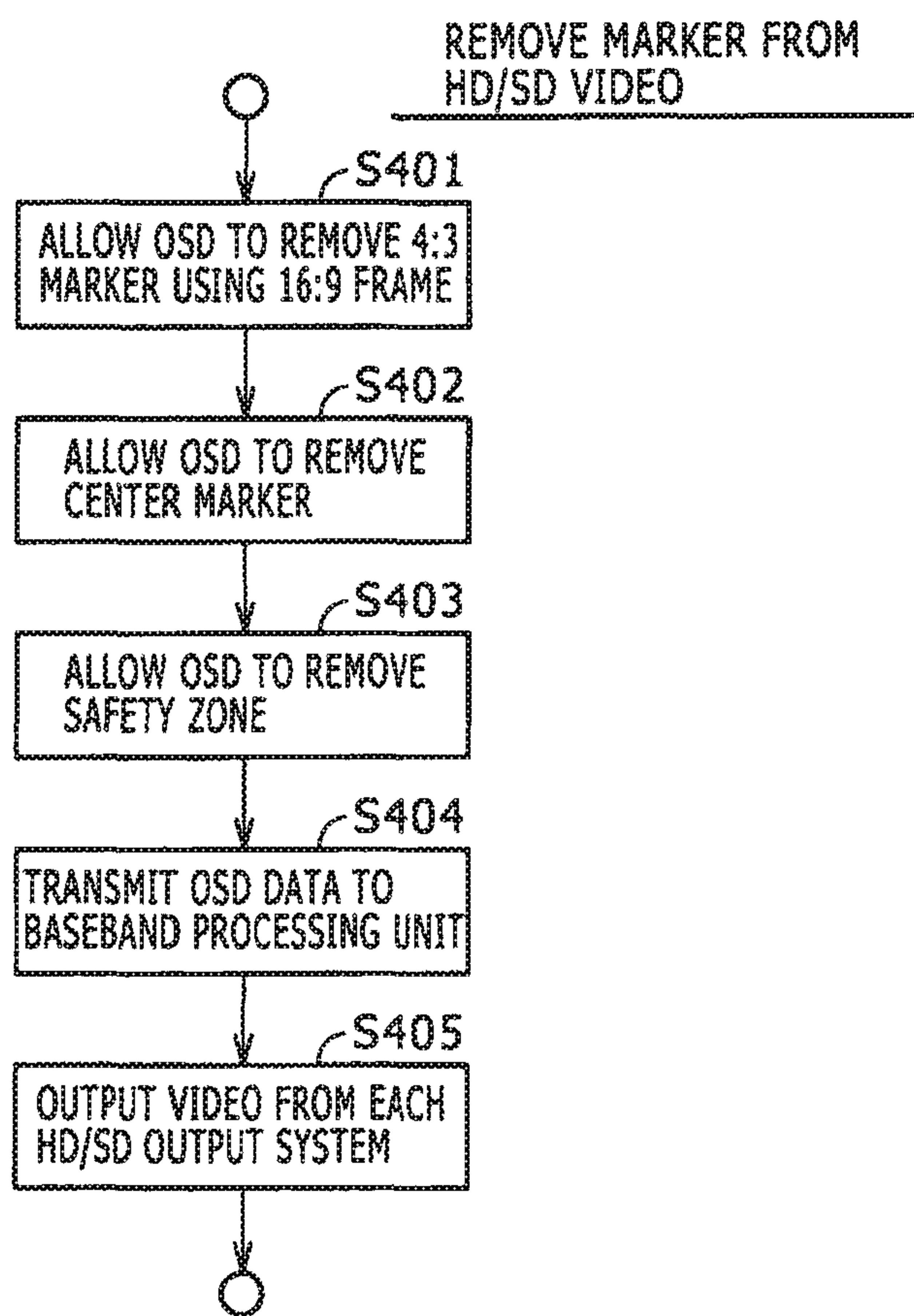
FIG. 11
