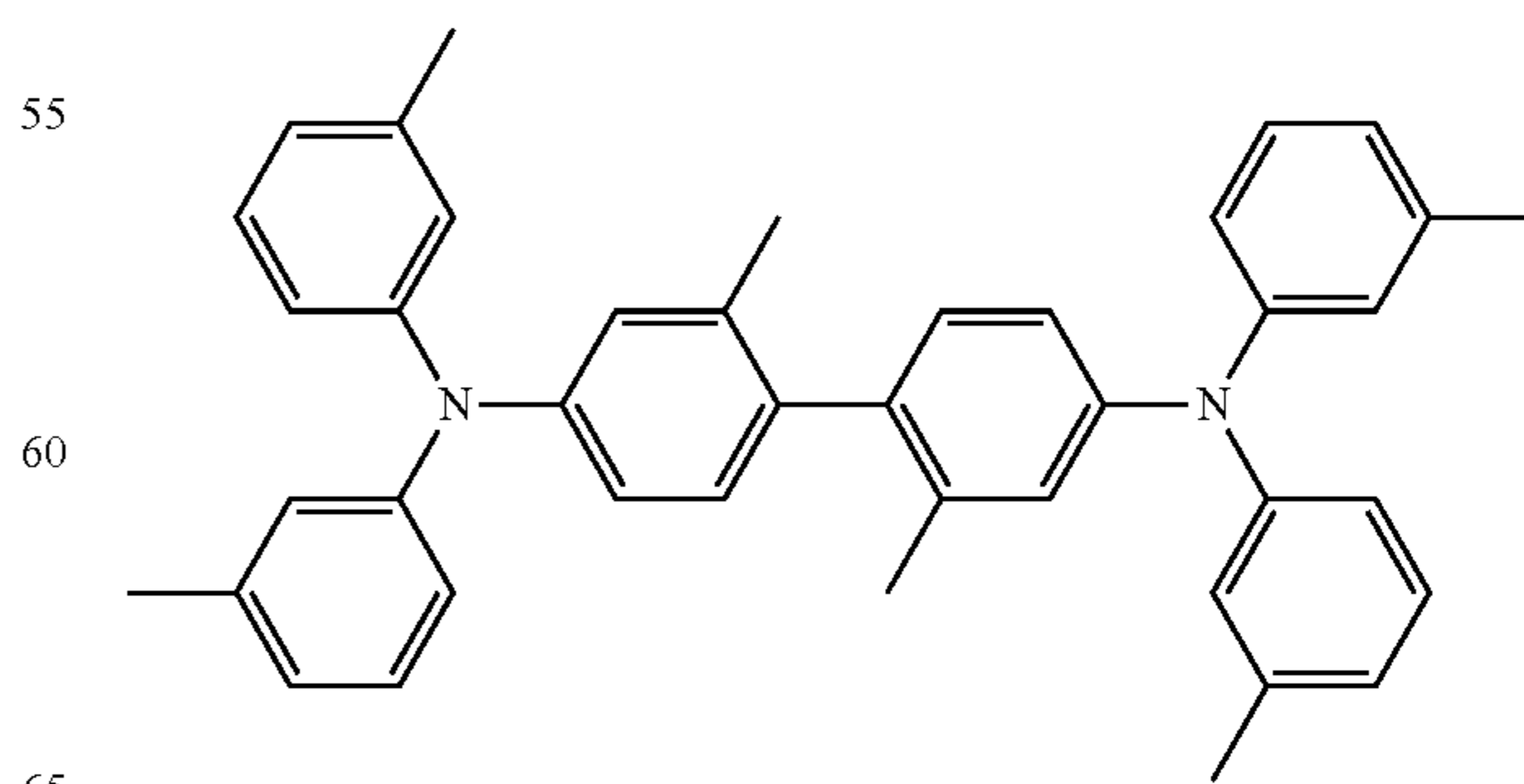
HMTPD
