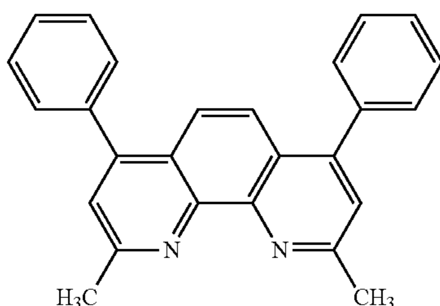
BCP
