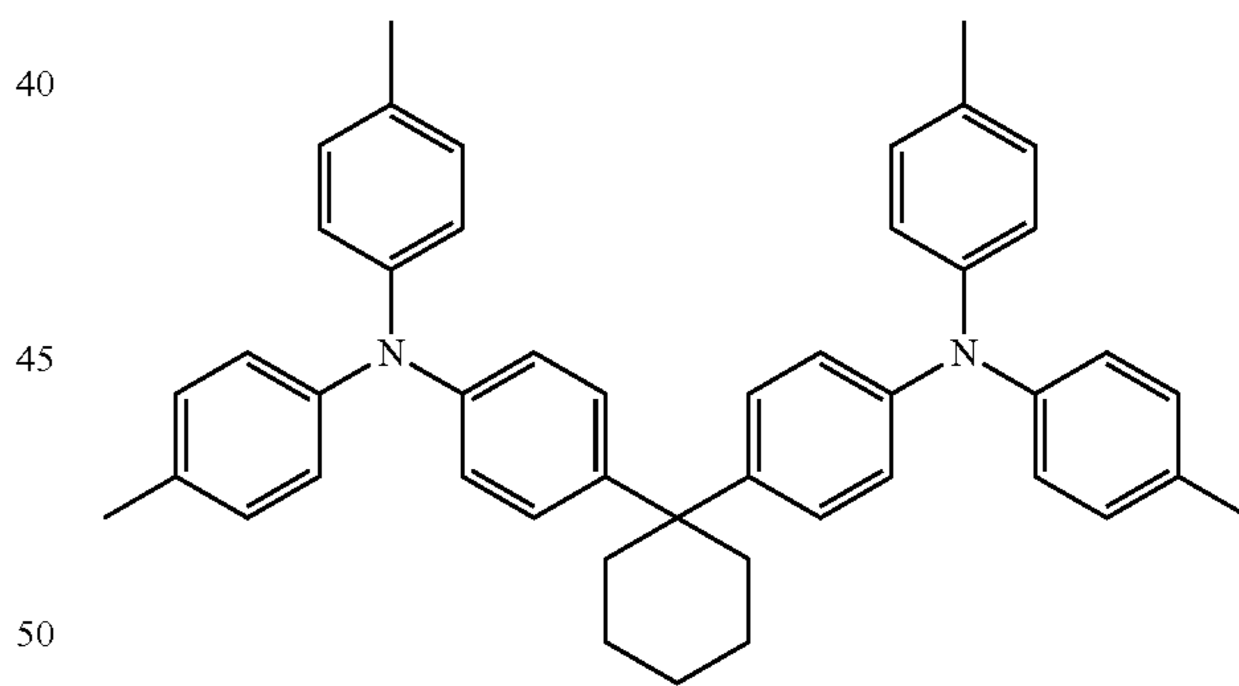
TAPC
