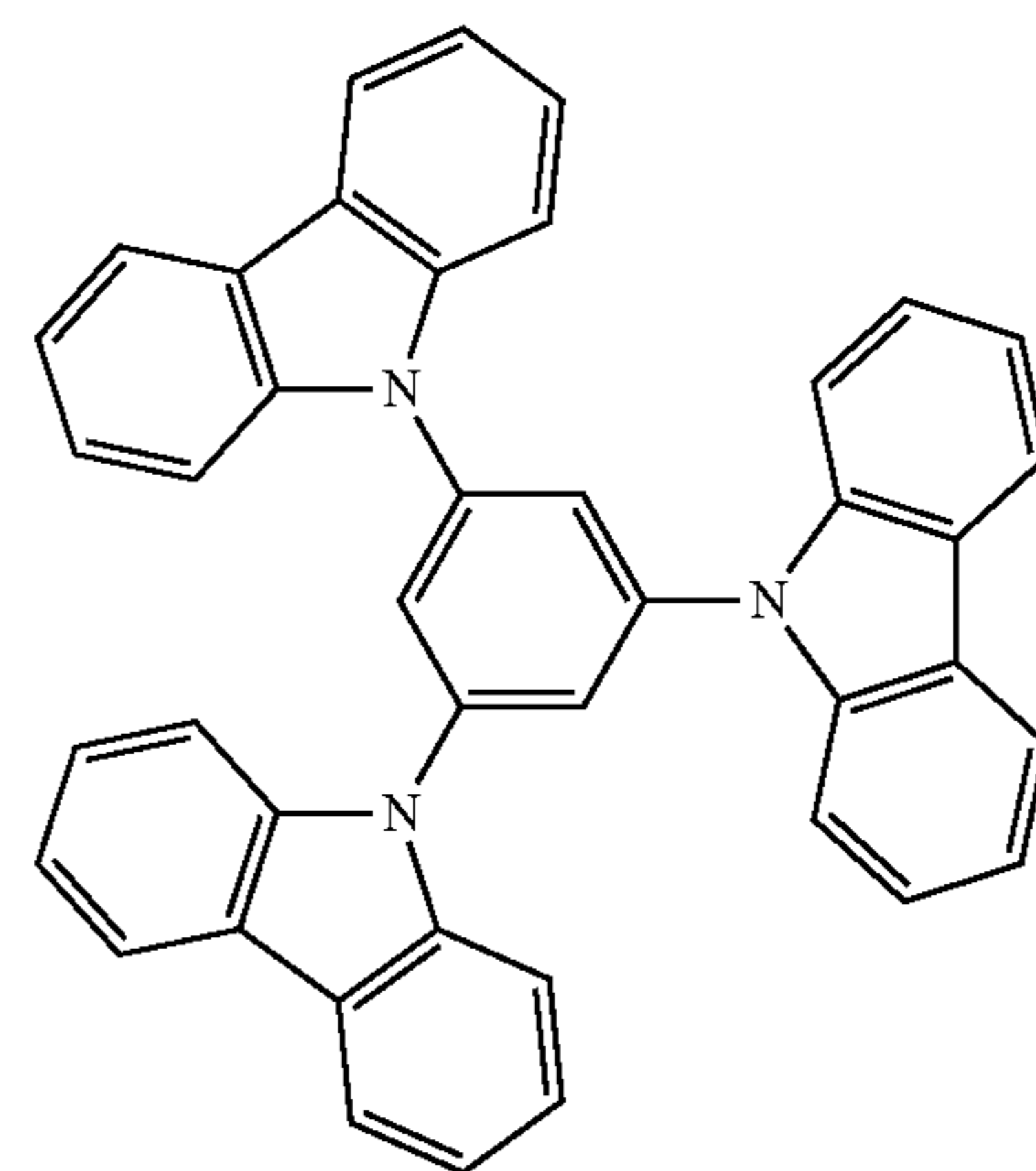
TCP
