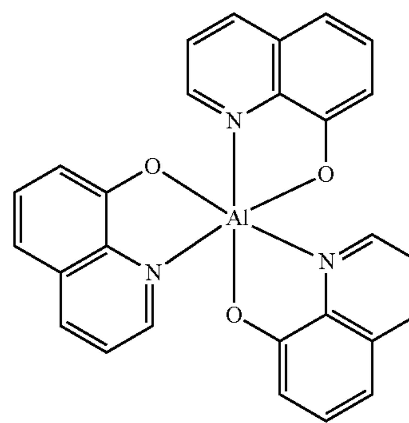
Alq 3
