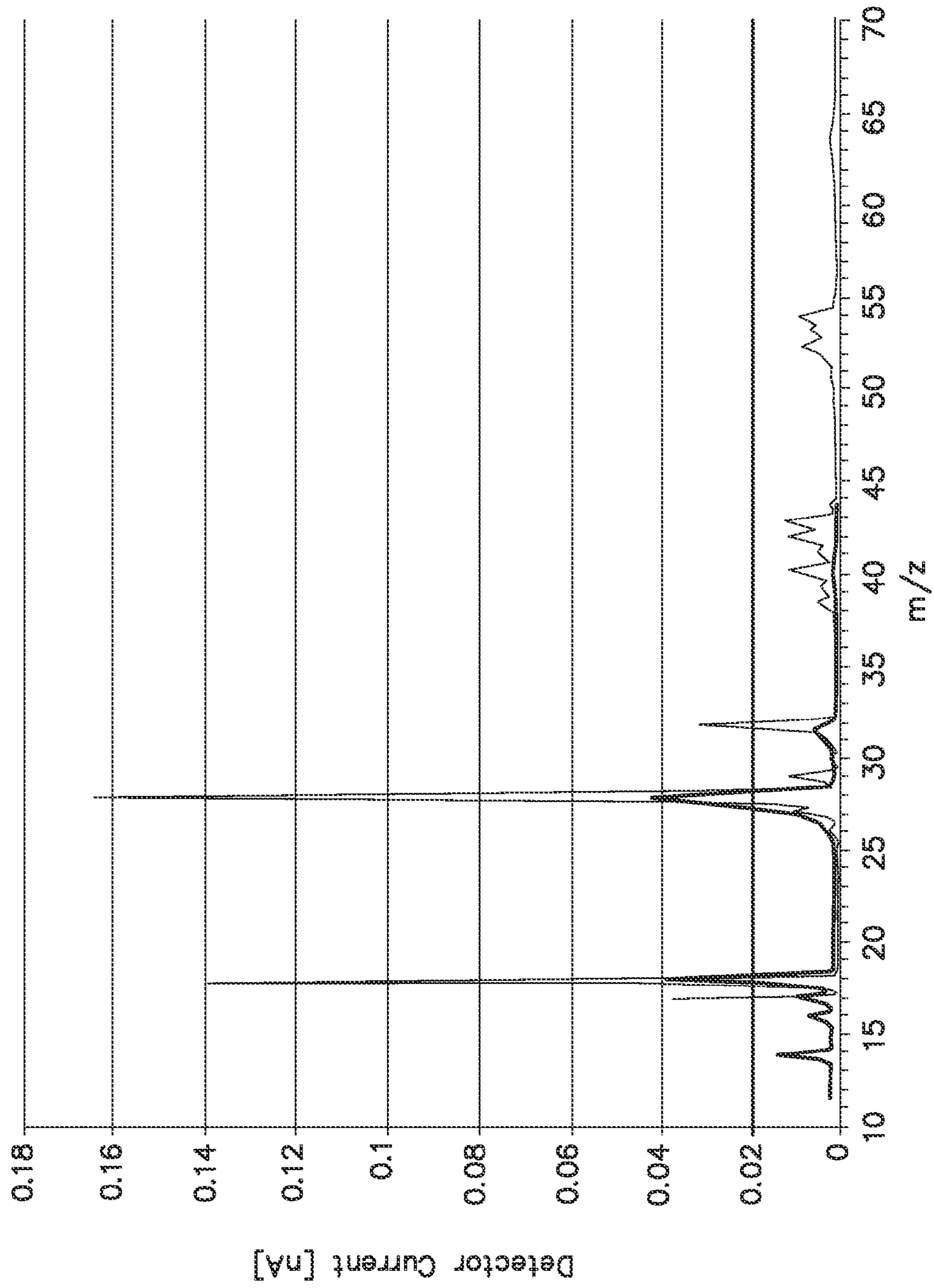
FIG. 30
