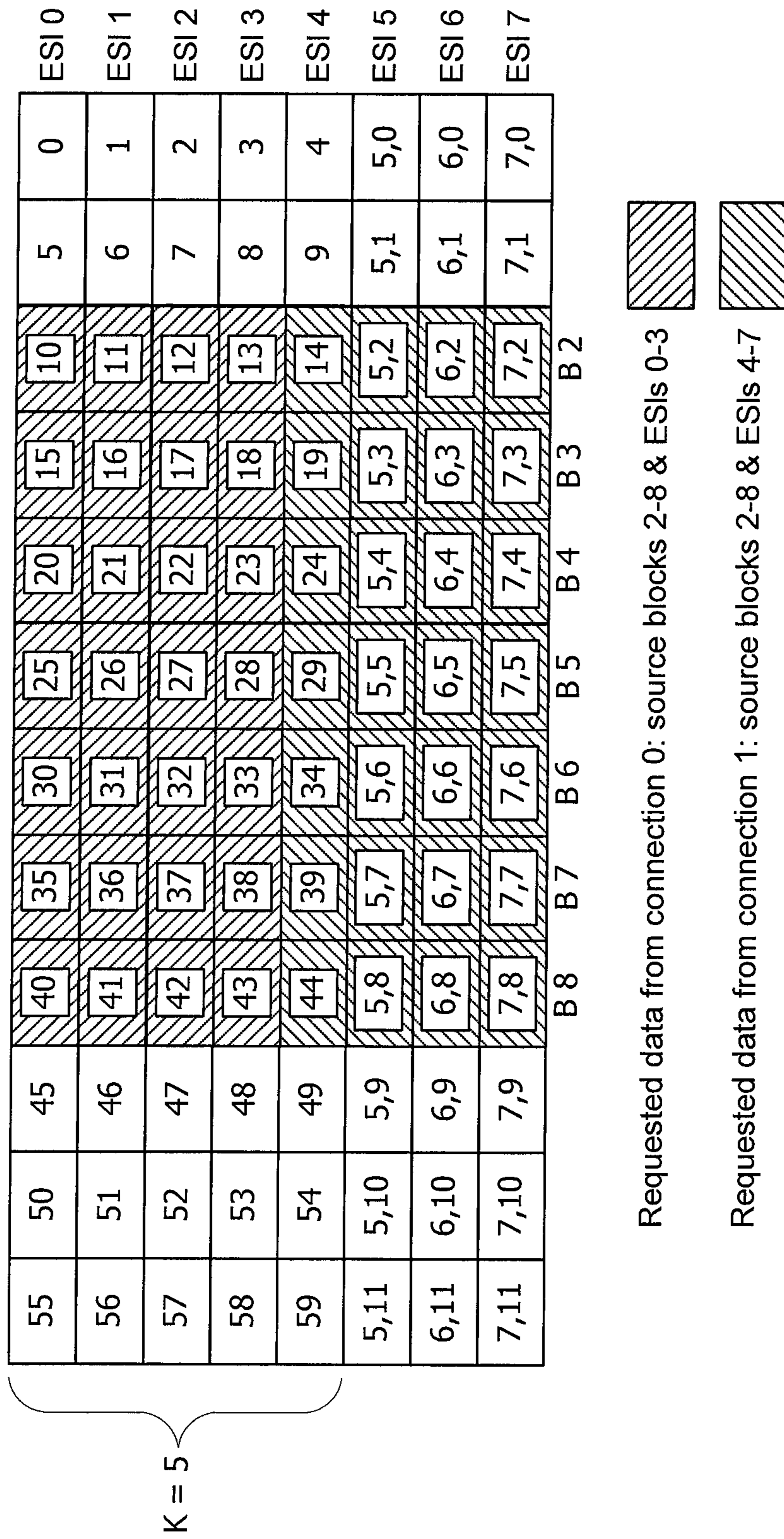
FIG. 14A
