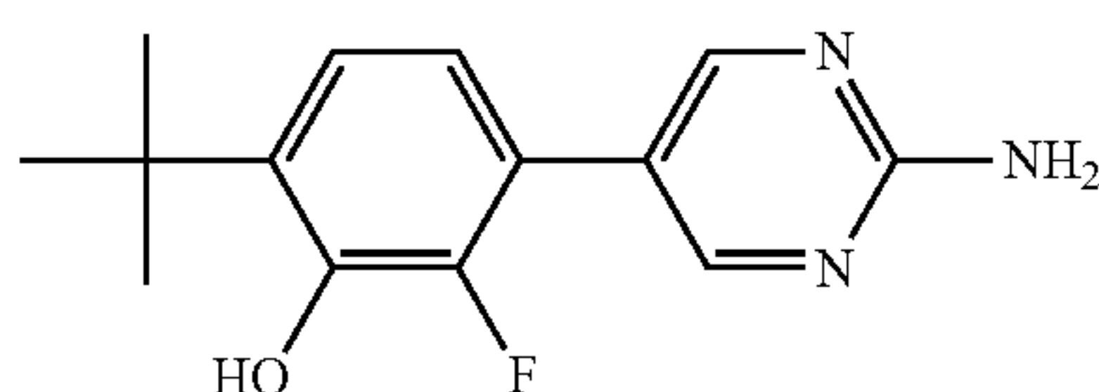
3-(2-Aminopyrimidin-5-yl)-6-tert-butyl-2-fluorophenol
