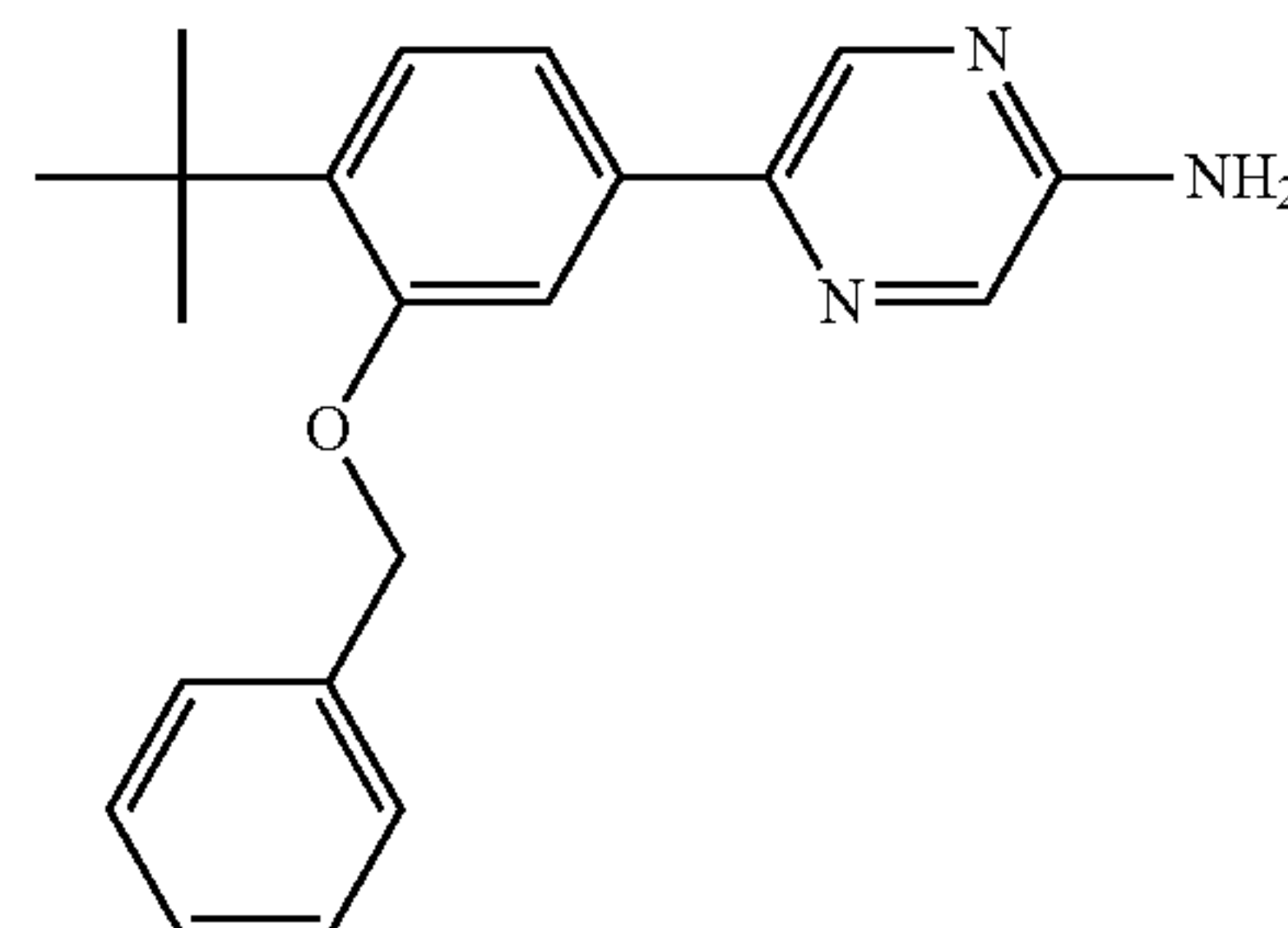
5-[3-(Benzyloxy)-4-tert-butylphenyl]pyrazin-2- amine
