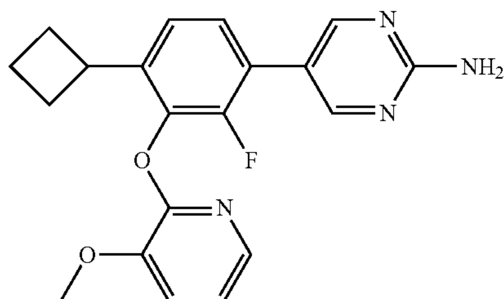
5-{4-Cyclobutyl-2-fluoro-3-[(3-methoxypyridin-2-yl)oxy]phenyl}pyrazin-2-amine
