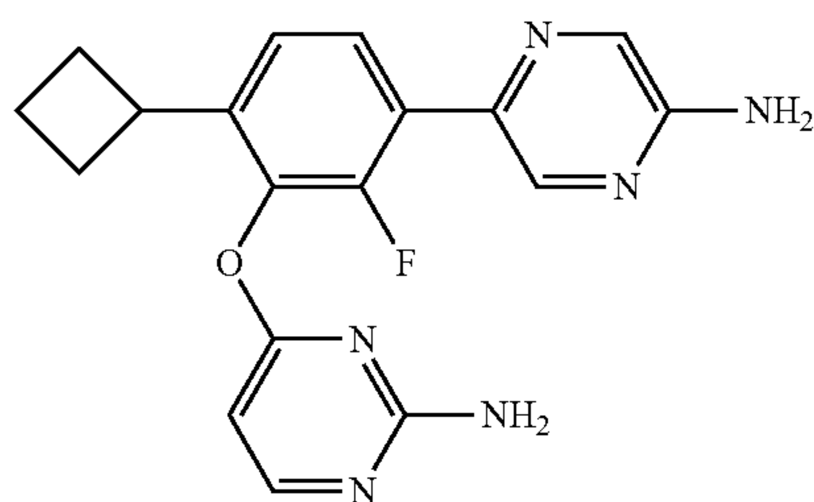
4-[3-(5-Aminopyrazin-2-yl)-6-cyclobutyl-2-fluorophenoxy]pyrimidin-2-amine
