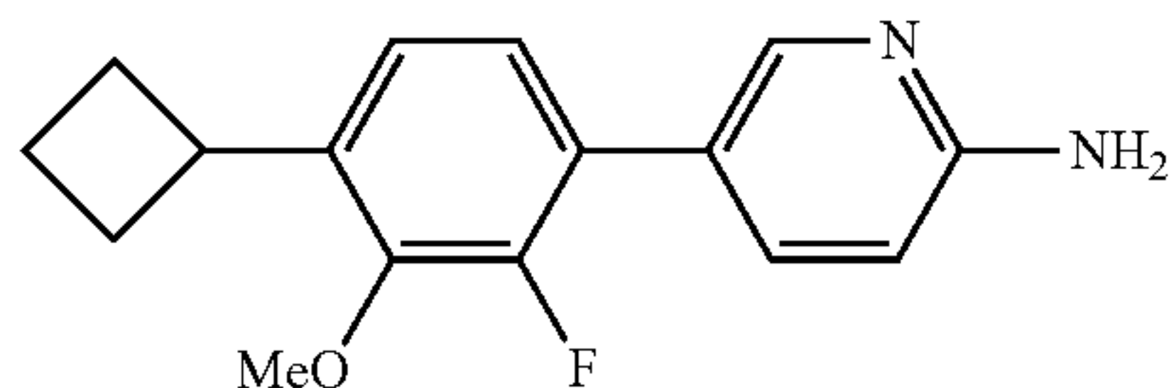
5-(4-Cyclobutyl-2-fluoro-3-methoxyphenyl)pyridin-2-amine hydrochloride salt
