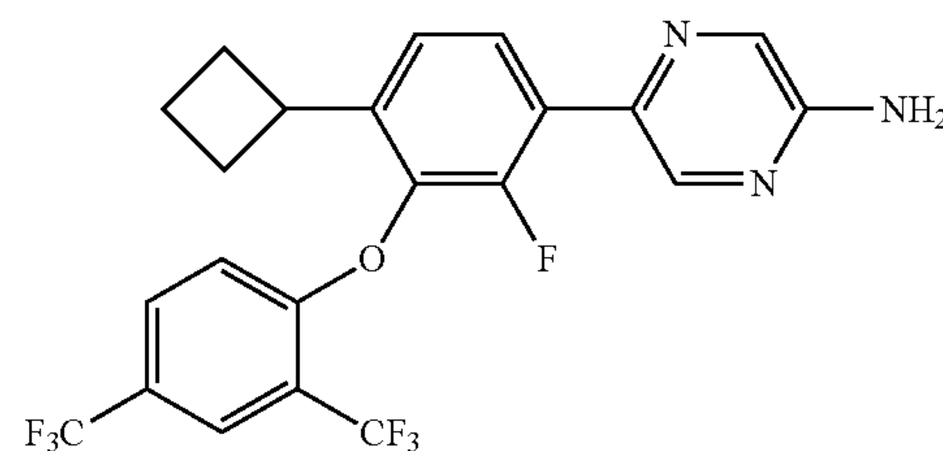
5-[3-[2,4-Bis(trifluoromethyl)phenoxy]-4-cyclobutyl-2-fluorophenyl]pyrazin-2-amine
