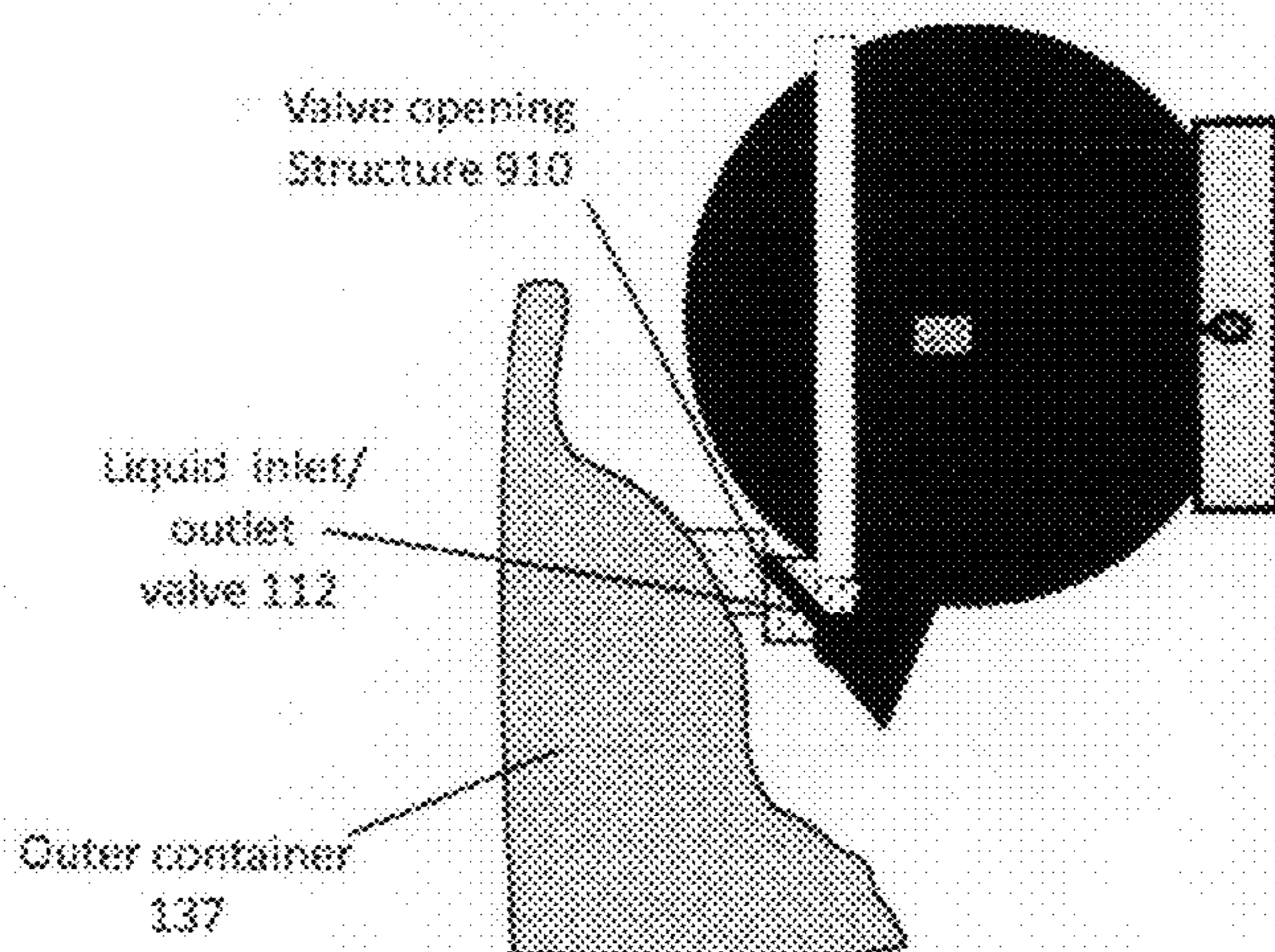
FIG. 9e: Valve Opening
