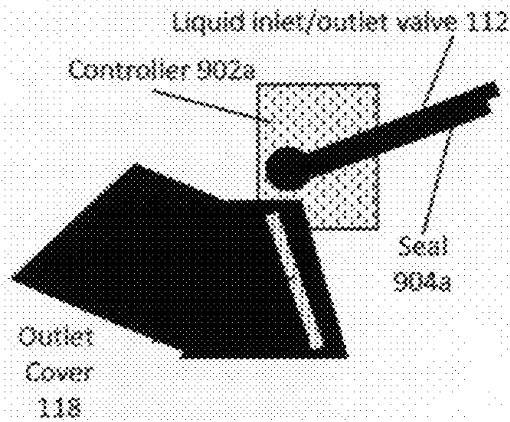
FIG. 9b: Inlet/Outlet valve open
