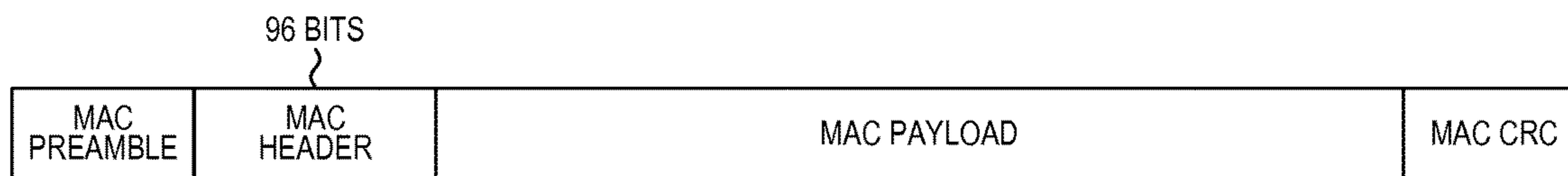
MAC FRAME (DATA MODE) FIG. 11
