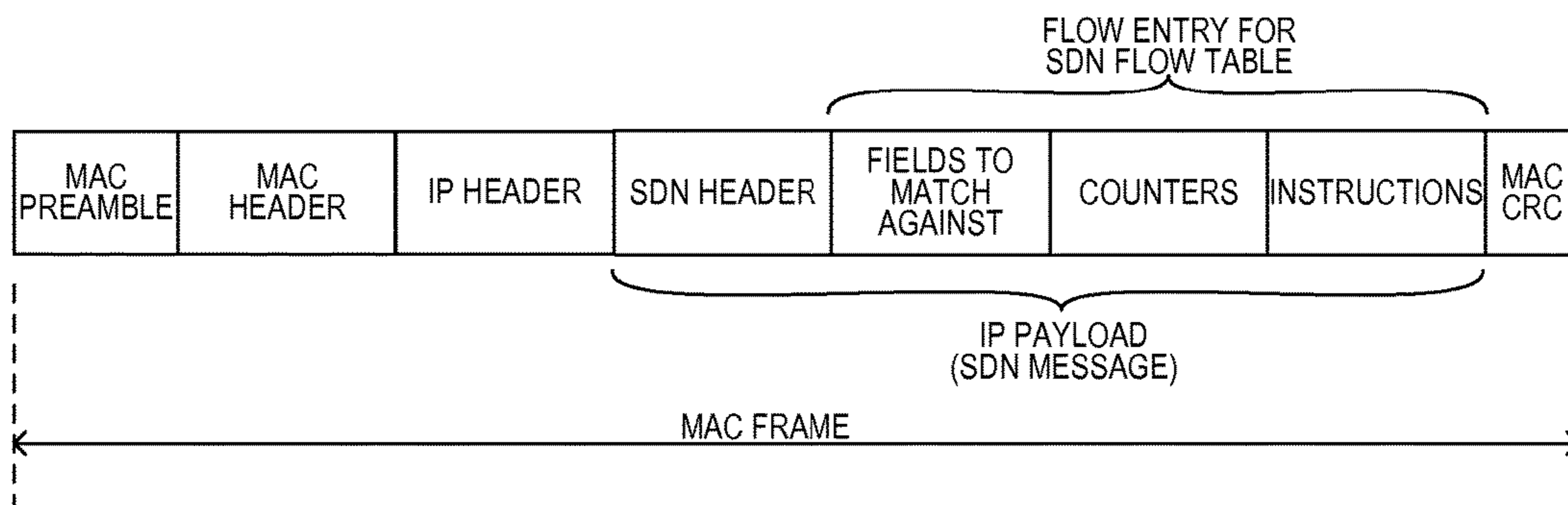
SDN MESSAGE FIG. 9
