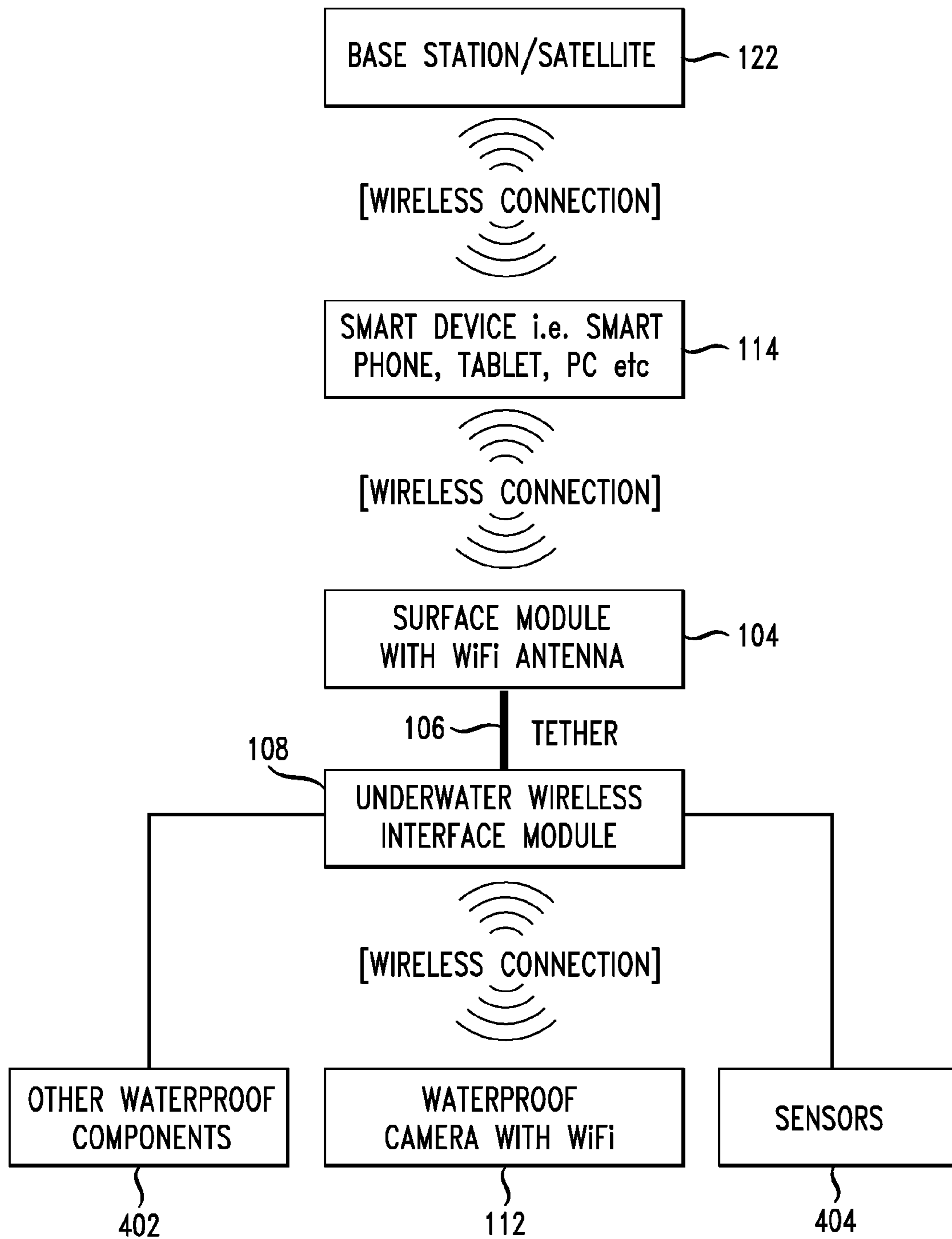
FIG. 4A
