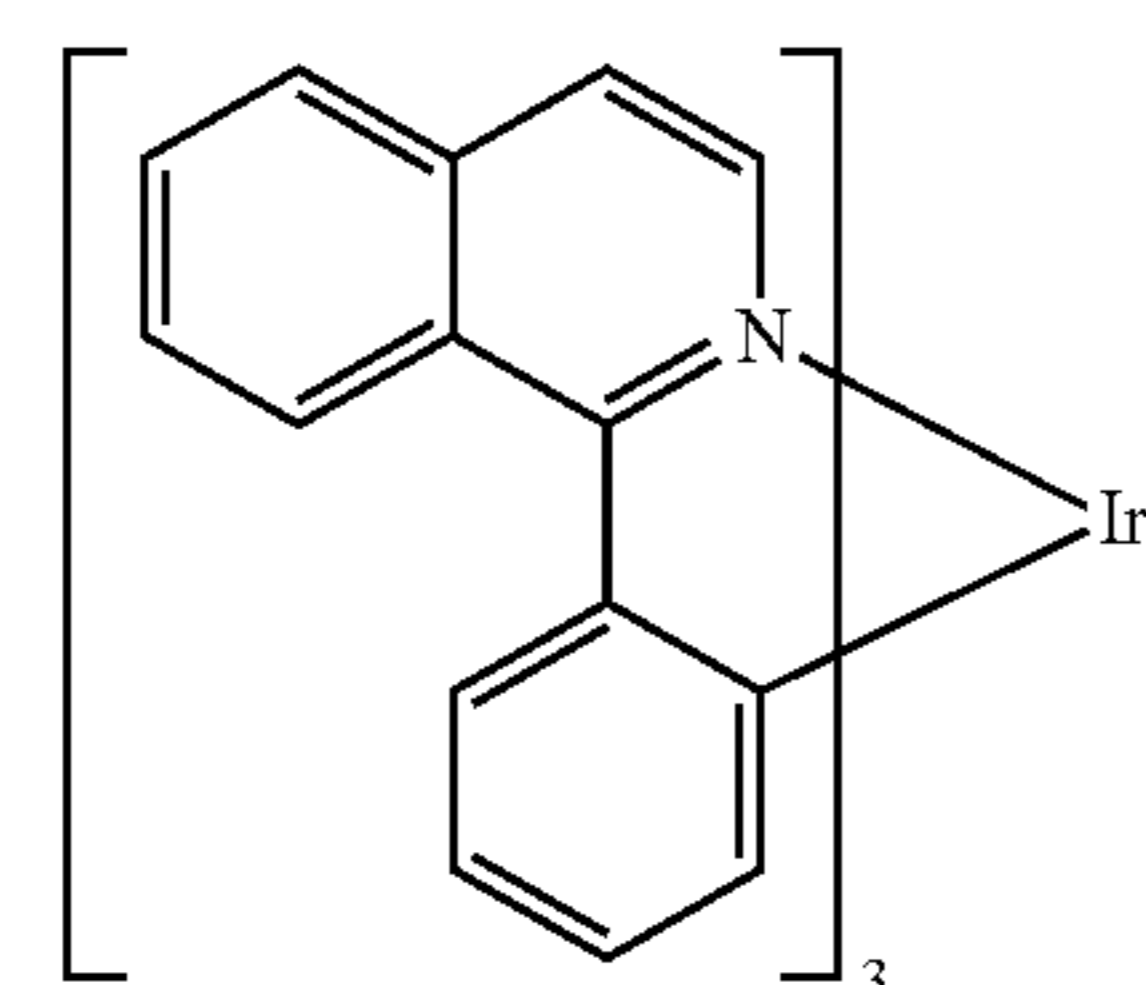
[Ir(piq) 3 ]
