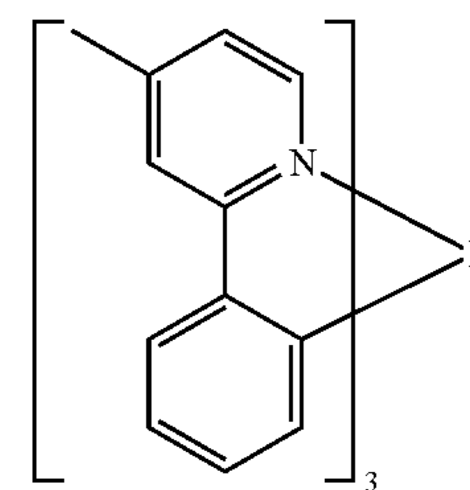
[Ir(mpyp) 3 ]
