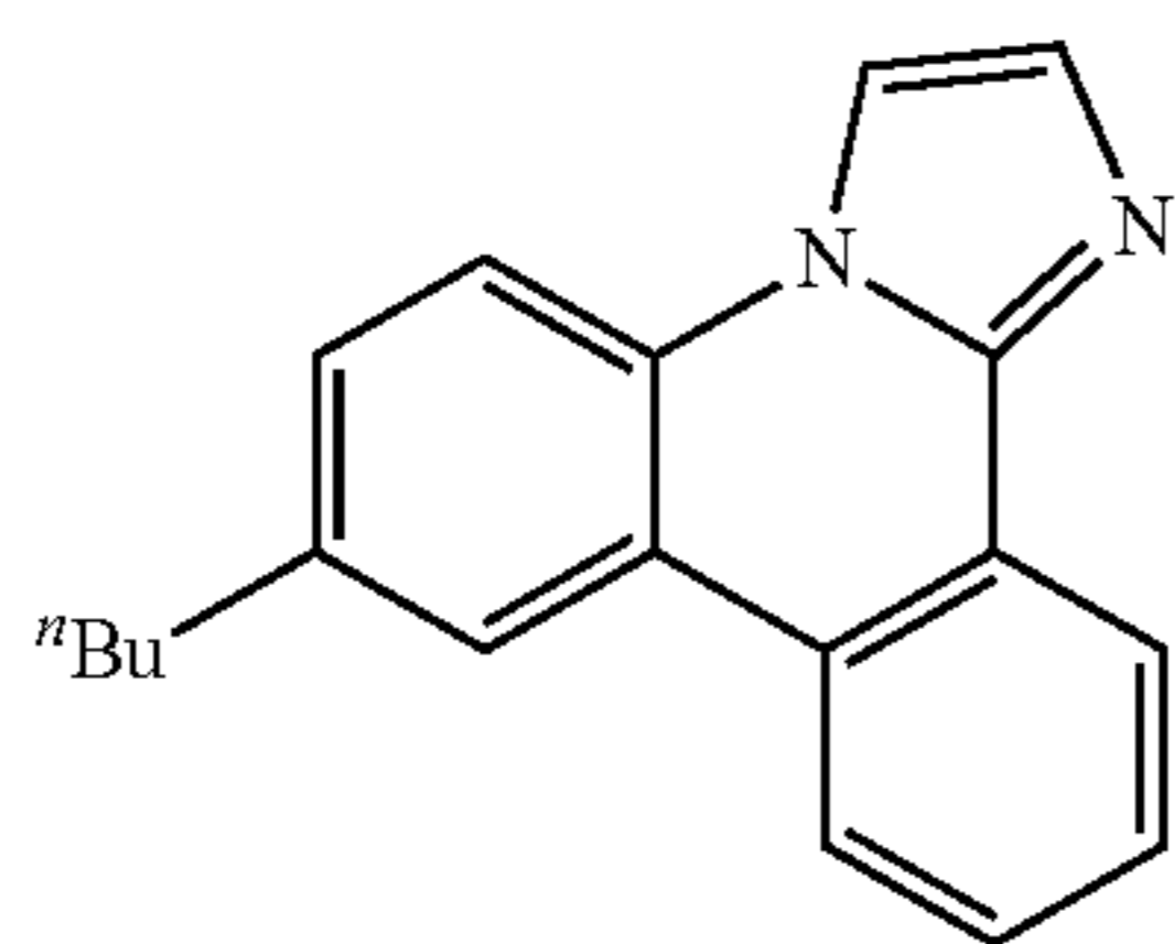
ligand
