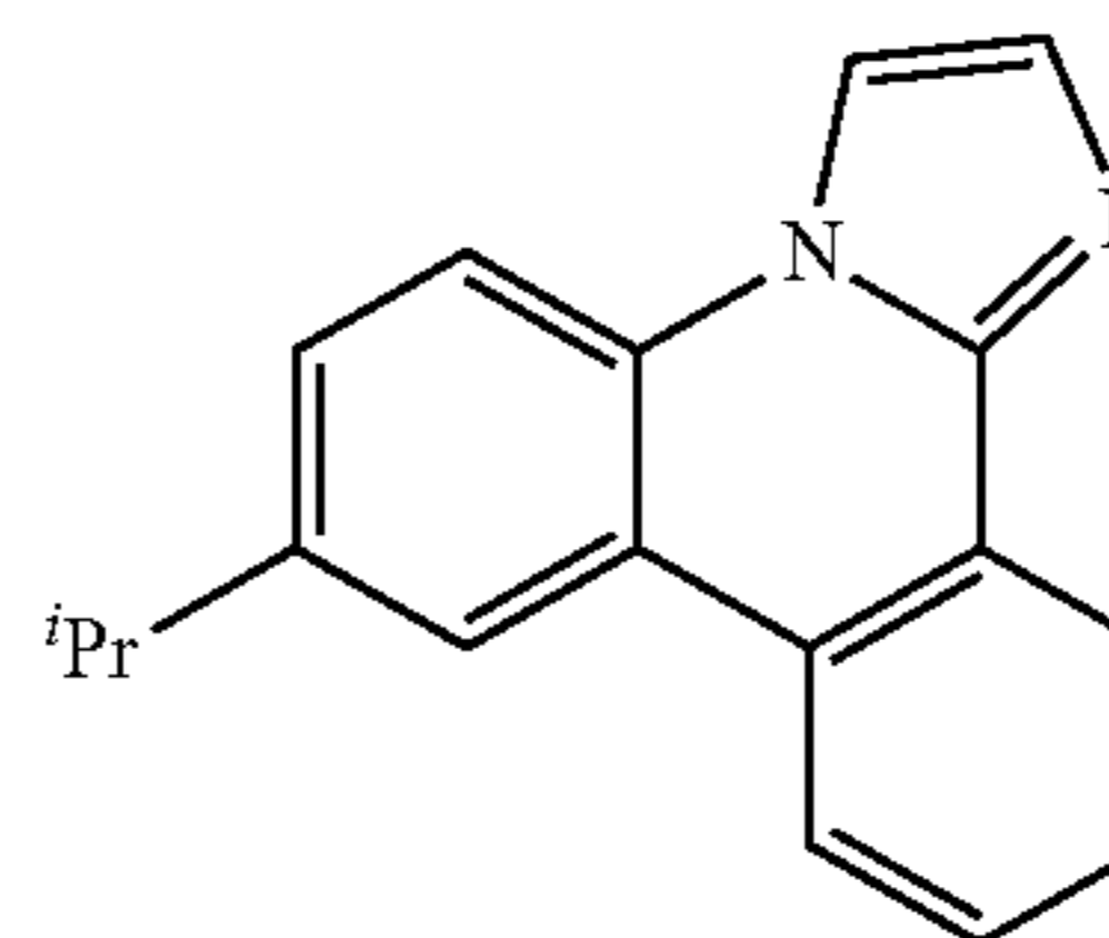
ligand
