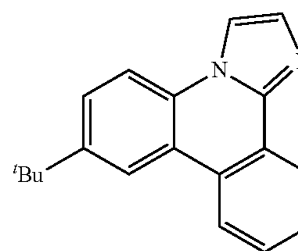
ligand
