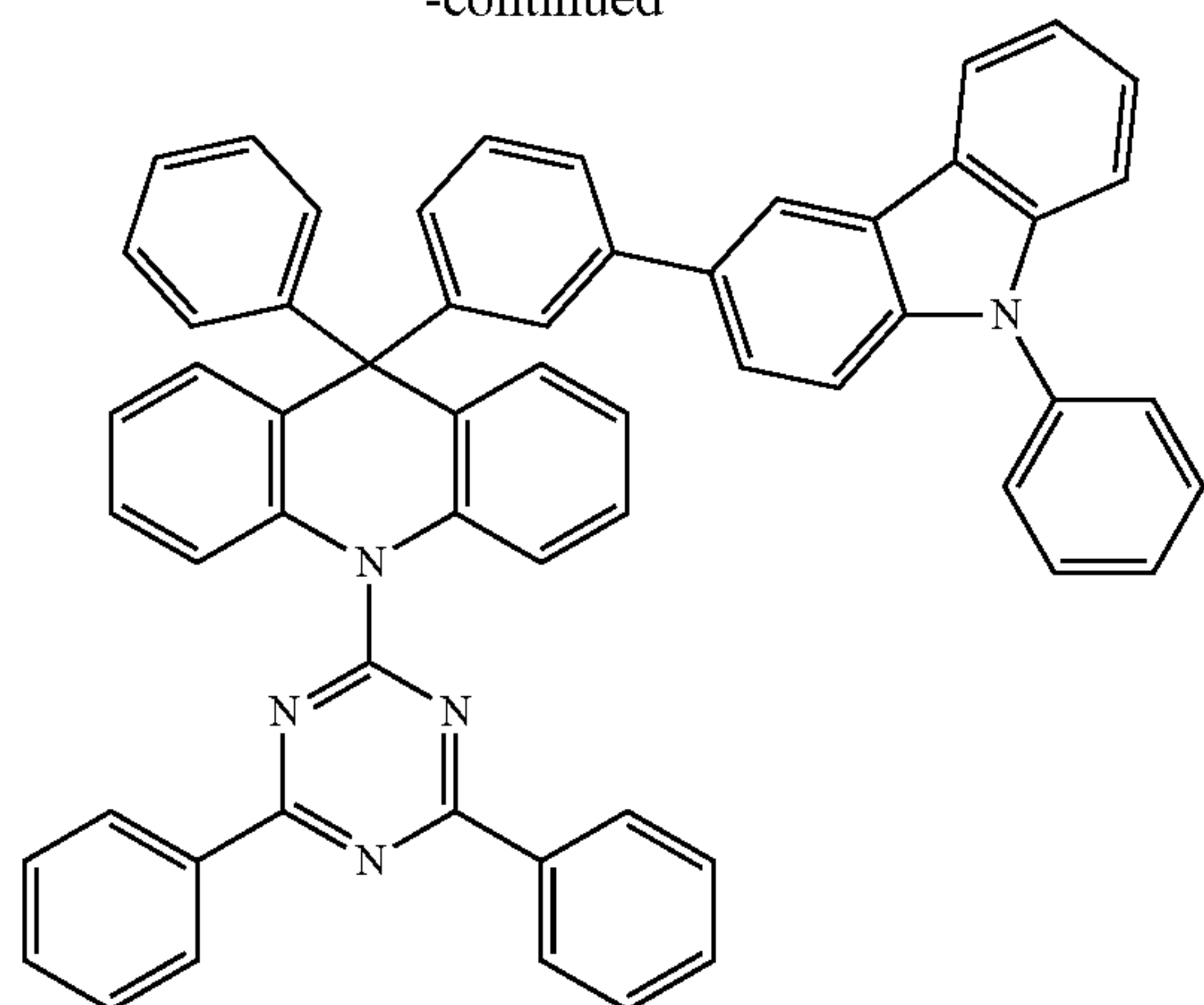
(A-22)
