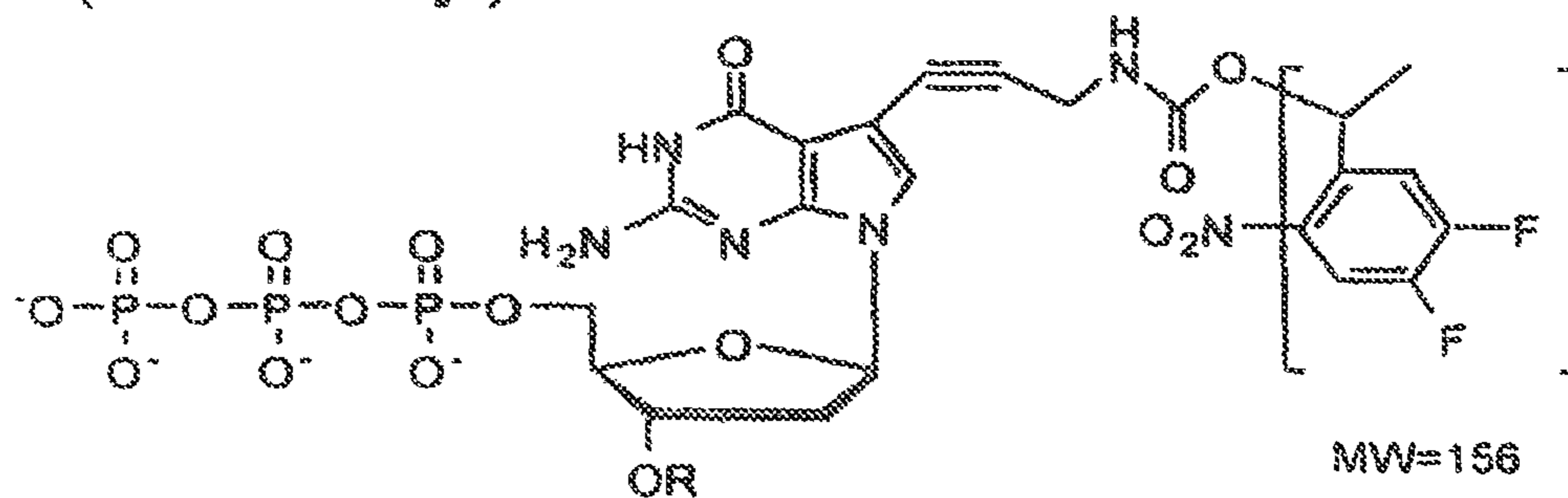
F-(Nitro-Benzyl)-dCTP
