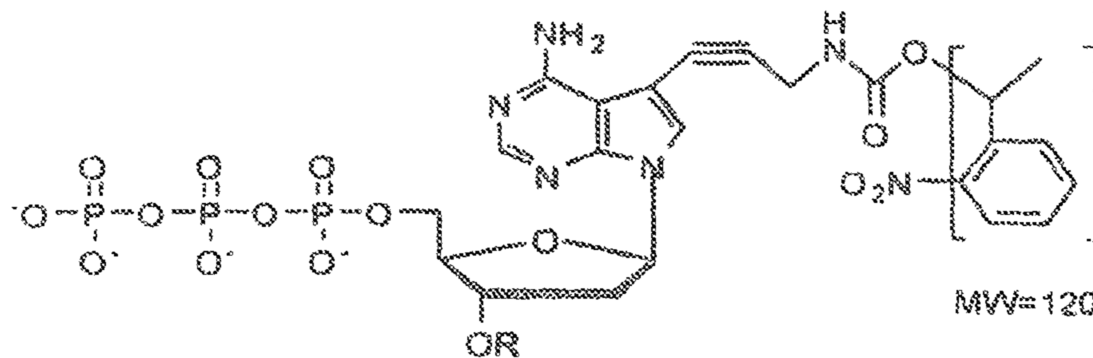
(Nitro-Benzyl)-dATP
