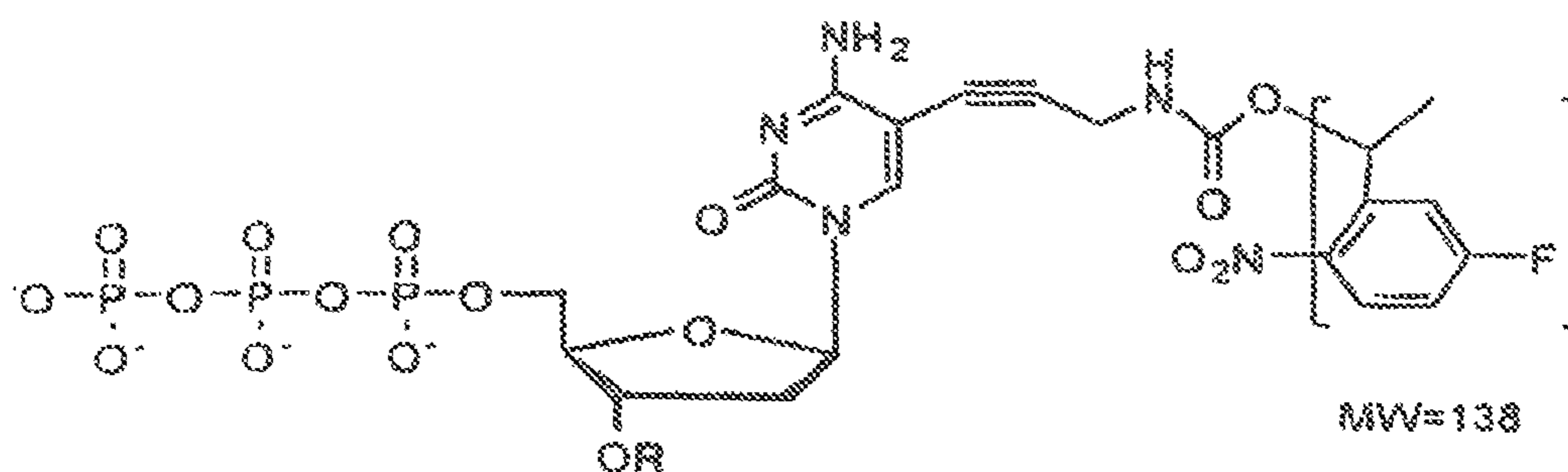
(Nitro-Benzyl)-dATP
