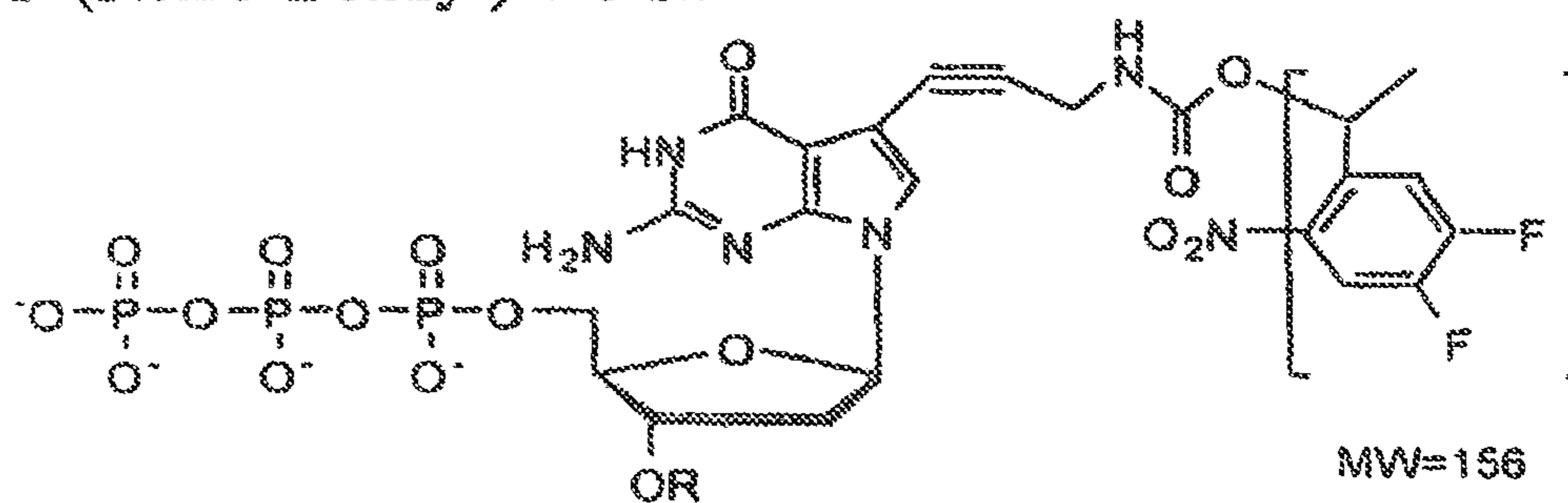
2F-(Nitro-Benzyl)-dGTP
