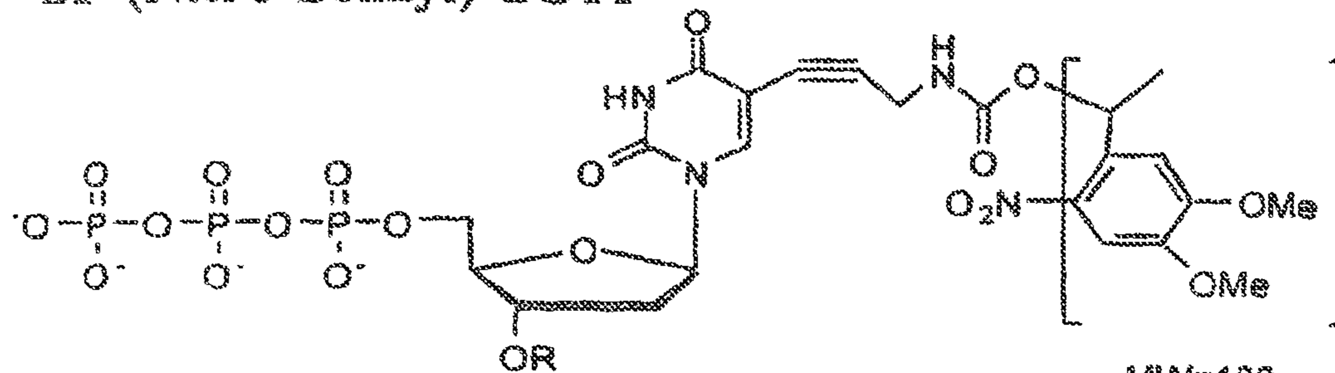
2(Meo)-(Nitro-Benzyl)-dTTP
