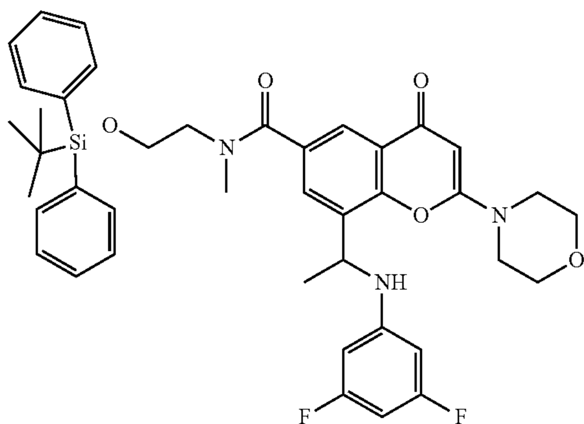
enantiomer 1
