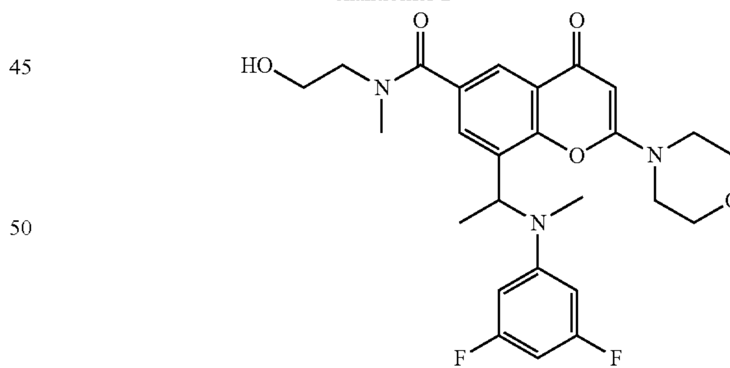
enantiomer 2
