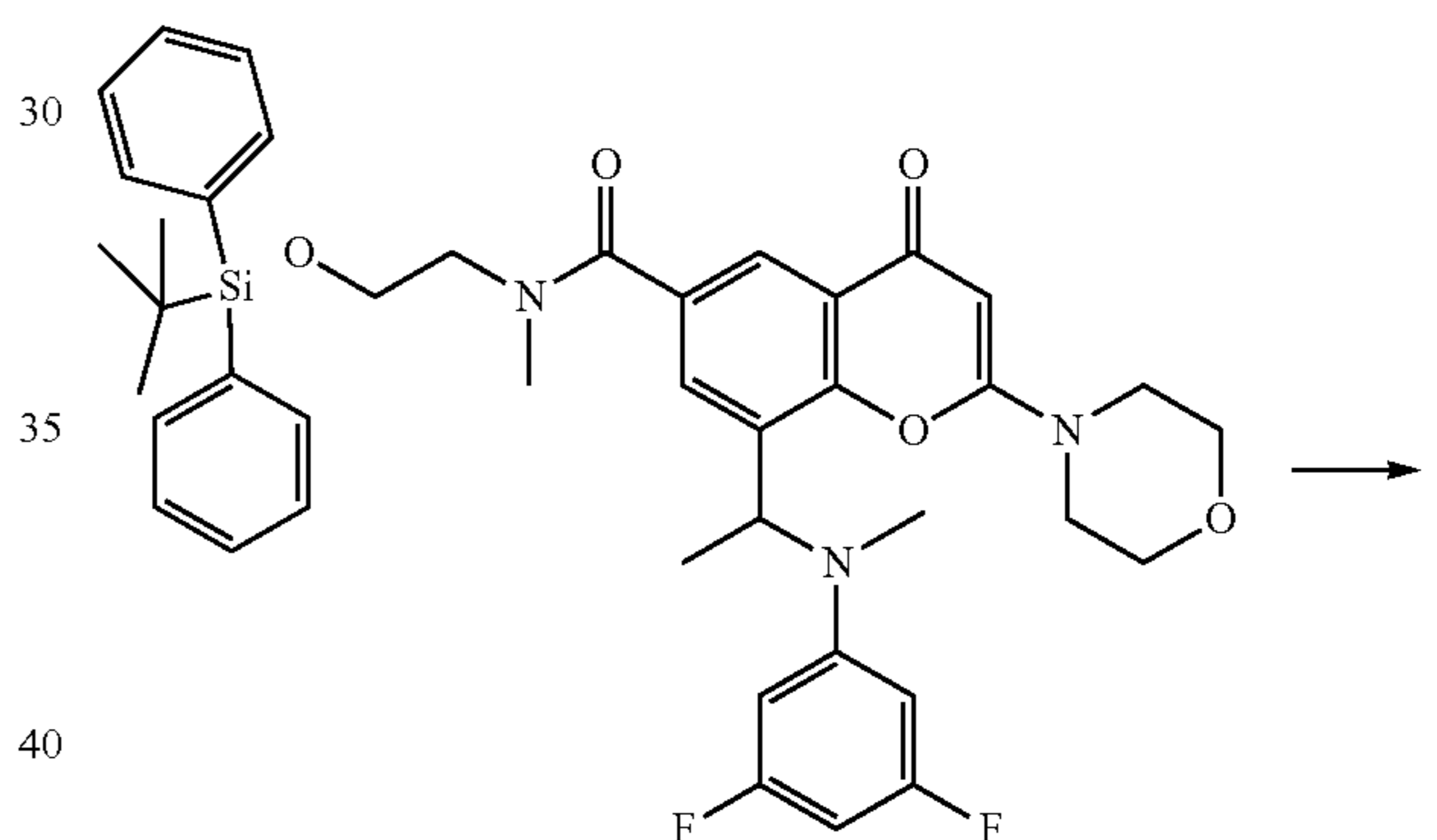
enantiomer 2
