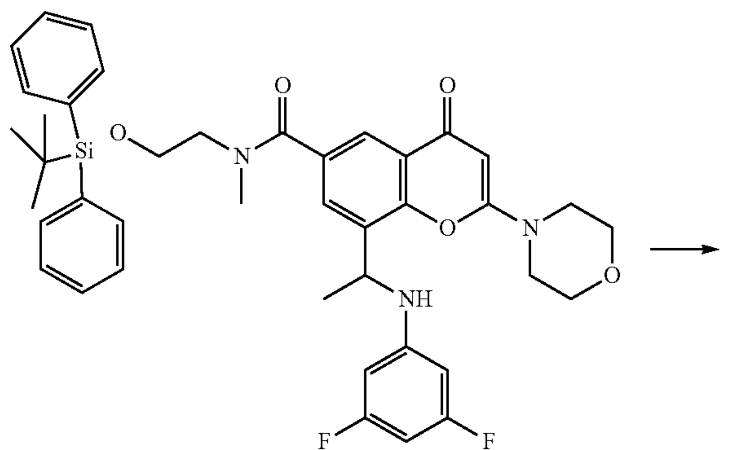
enantiomer 1
