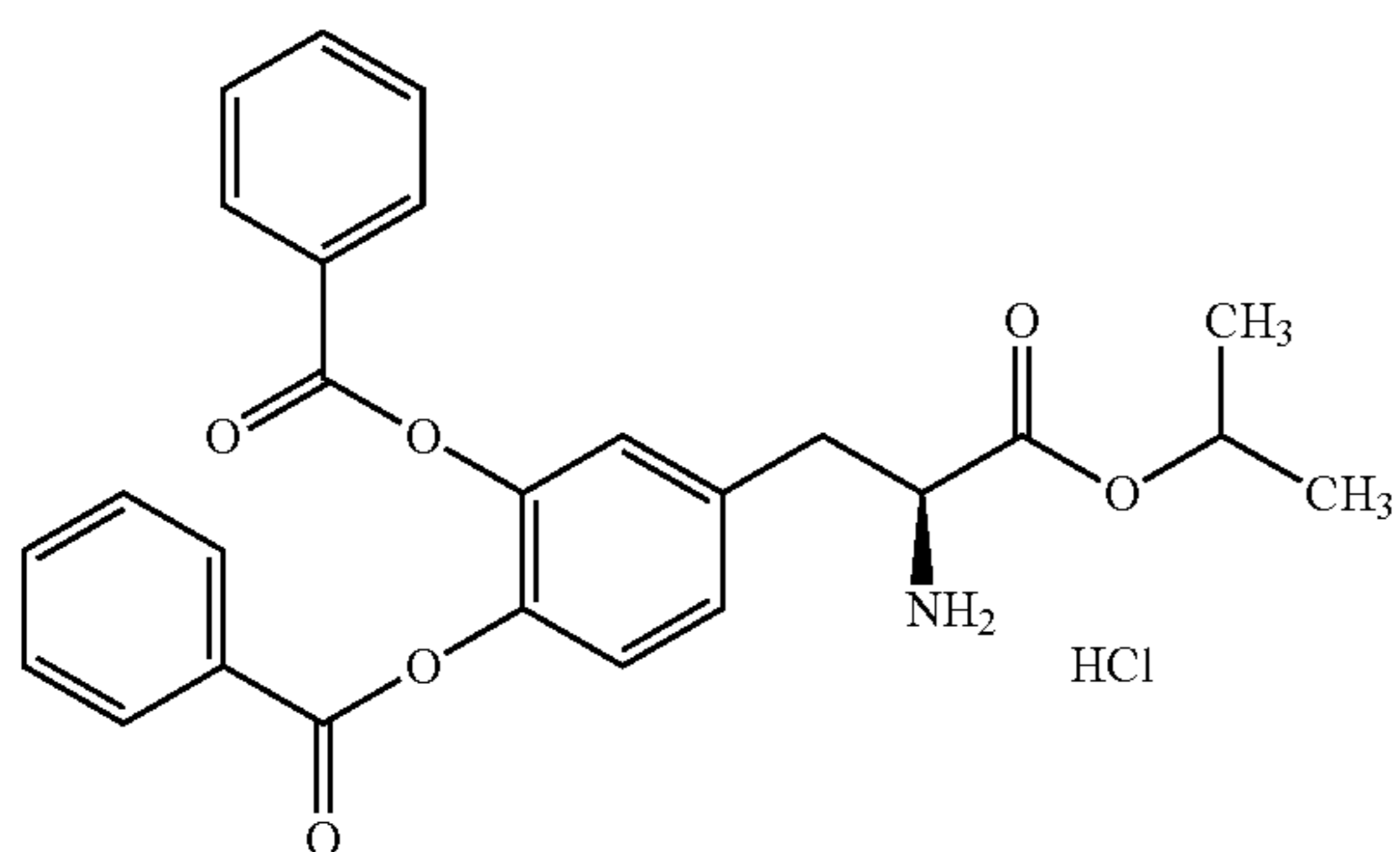
(S)-4-(2-amino-3-isopropoxy-3-oxopropyl)-1,2-phenylene dibenzoate hydrochloride
