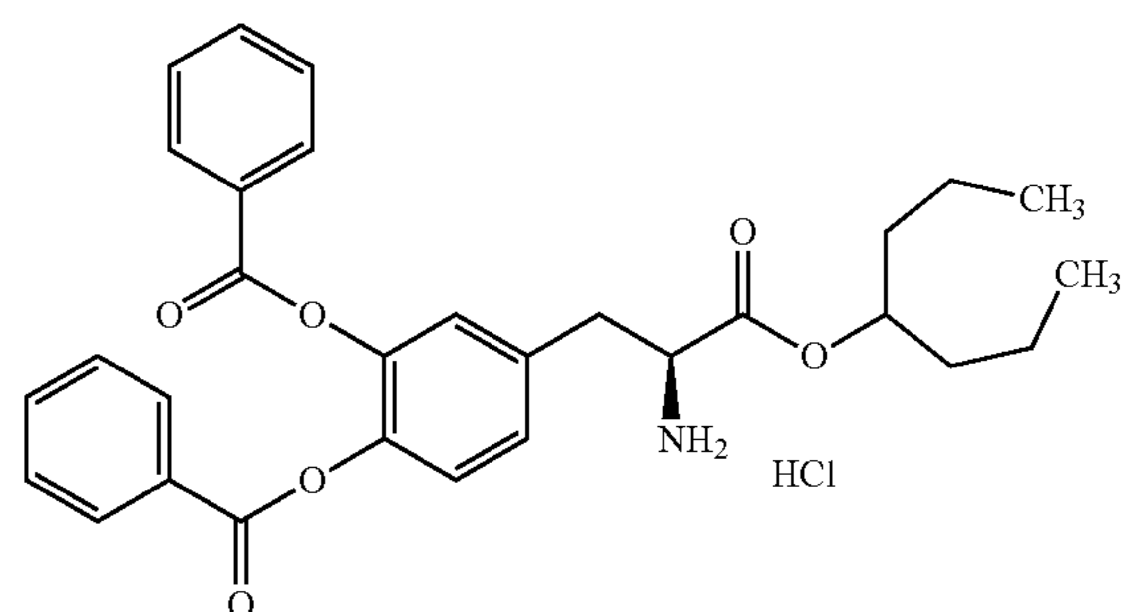
(S)-4-(2-amino-3-(heptan-4-yloxy)-3-oxopropyl)-1,2-phenylene dibenzoate
