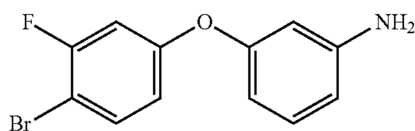
3-(4-bromo-3-fluorophenoxy)benzenamine
