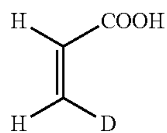
(Z)-3-deuteriumacrylic acid
