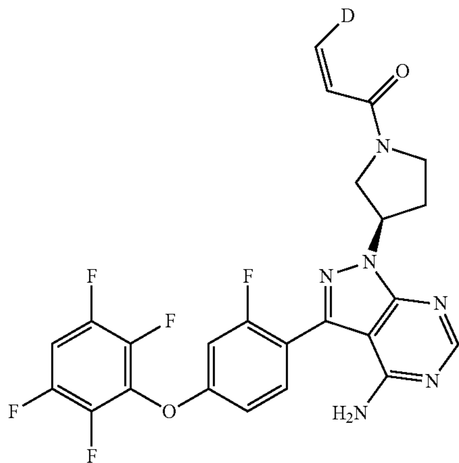
(Z)-1-((R)-3-(4-amino-3-(2-fluoro-4-(3-fluorophenoxy)phenyl)-1H-pyrazolo[3,4-d]pyrimidin-1-yl)pyrrolidin-1-yl)-3-deuterium-prop-2-en-1-one
