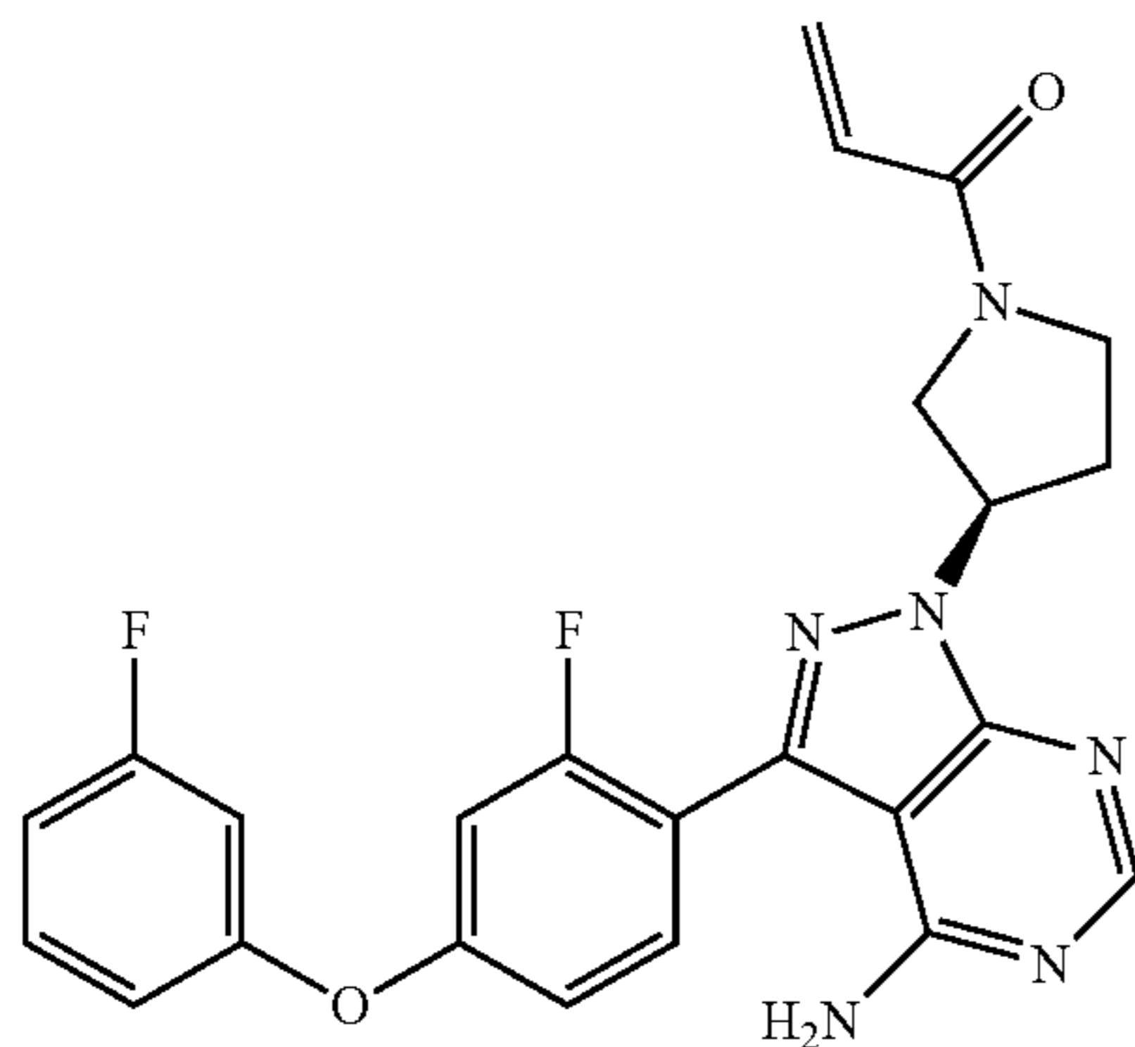
1-((R)-3-(4-amino-3-(2-fluoro-4-(3-fluorophenoxy)phenyl)-1H-pyrazolo[3,4-d]pyrimidin-1-yl)pyrrolidin-1-yl)prop-2-en-1-one
