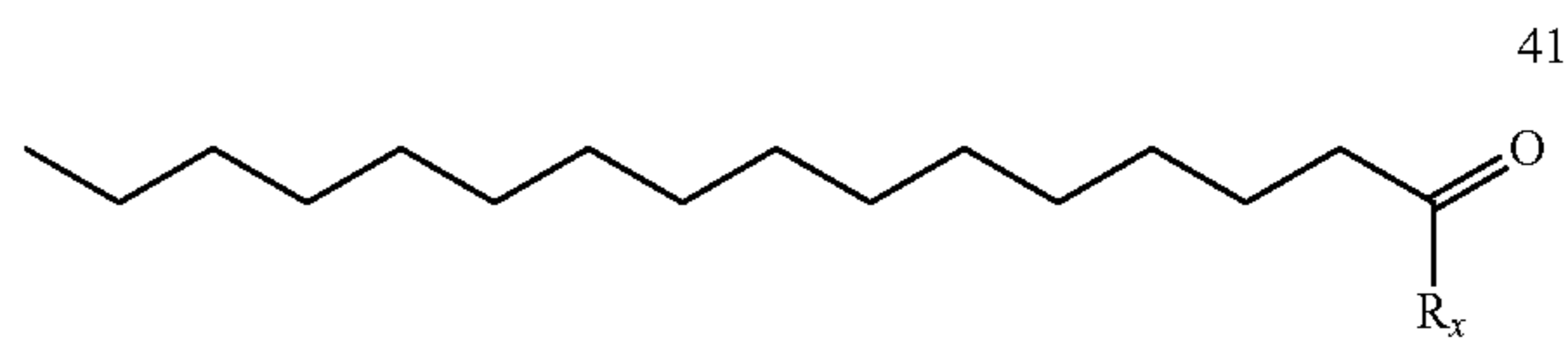
(16:Ald)
