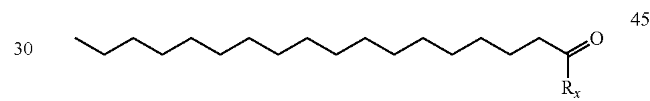
(18:Ald)
