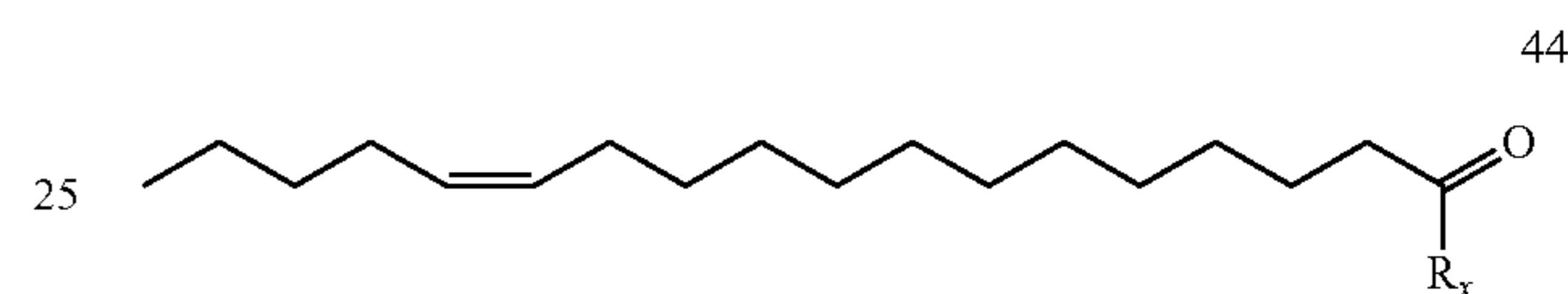
(Z13-18:Ald)
