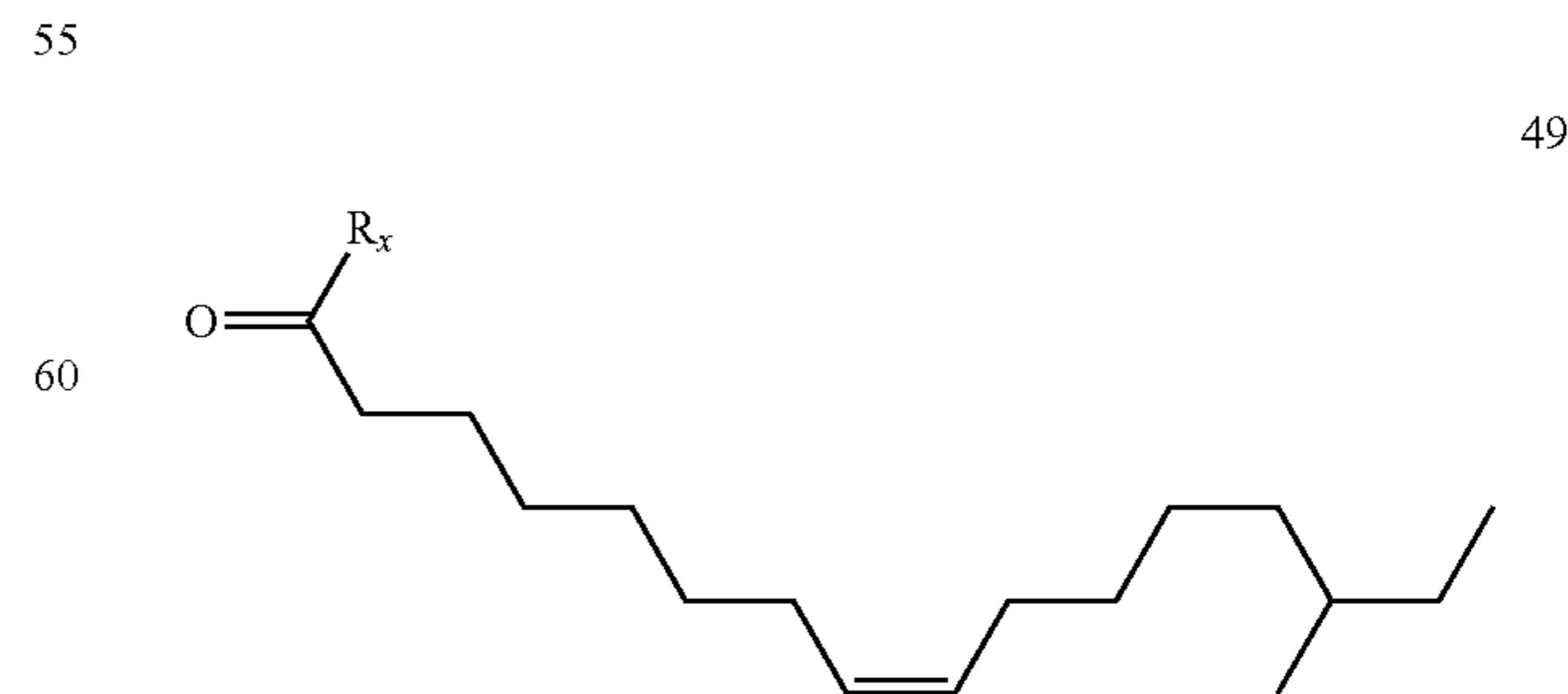
(14Me-Z8-16:Ald, Z-trogoderma)
