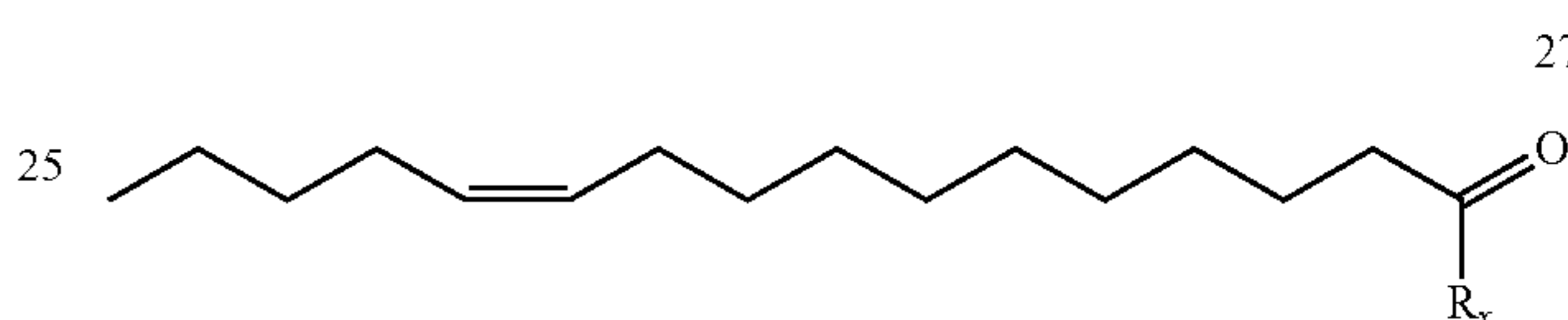
(Z11-16:Ald)
