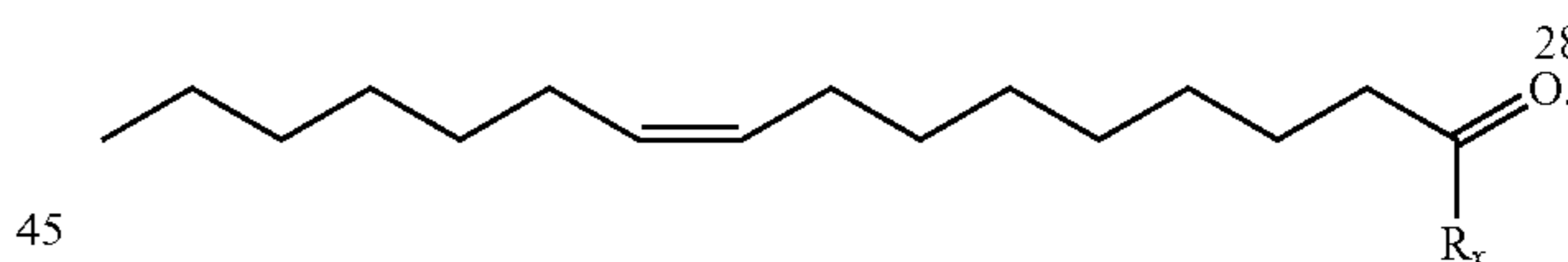
(Z9-16:Ald)
