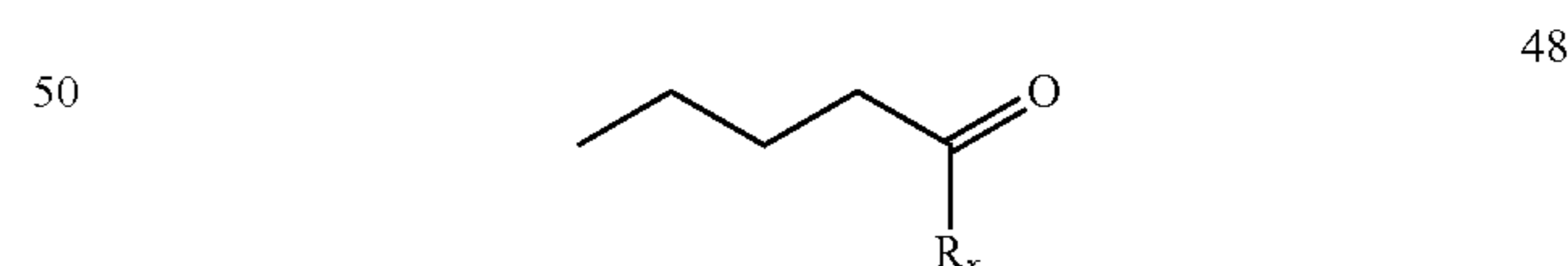
(5:Ald)
