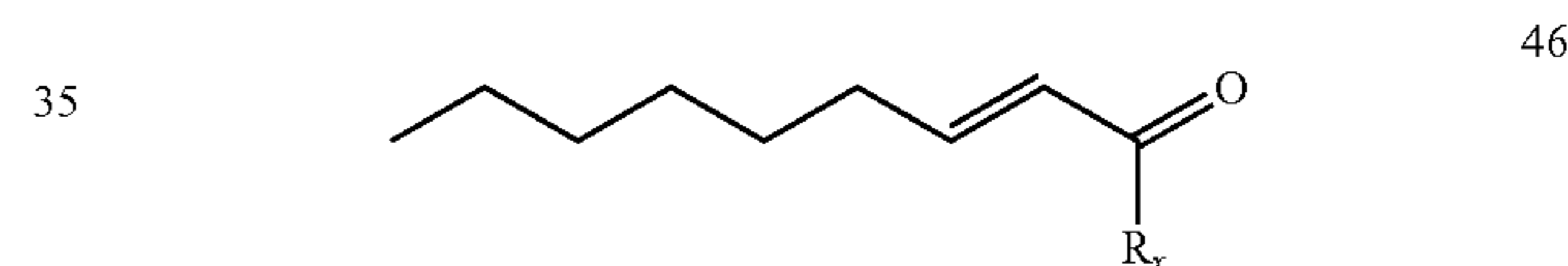
(E2-9:Ald)
