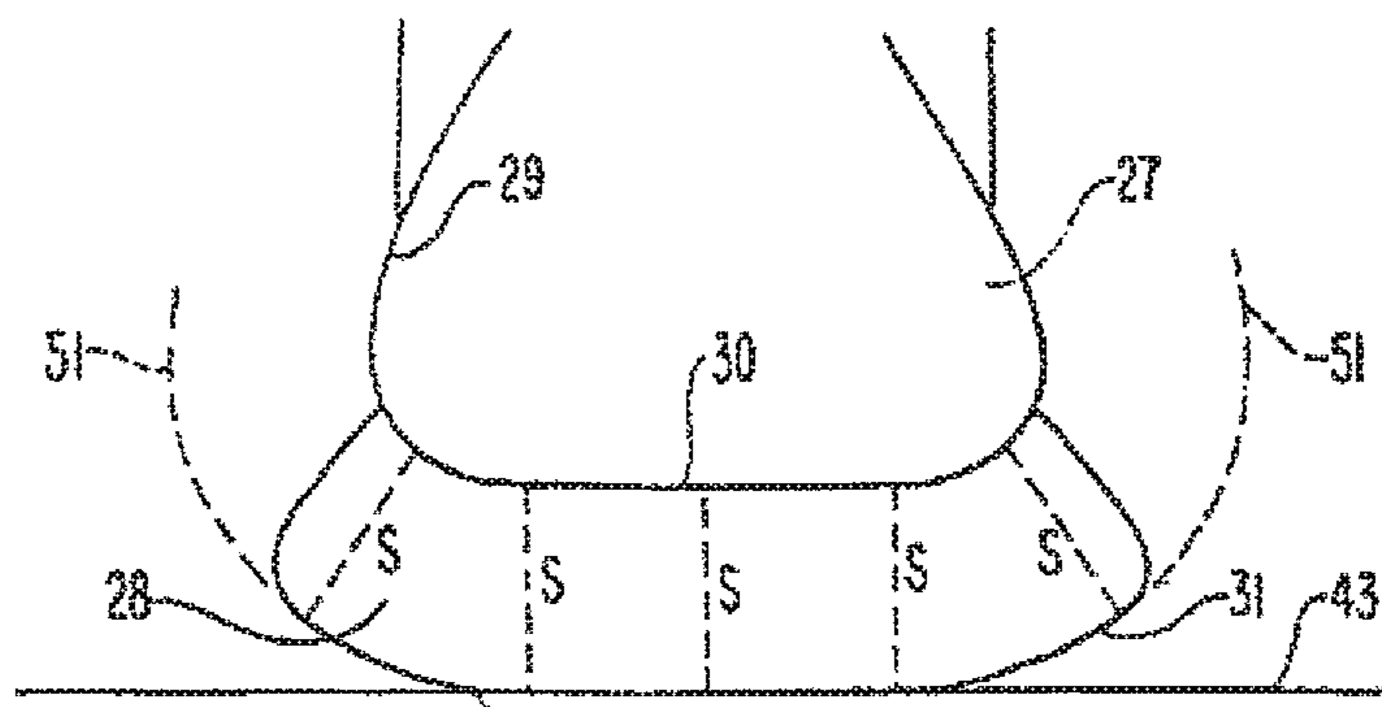
145 FIG. 14C PRIOR ART
