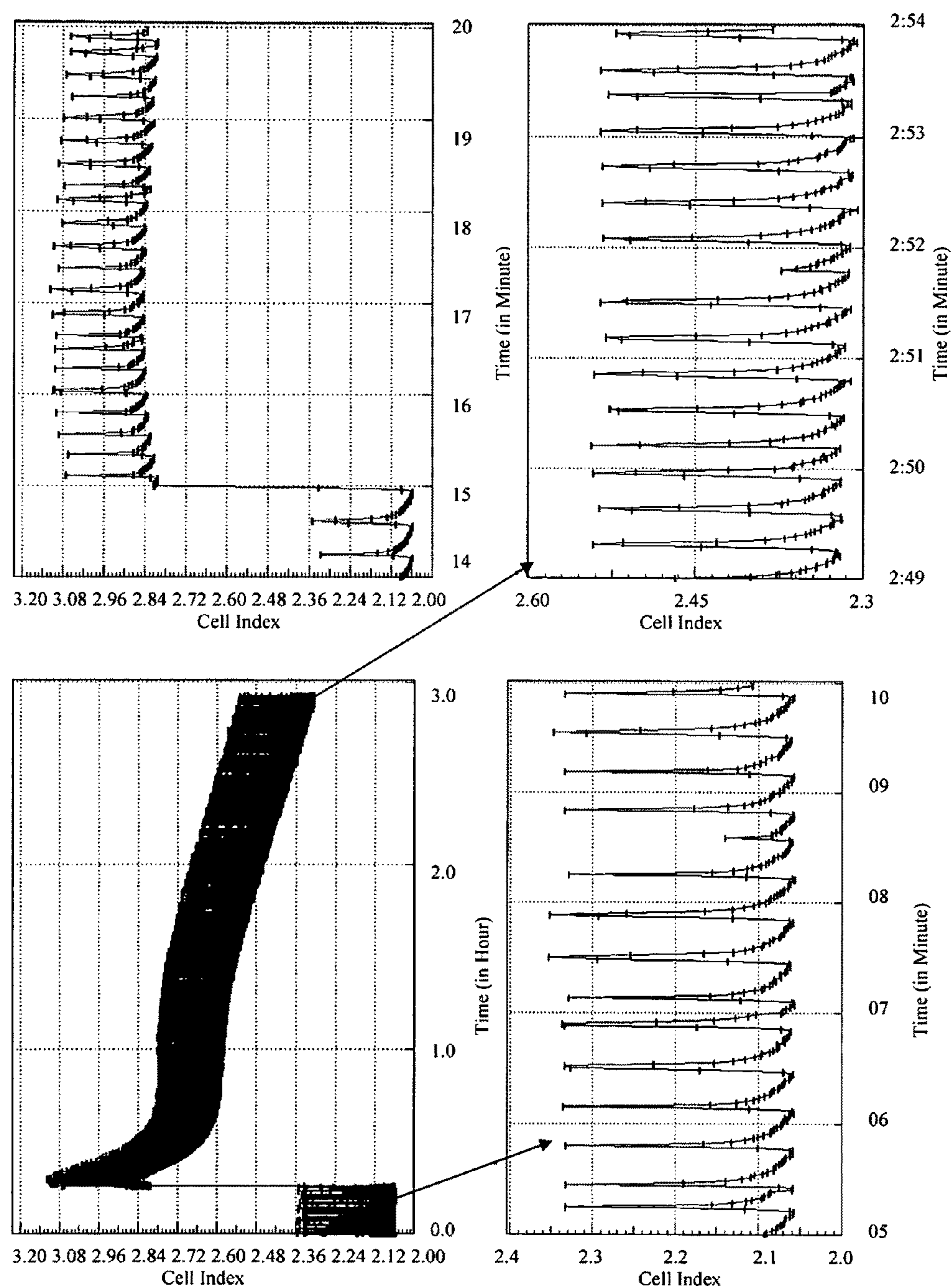
FIG. 11S DMSO 0.13%
