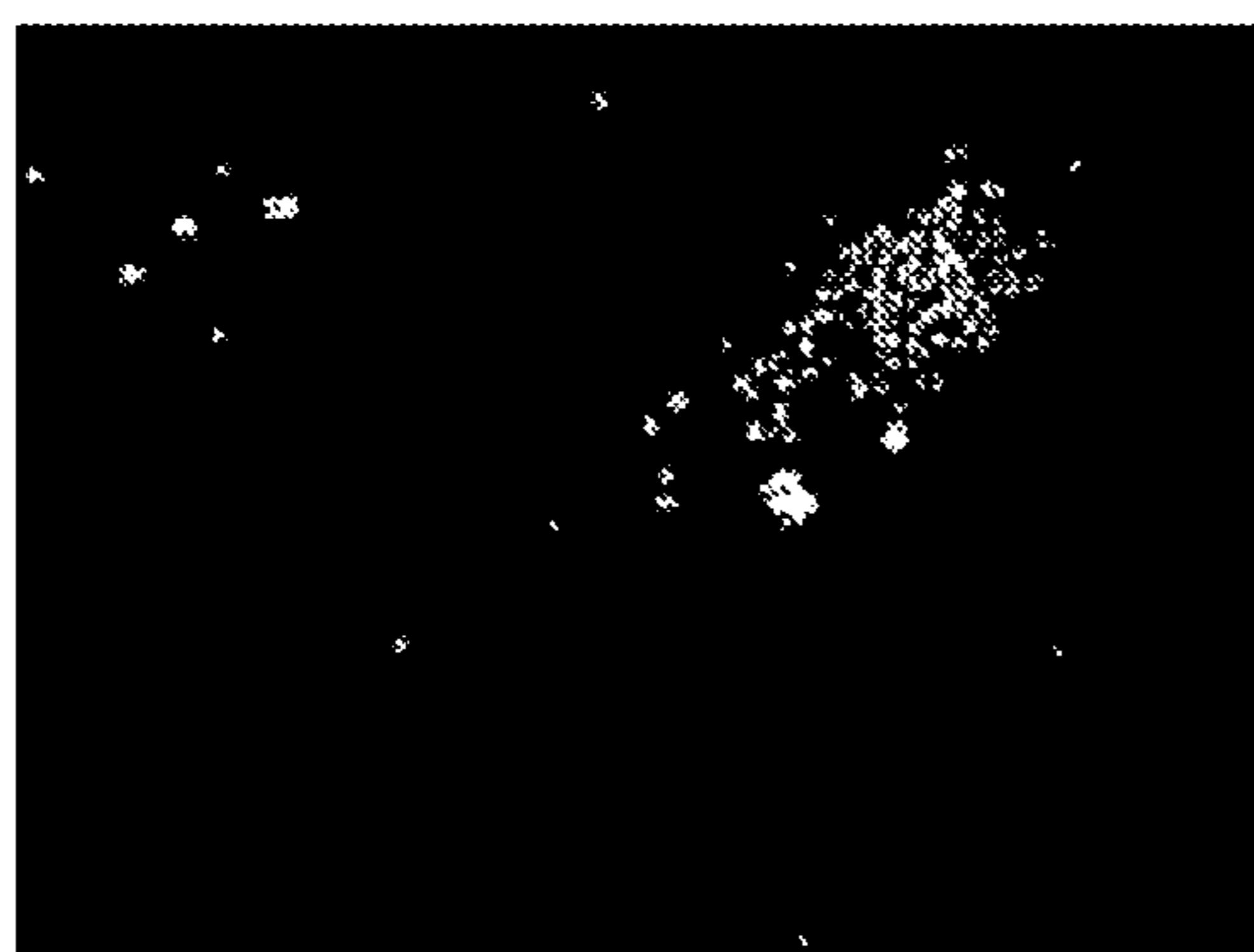
beta-D-amino-LNA; 2752
