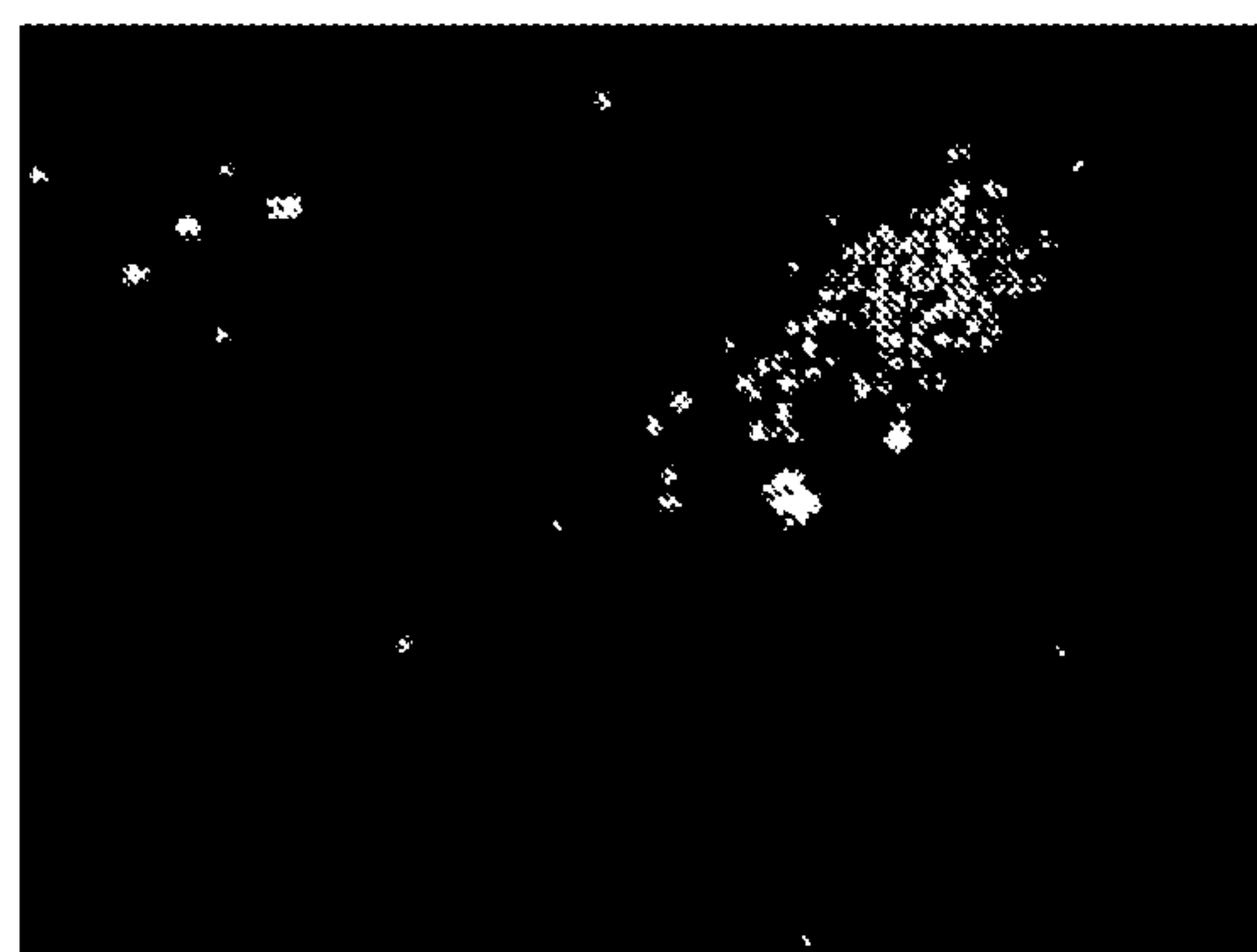
beta-D-amino-LNA; 2752
