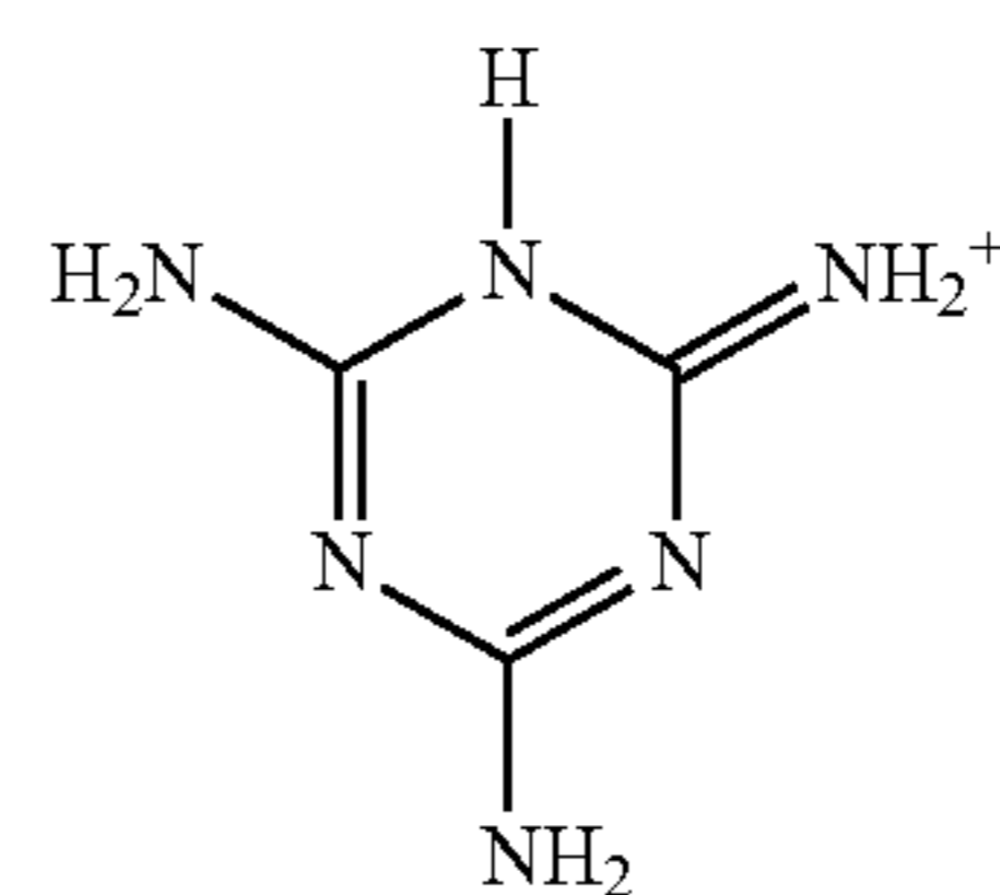
melamine
