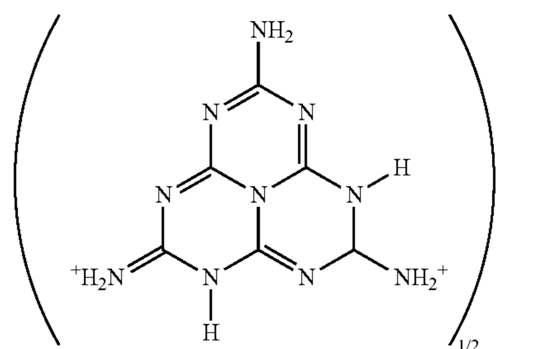
melem
