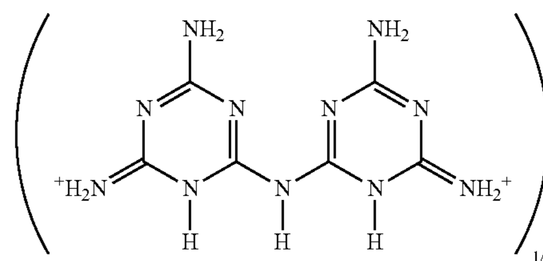
melam
