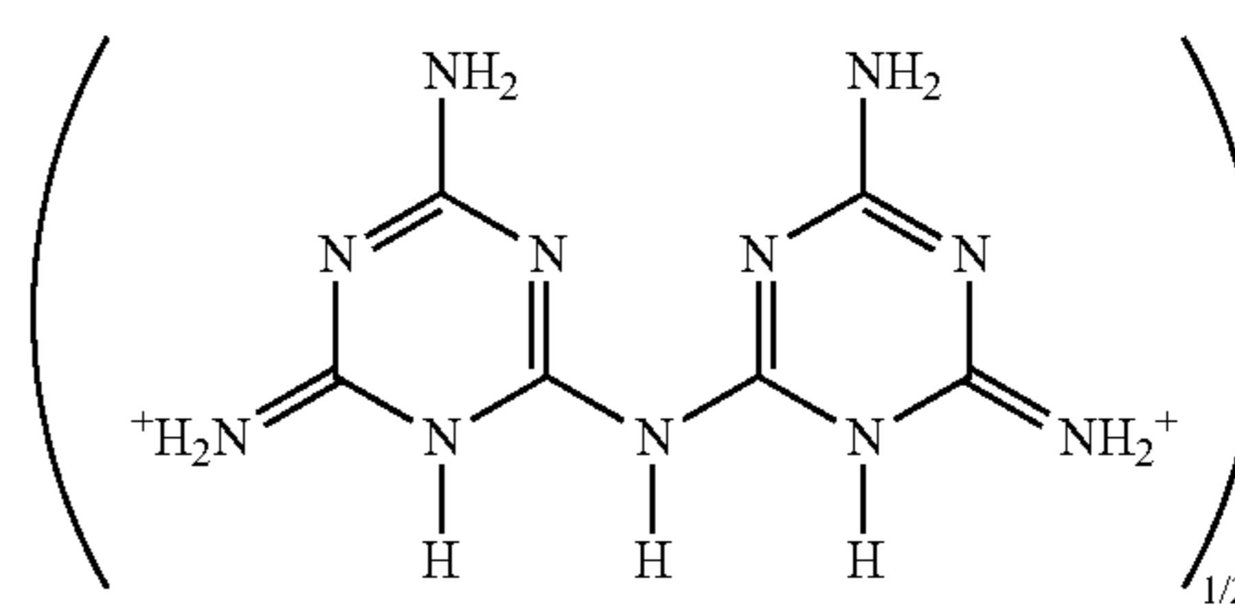
melam
