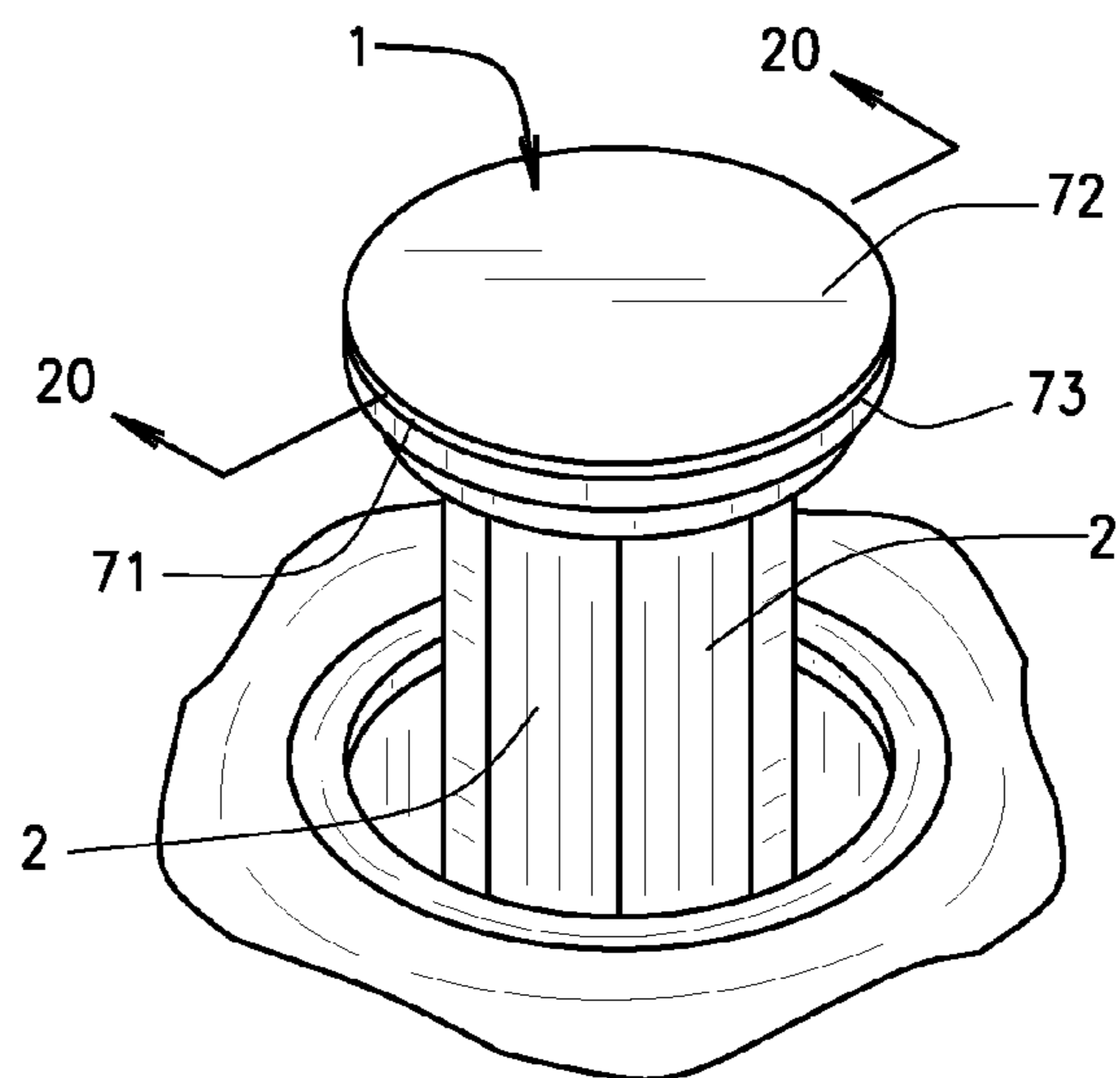
FIG. 19
