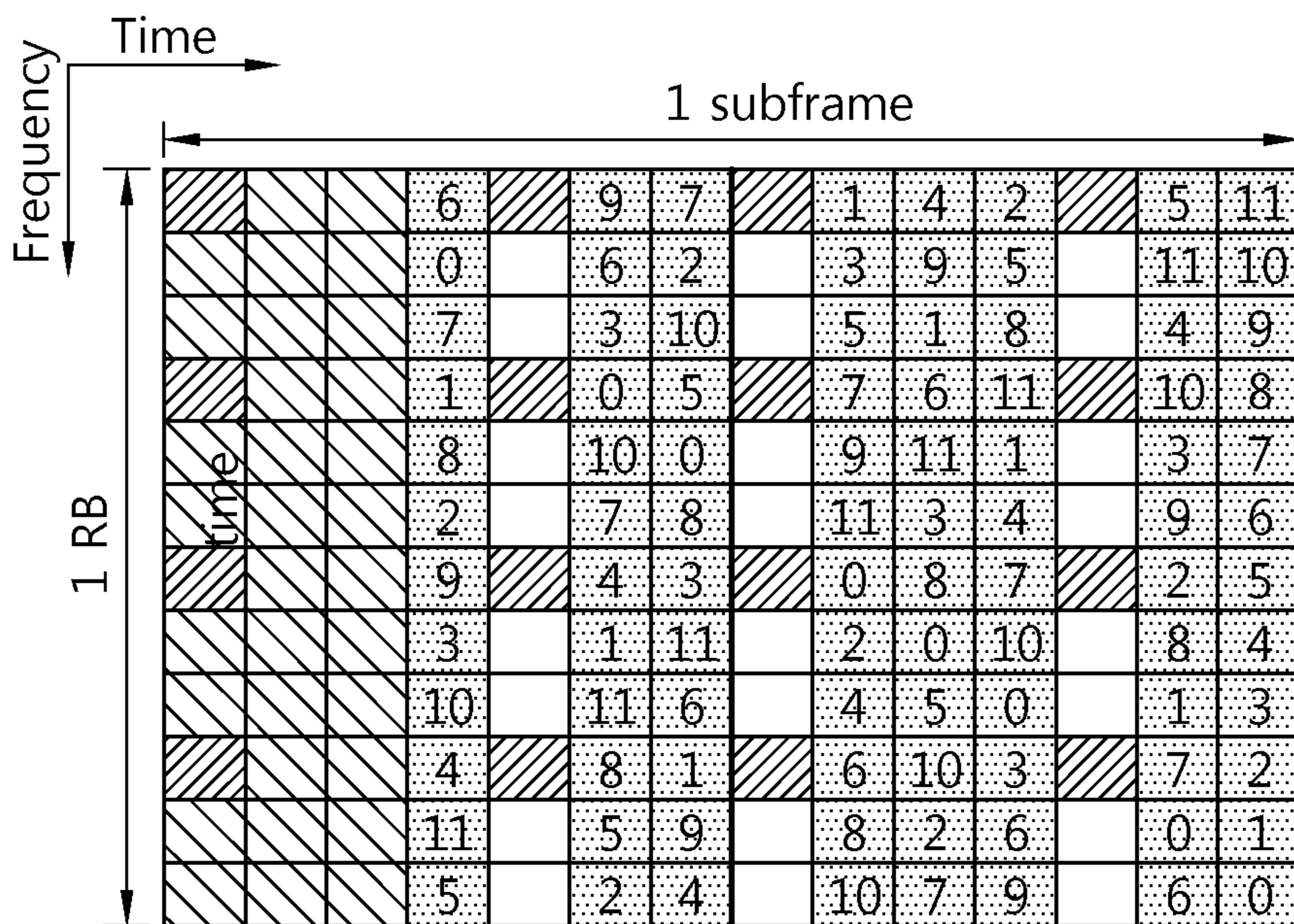
Normal subframe
