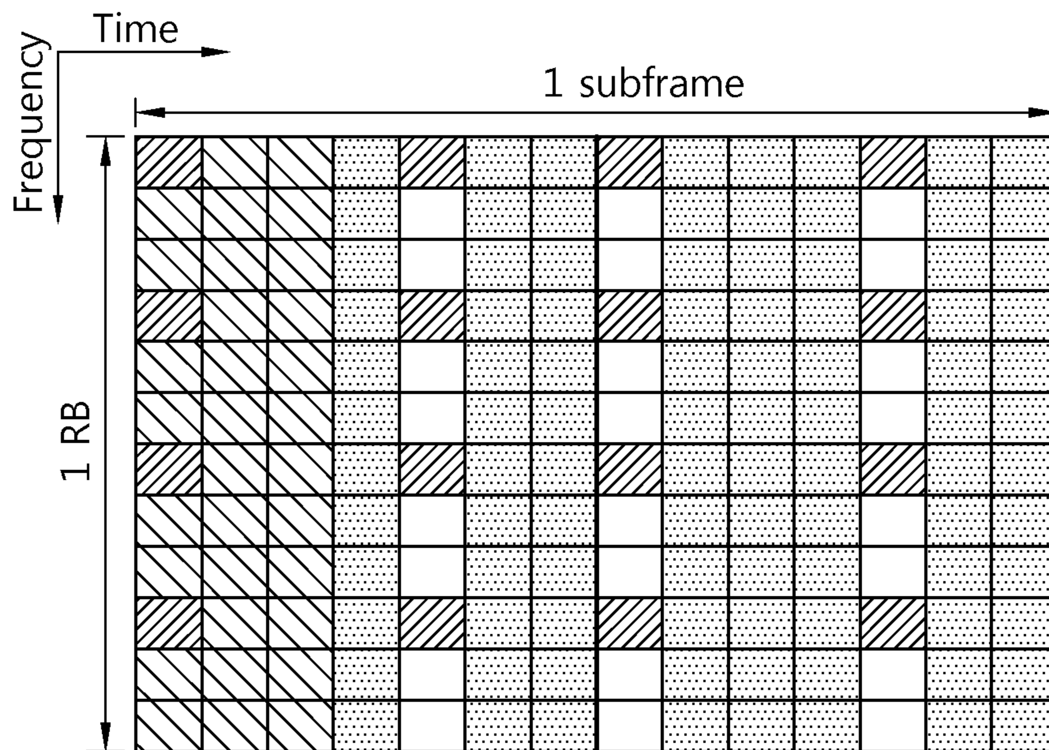
Normal subframe
