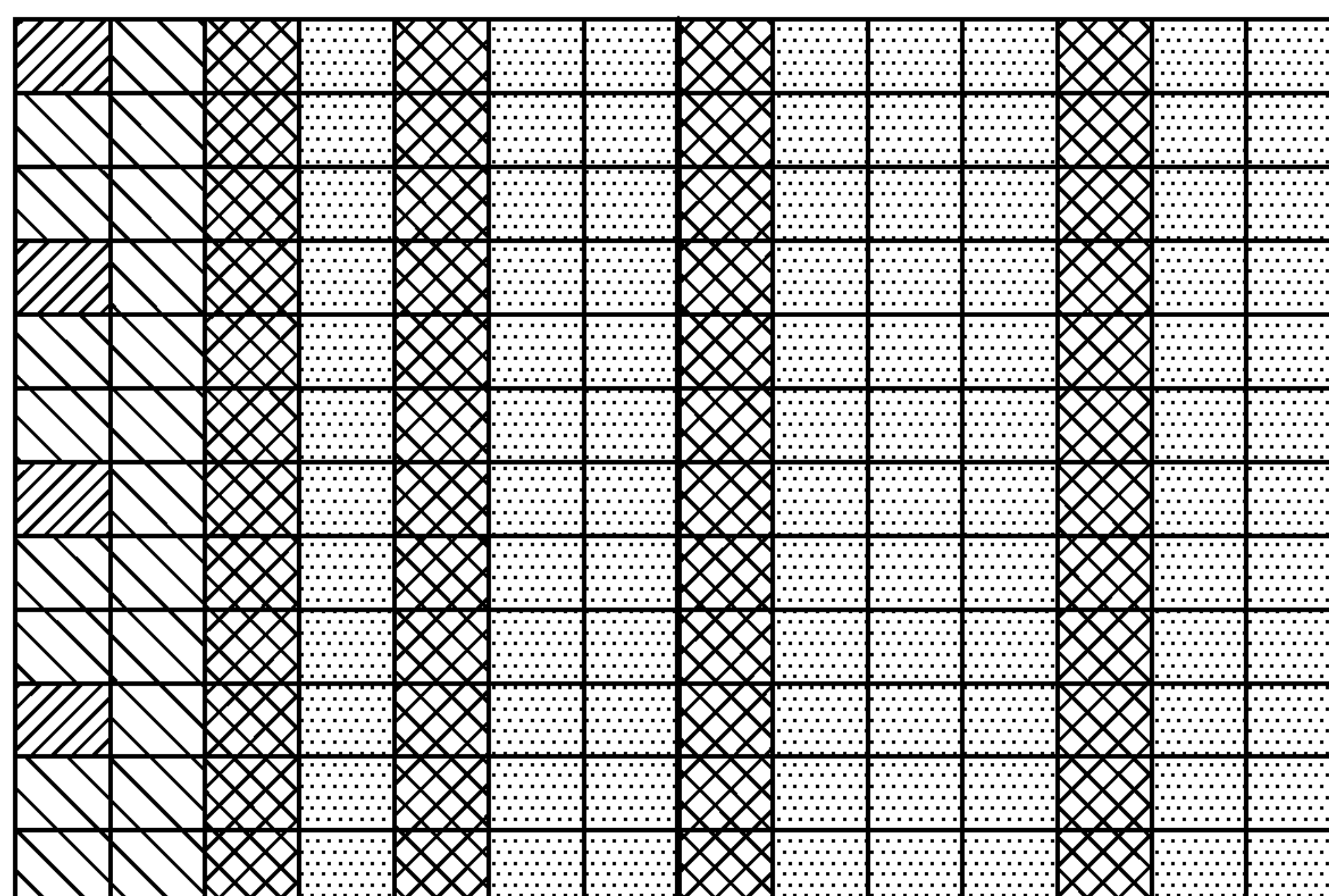
MBSFN subframe
