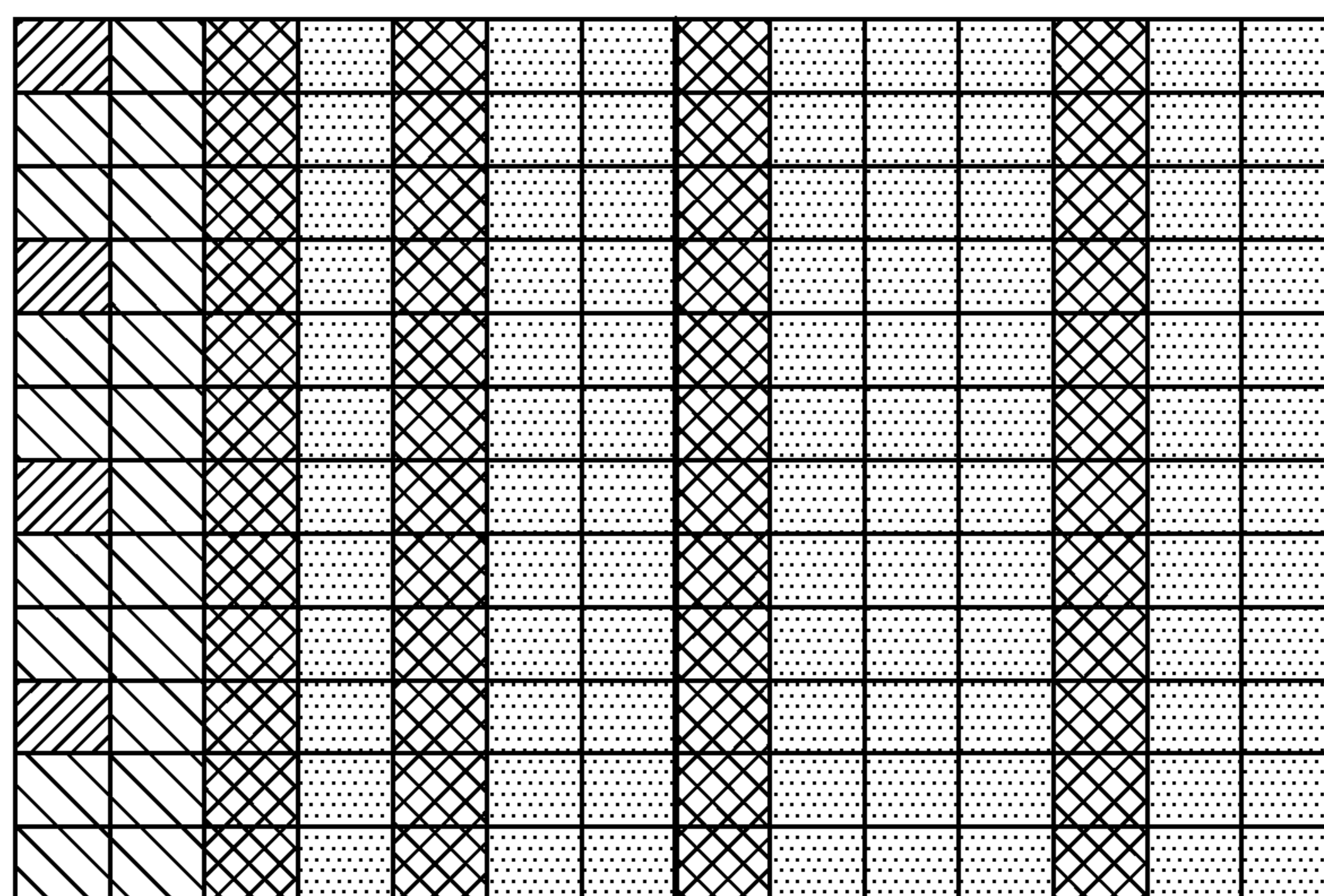
MBSFN subframe
