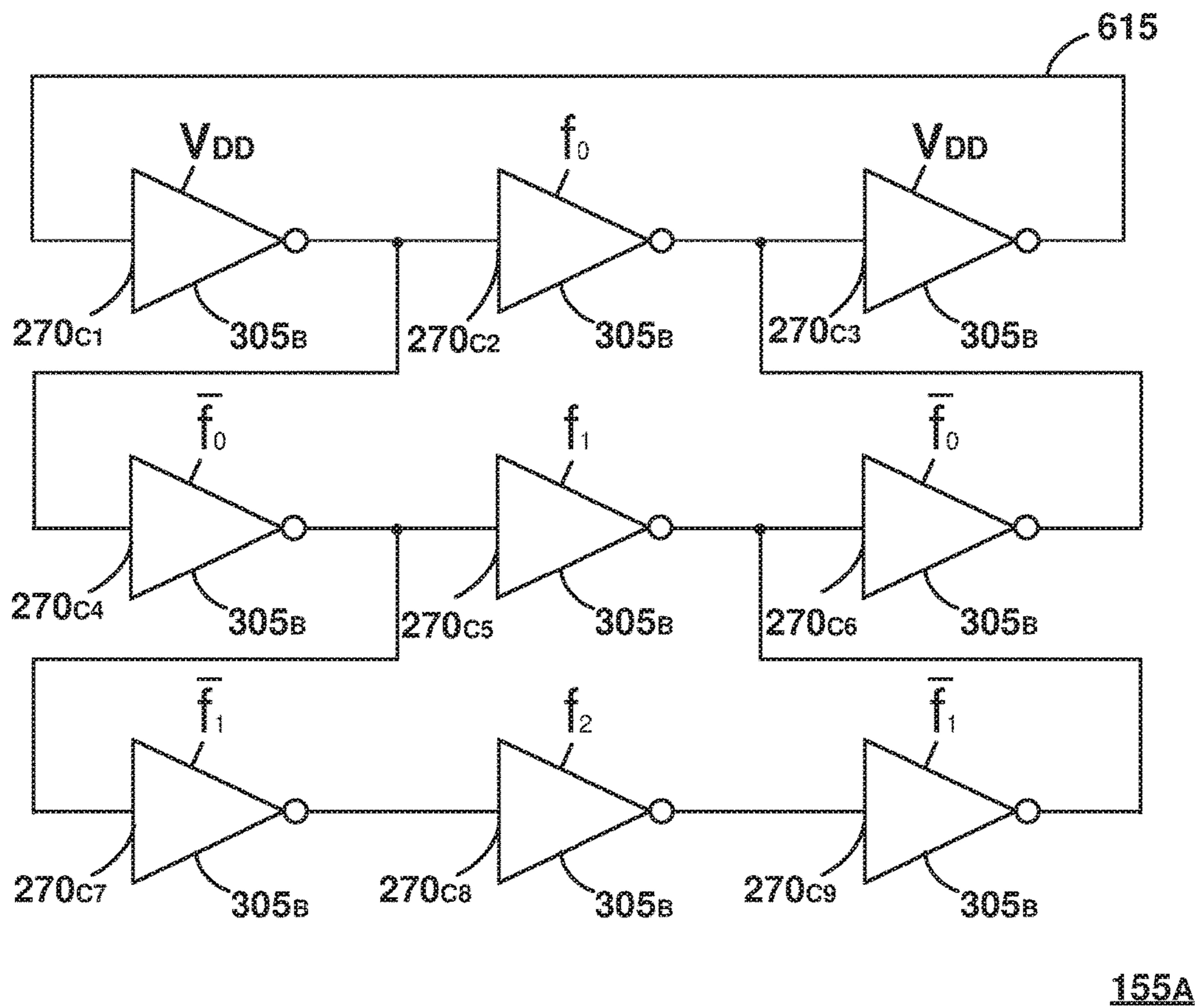
FIG. 31
