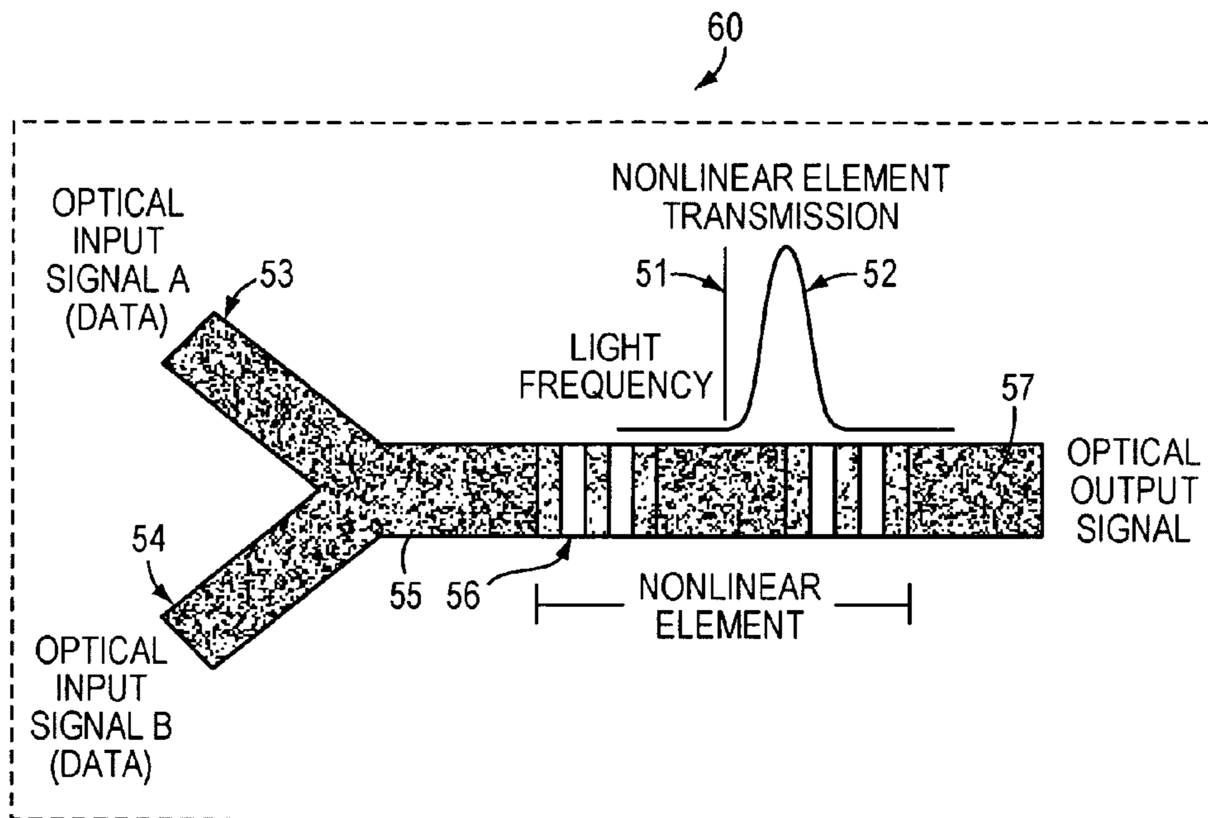
ALL-OPTICAL XOR GATE
