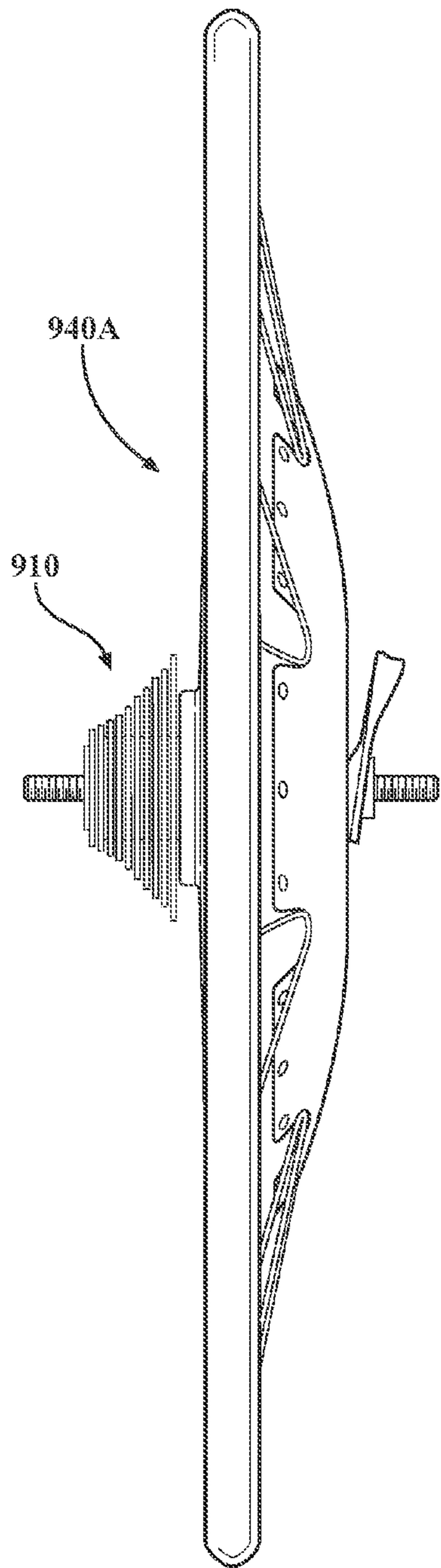
FIG. 10A
