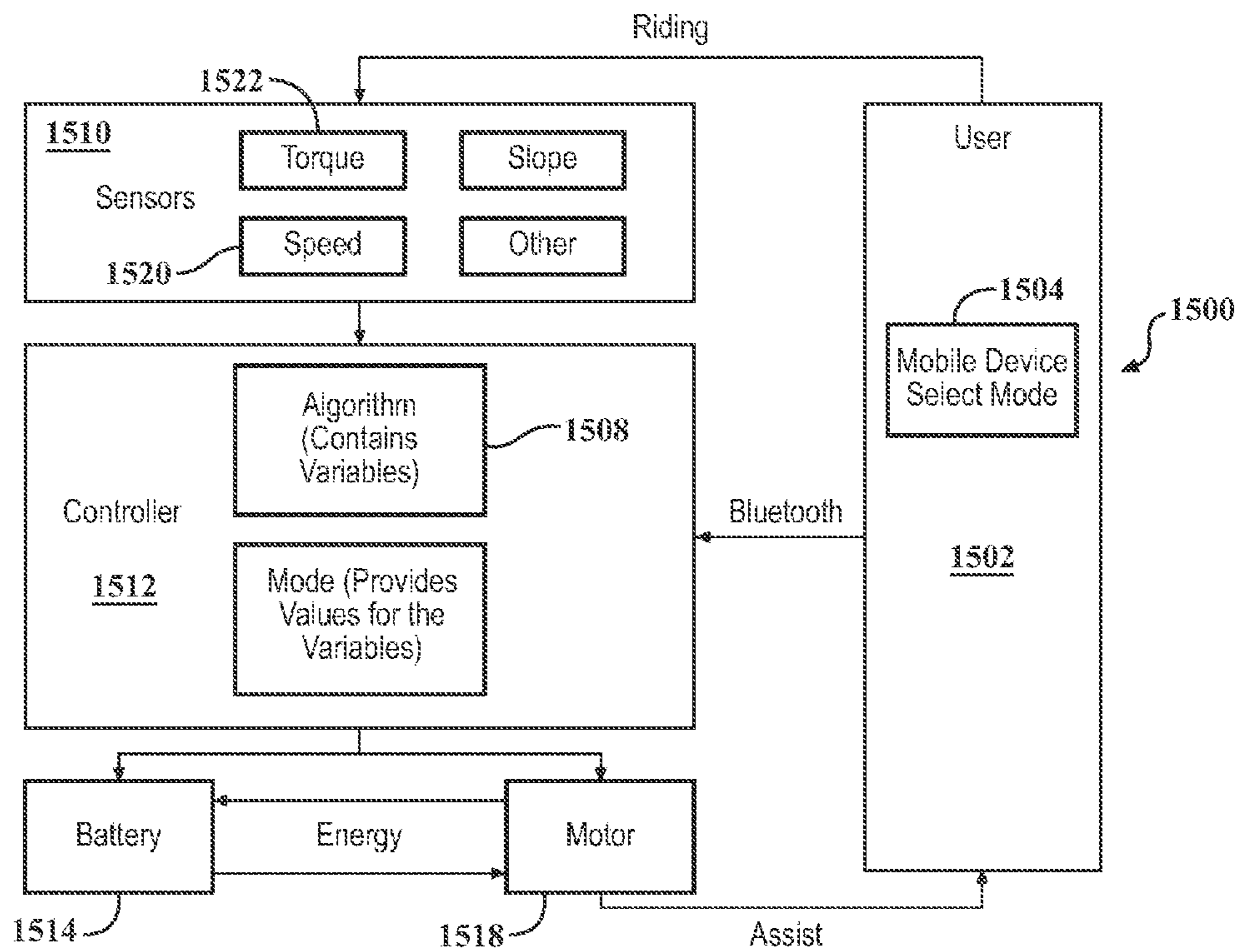
FIG. 15A
