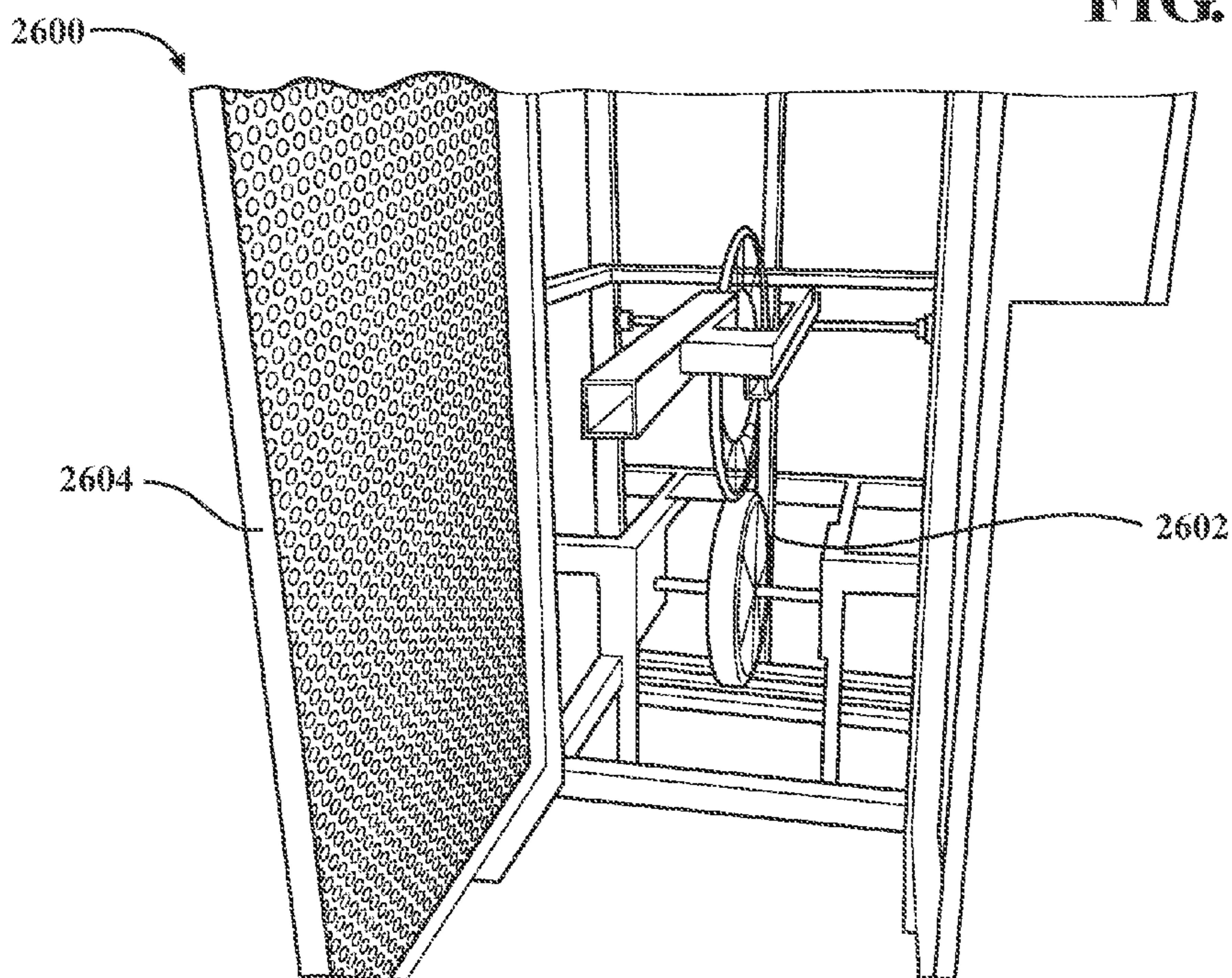
FIG. 26A
