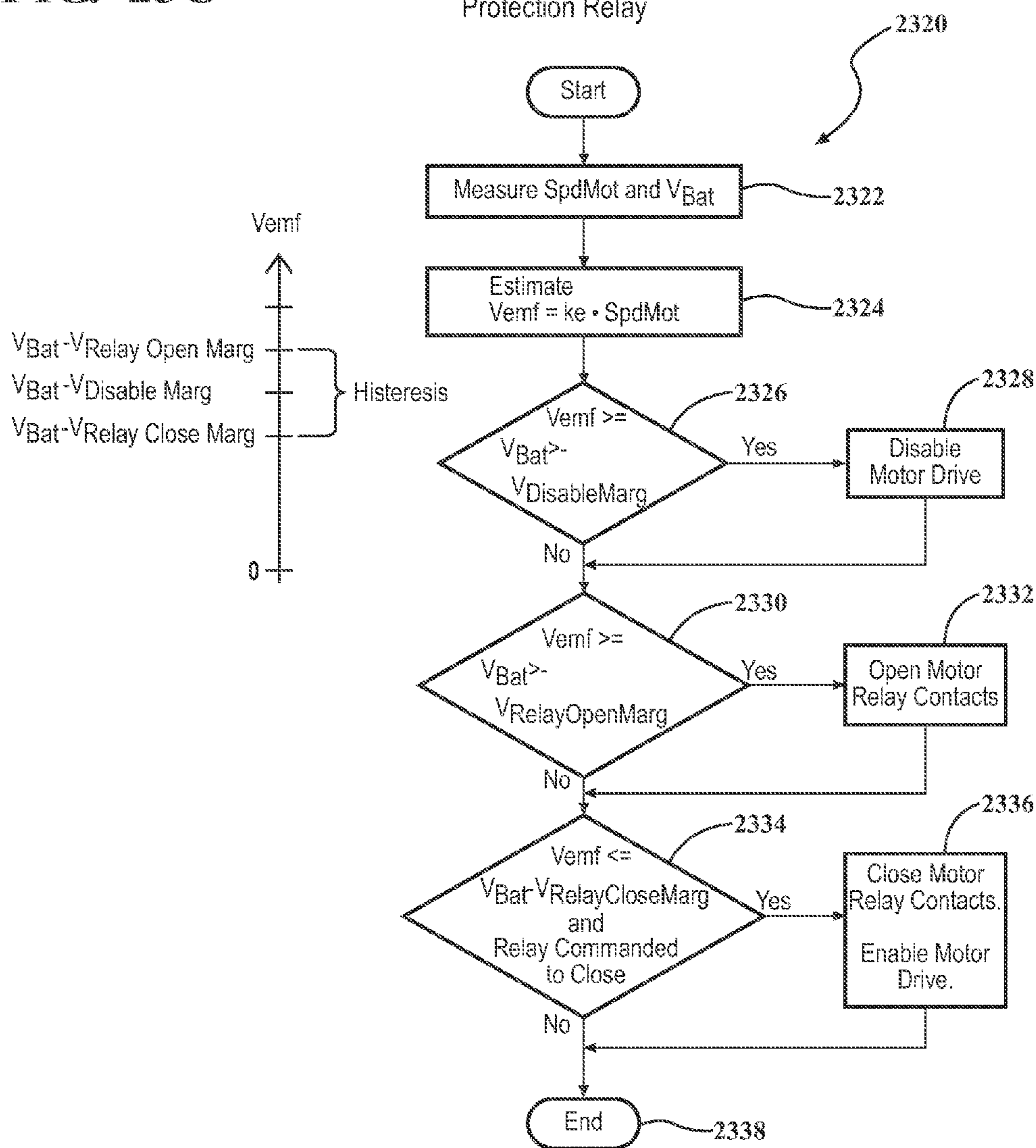
FIG. 23C
