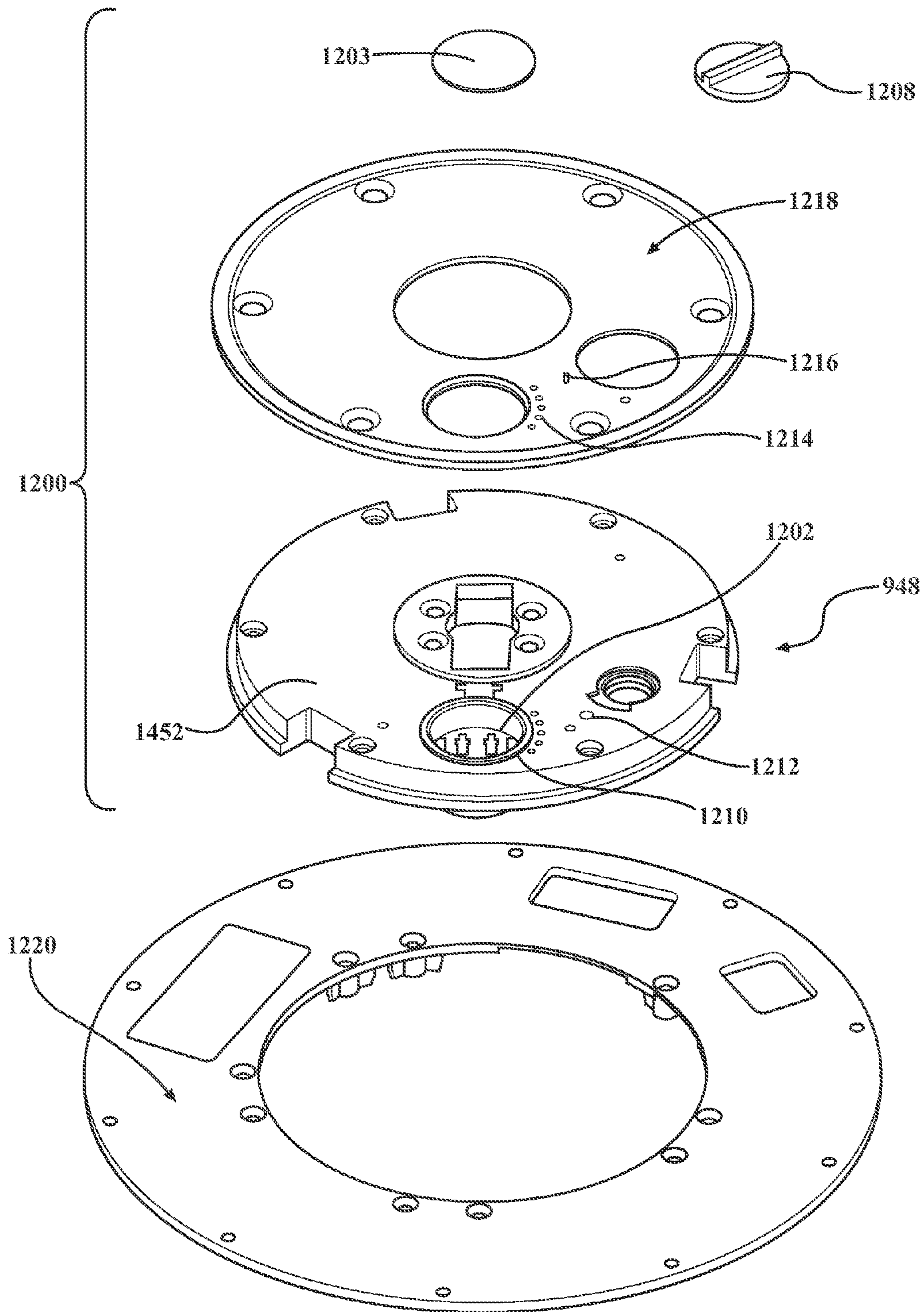
FIG. 12B
