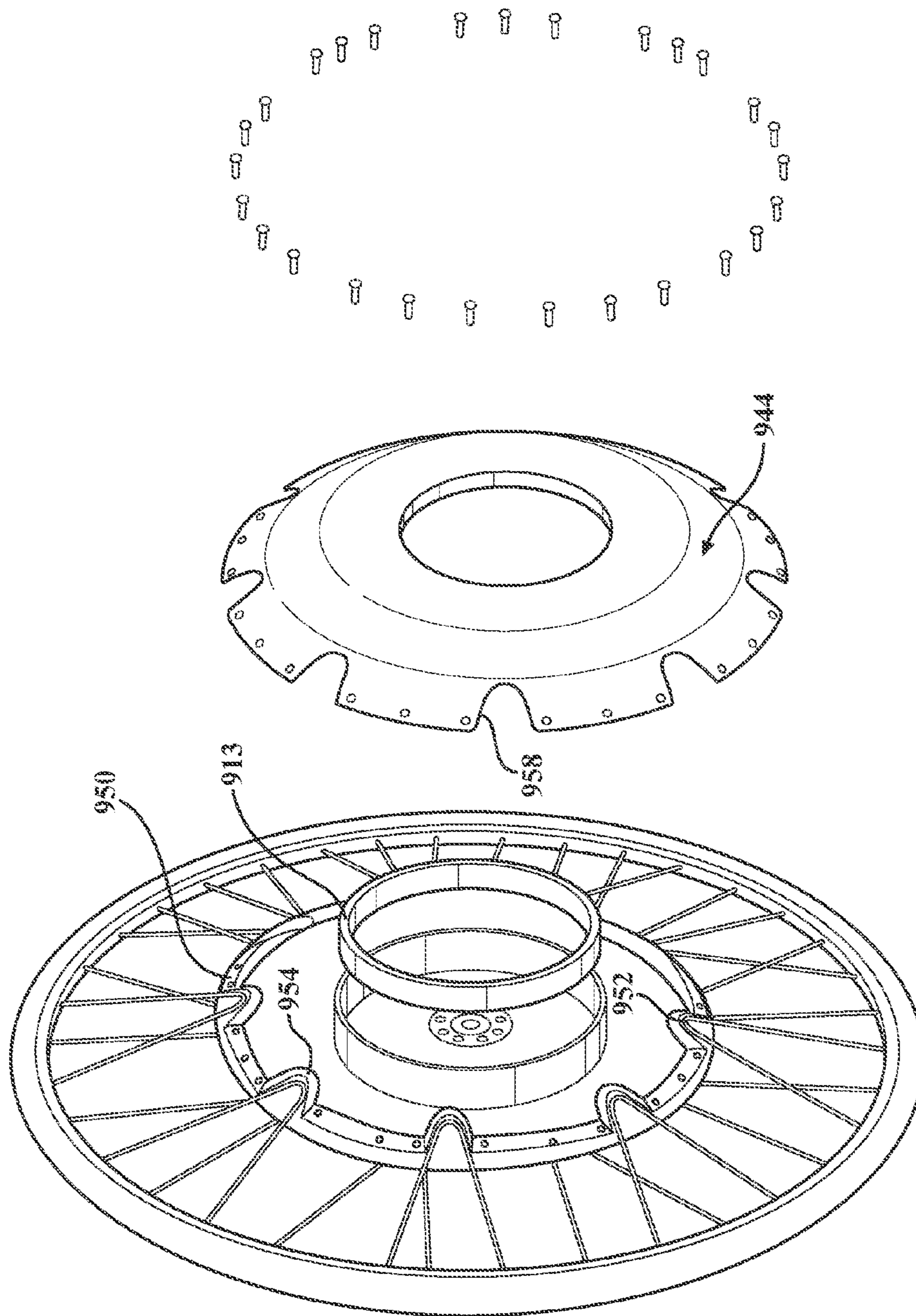
FIG. 9I
