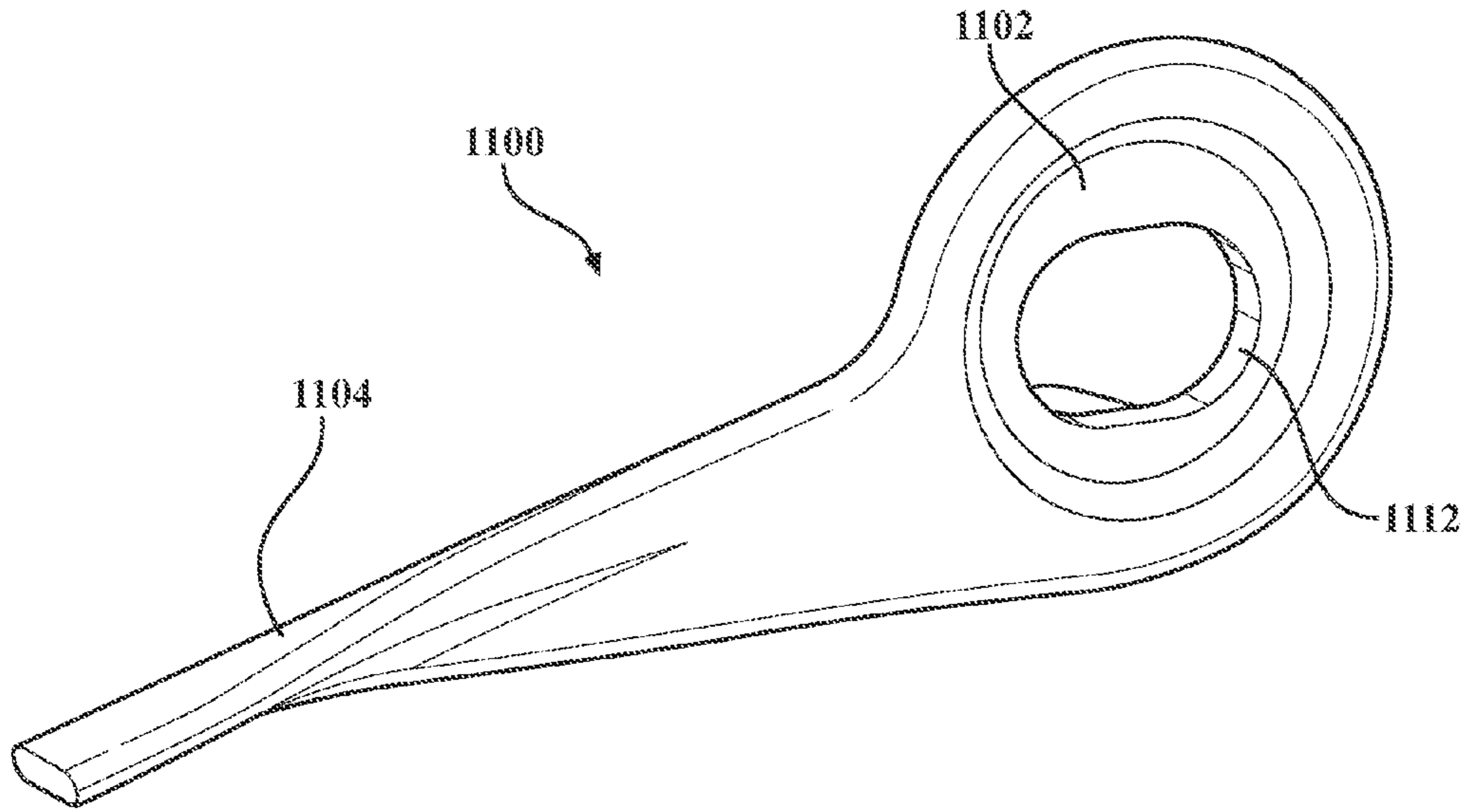
FIG. 11C
