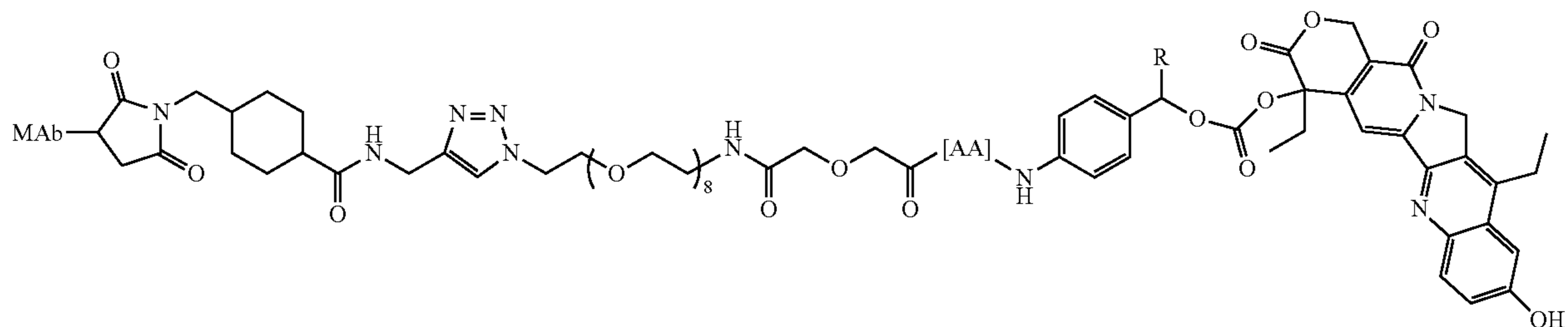
MAb-CLX-SN-38
