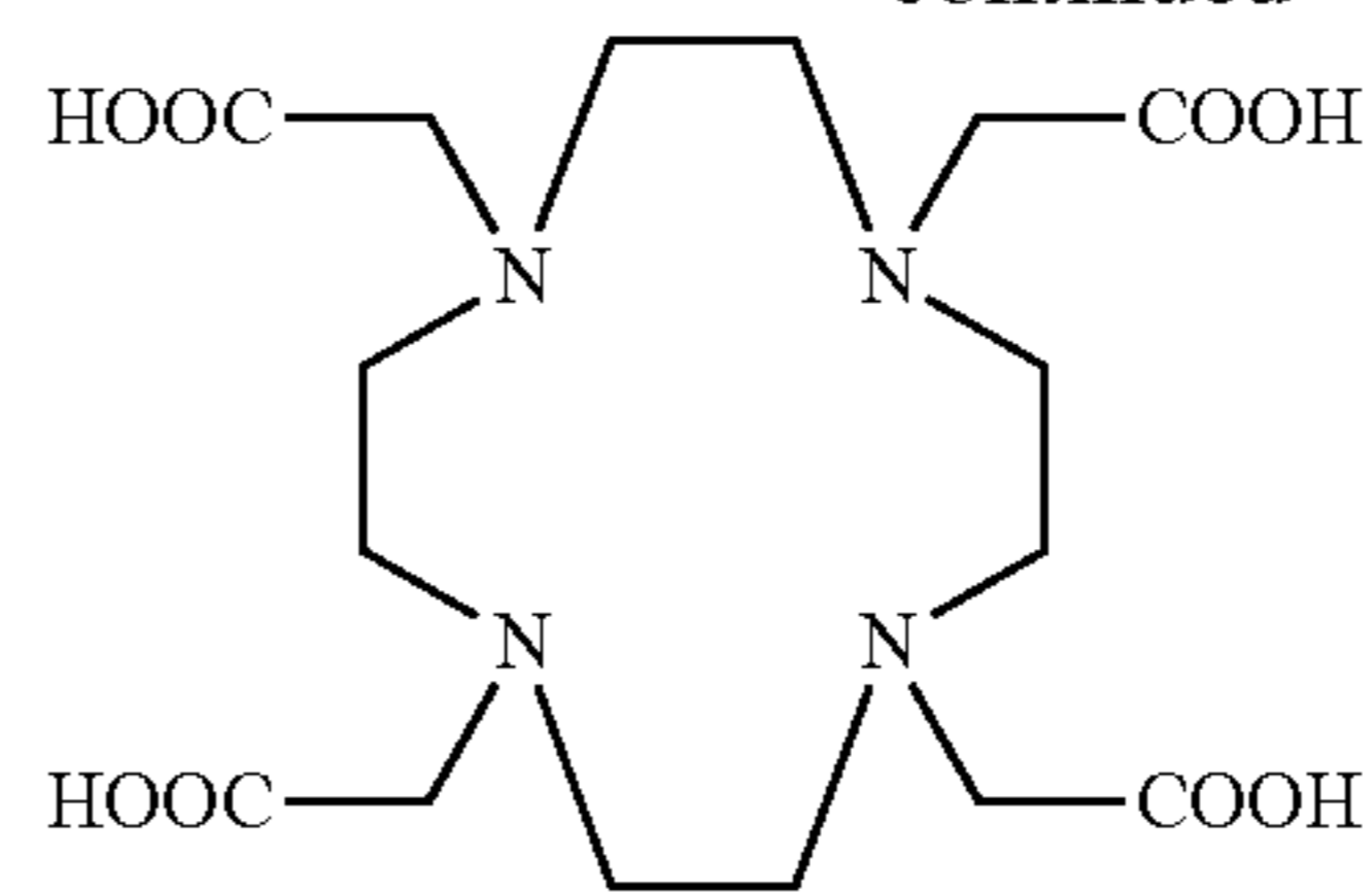
DOTA
