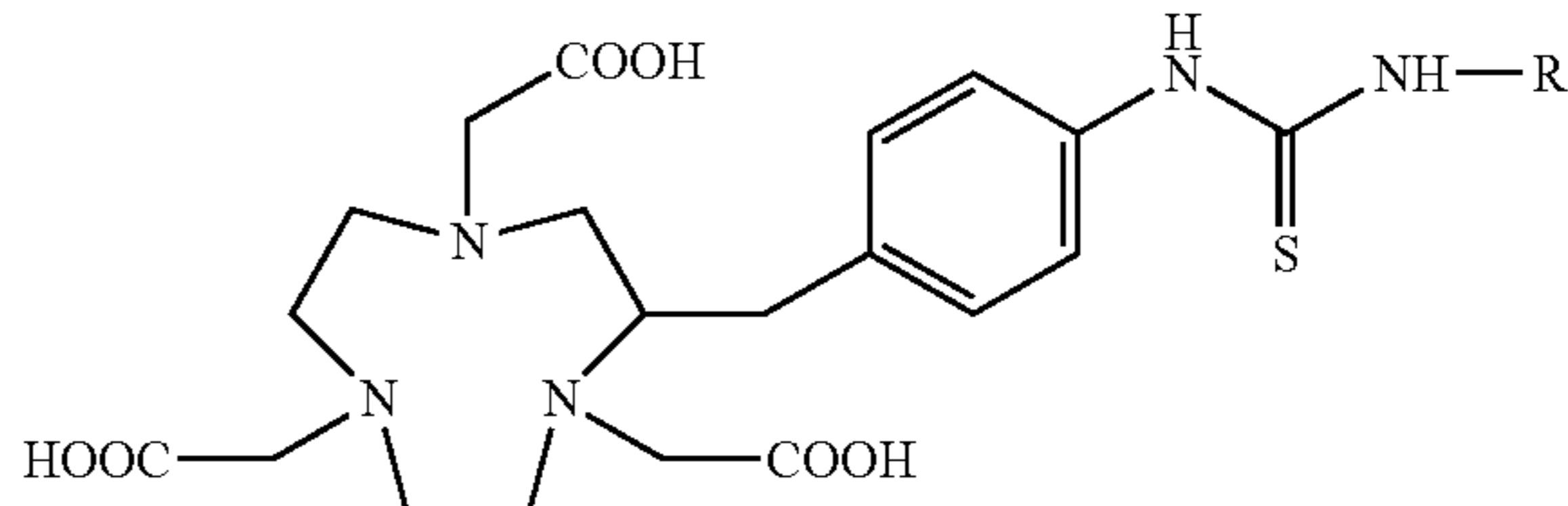
NOTA-Bn-R
