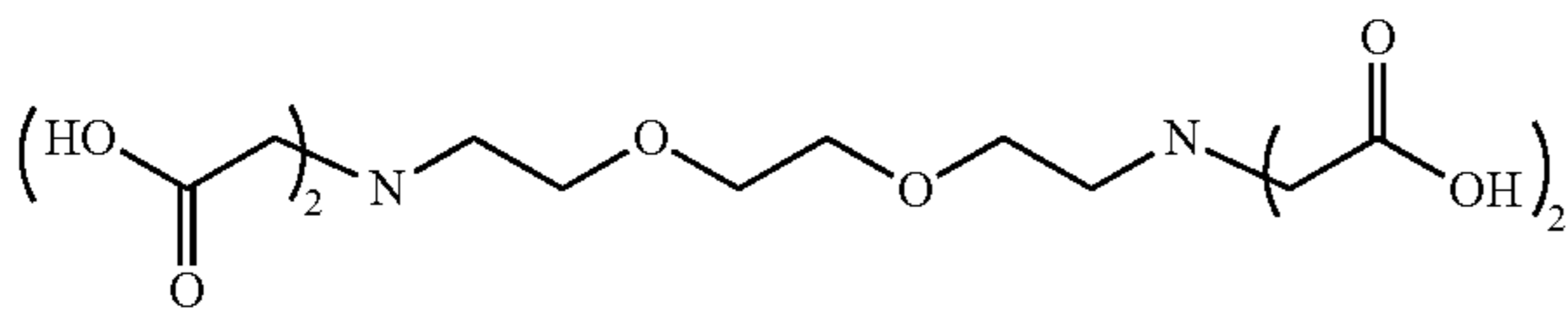
EGTA
