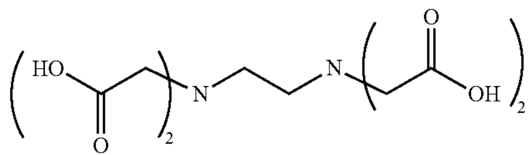
EDTA
