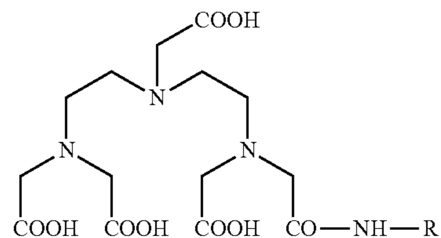
DPTA-monoamide
