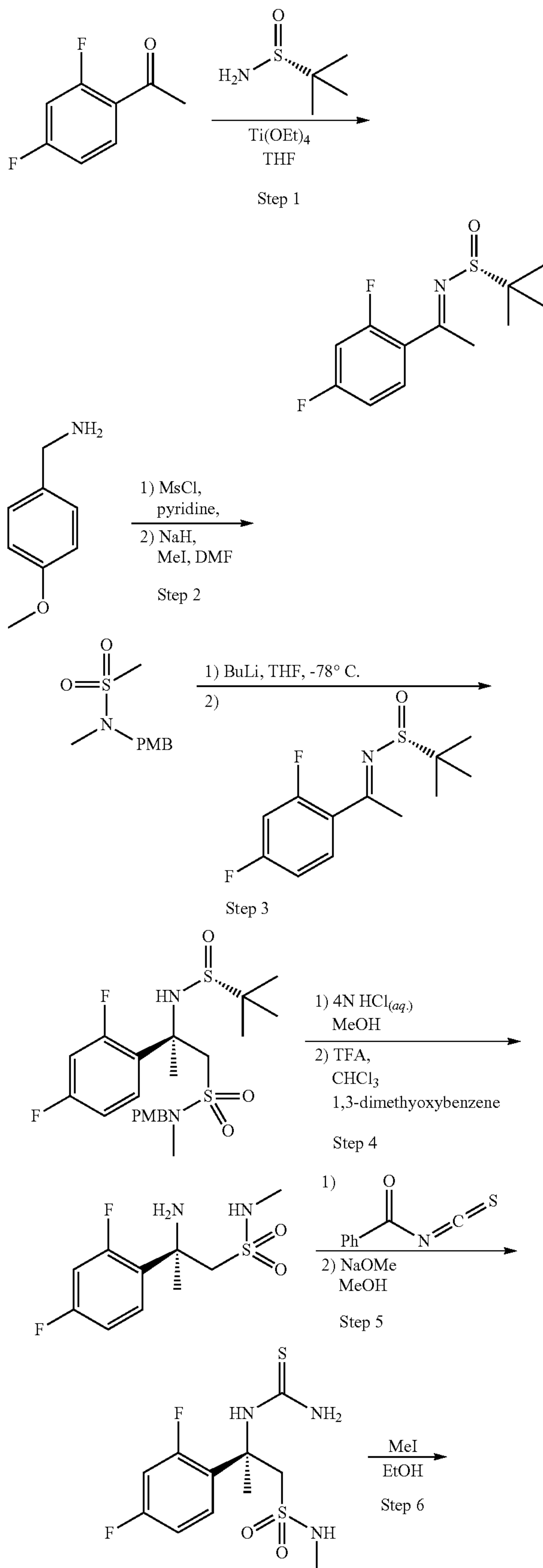
Scheme 1a
