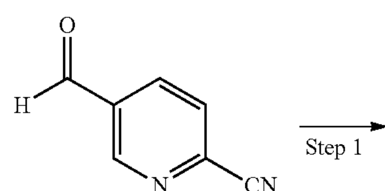
Scheme 11ab:
