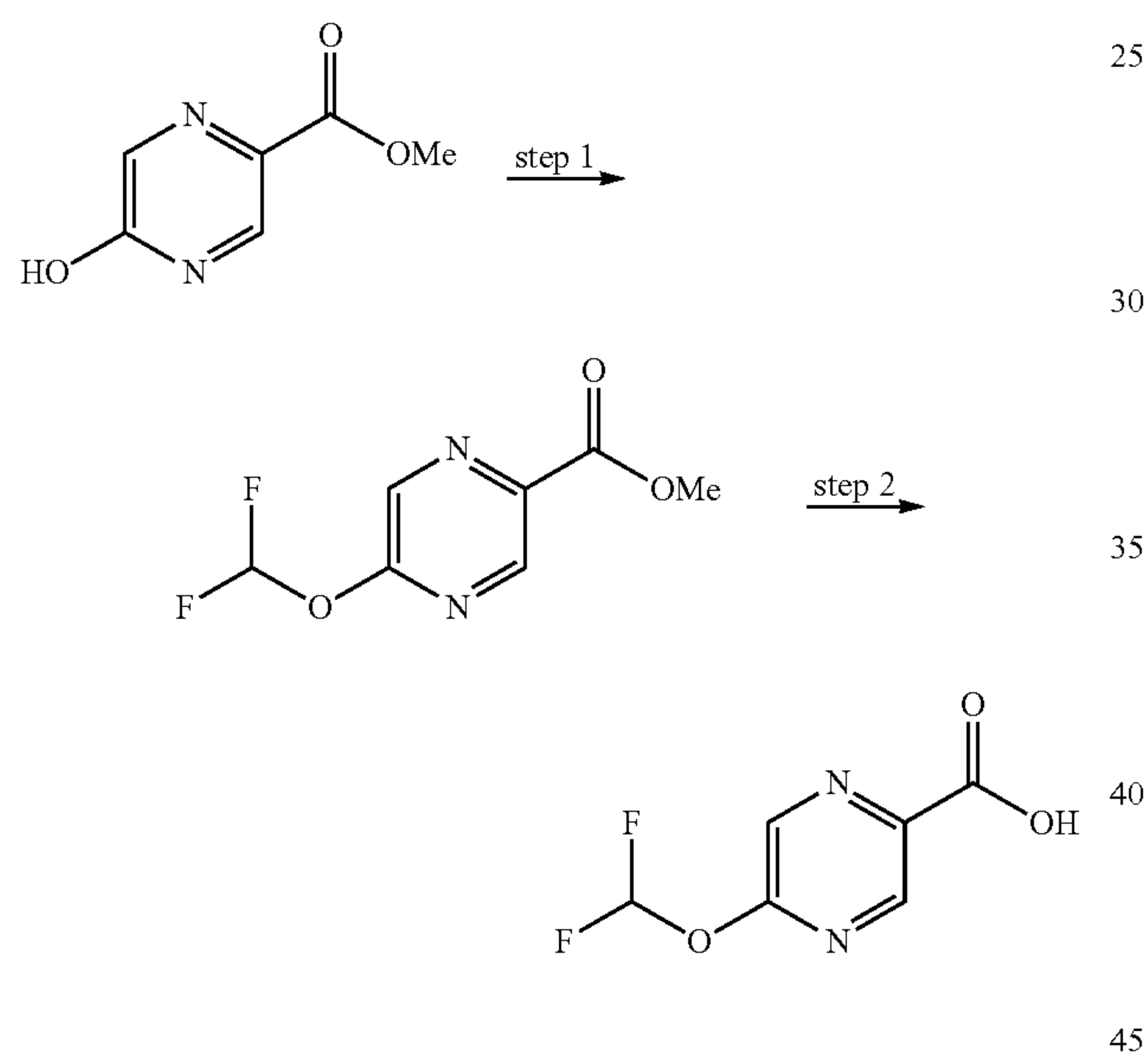
Scheme 11j:
