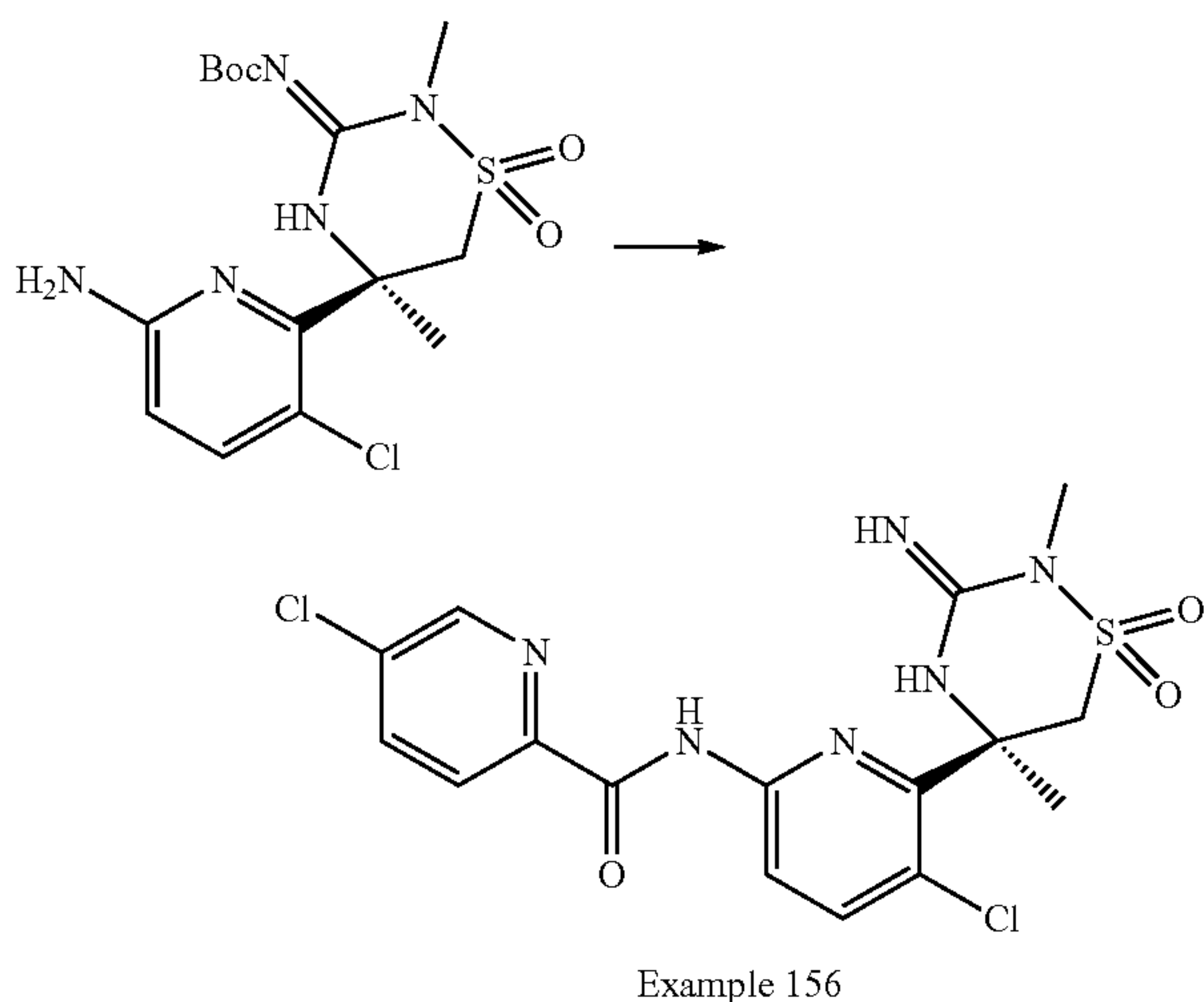
Scheme 37:
