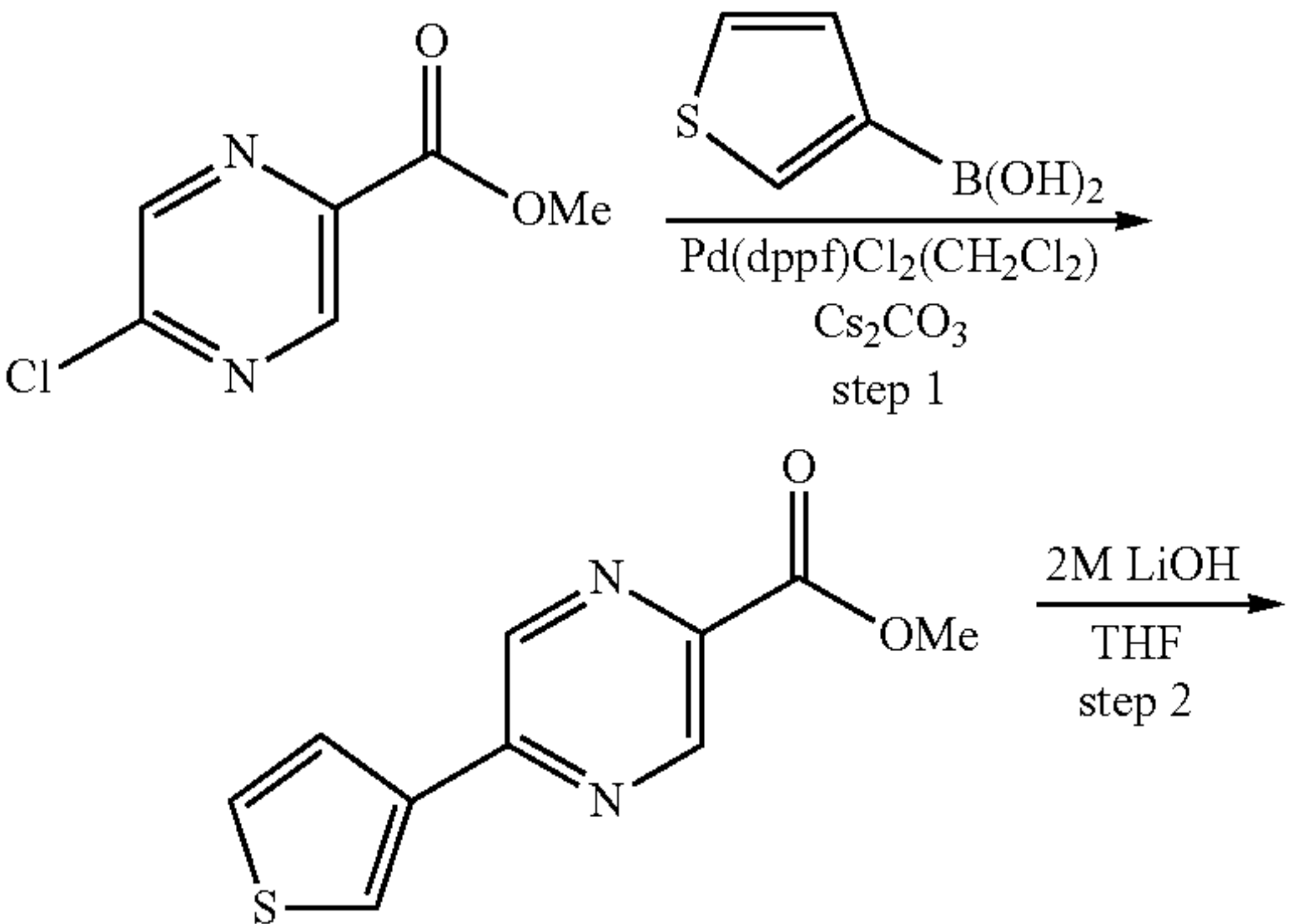
Scheme 11e:
