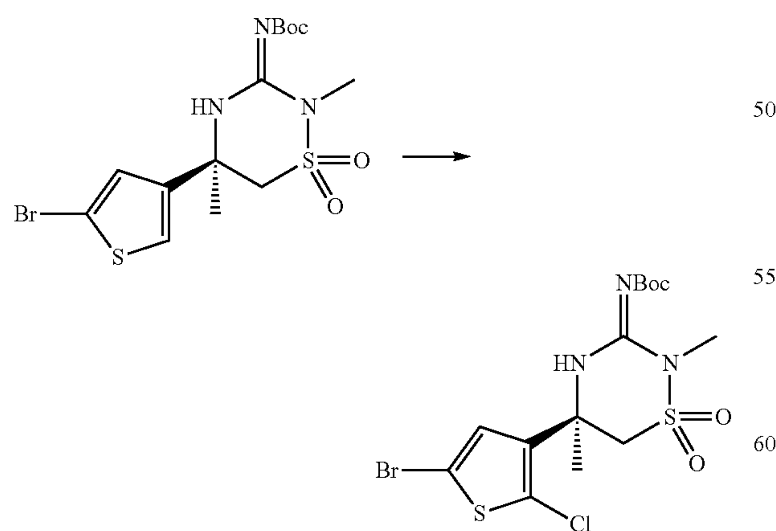
Scheme 9a:
