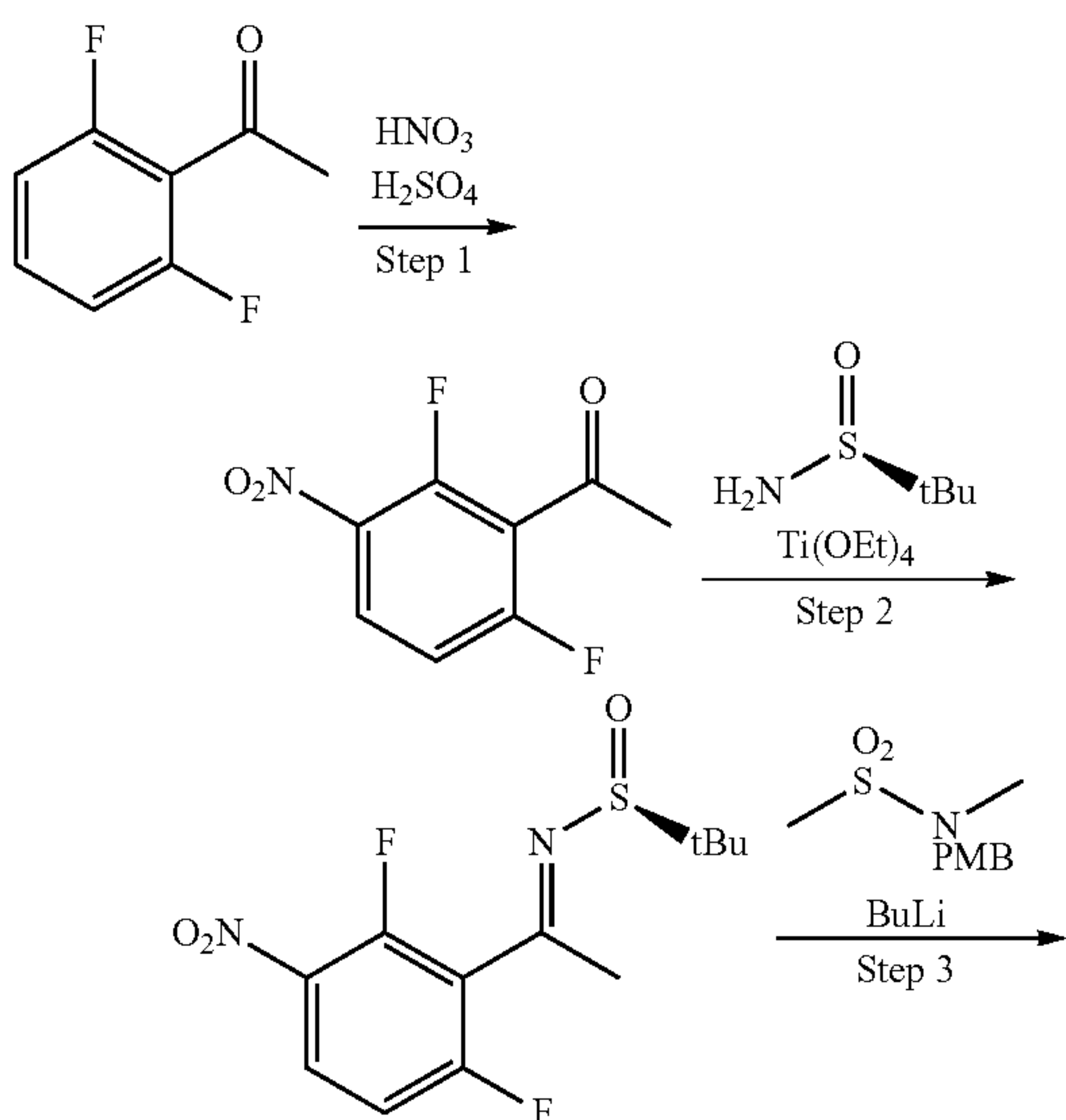
Scheme 43:
