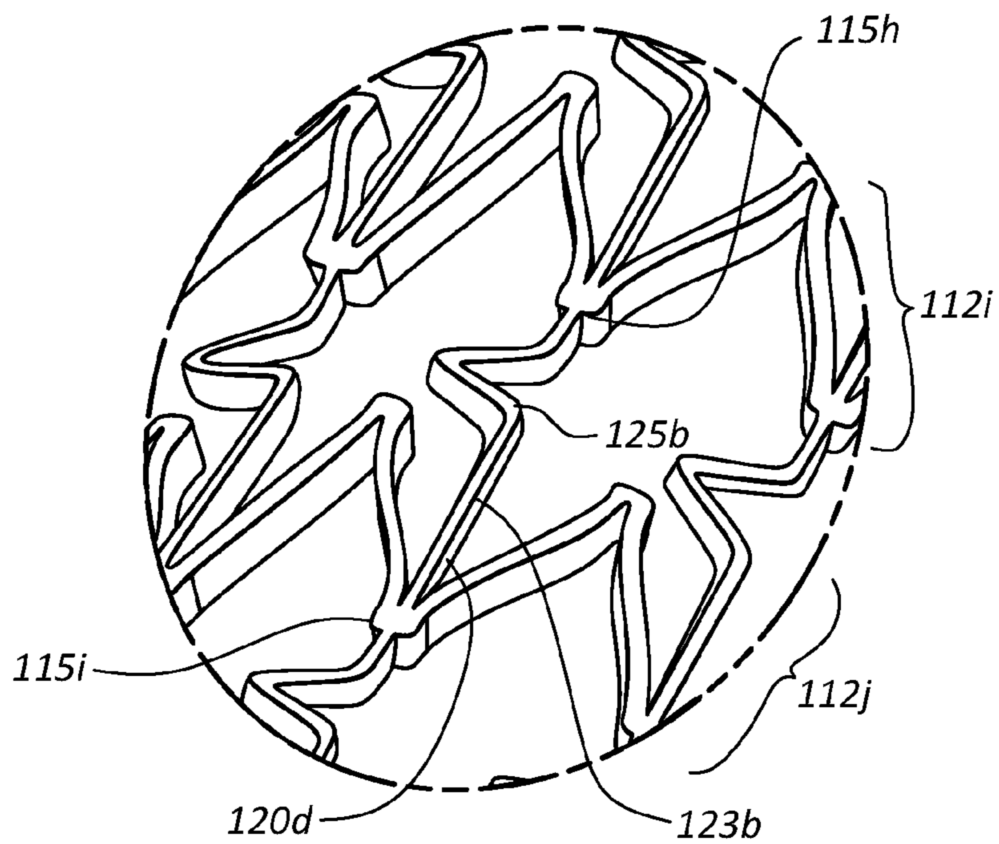
FIG. 1E
