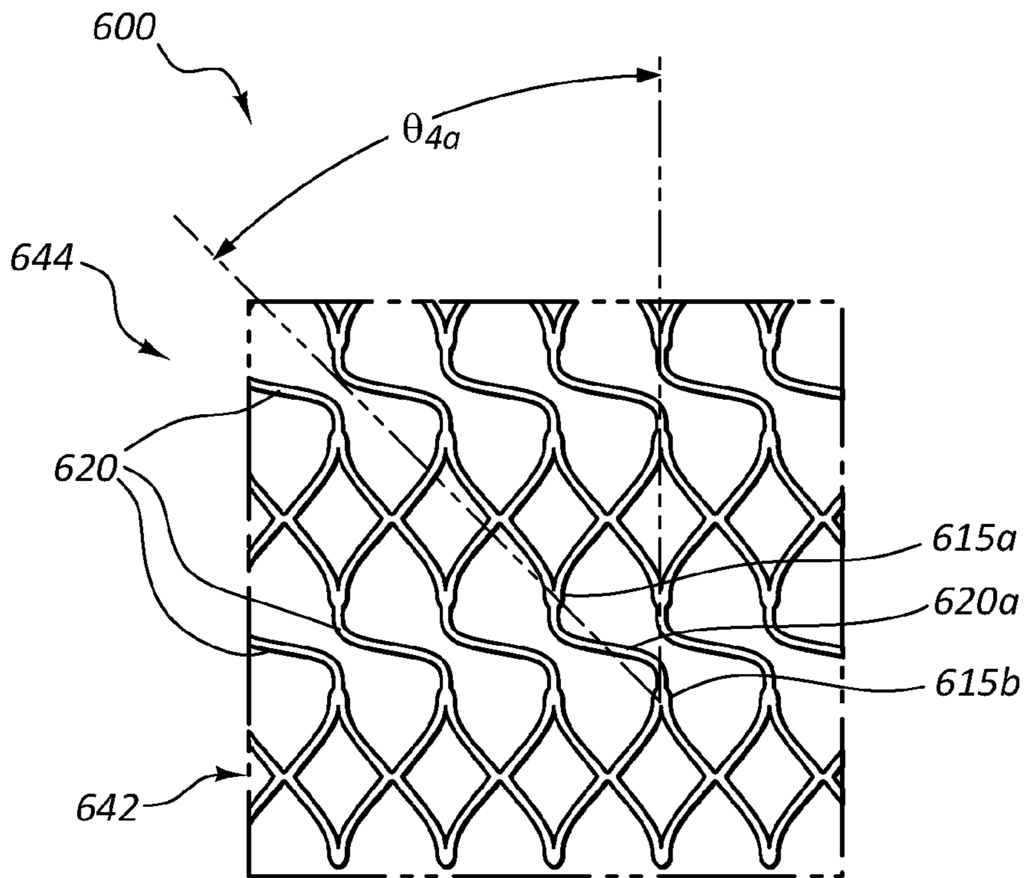
FIG. 6A
