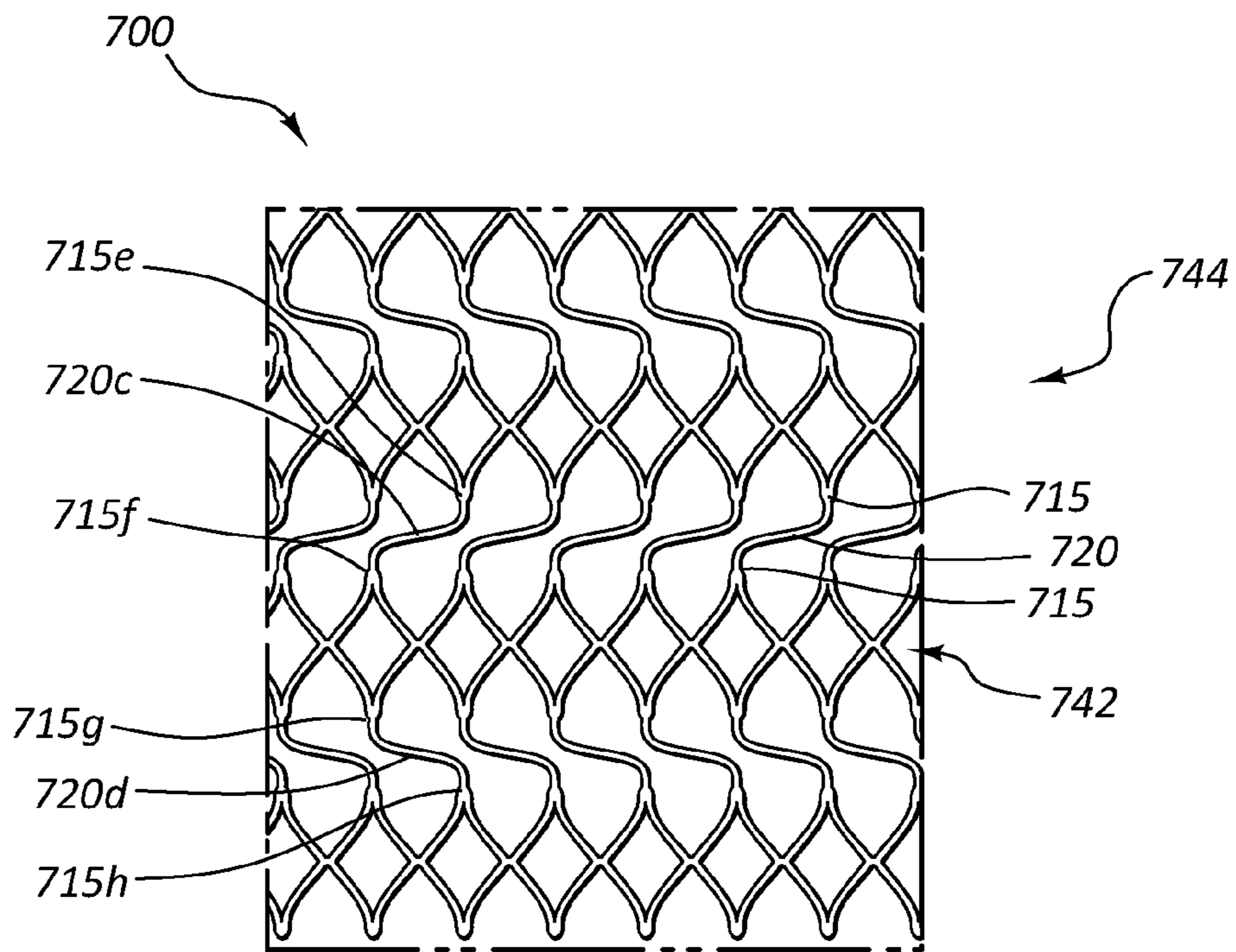
FIG. 7B
