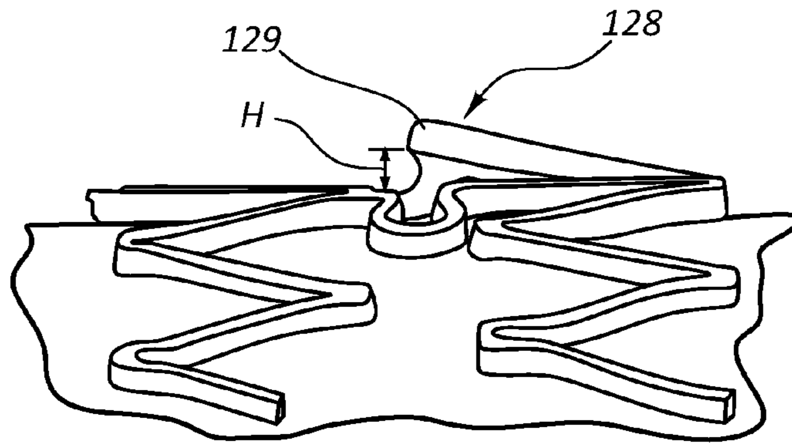
FIG. 1G
