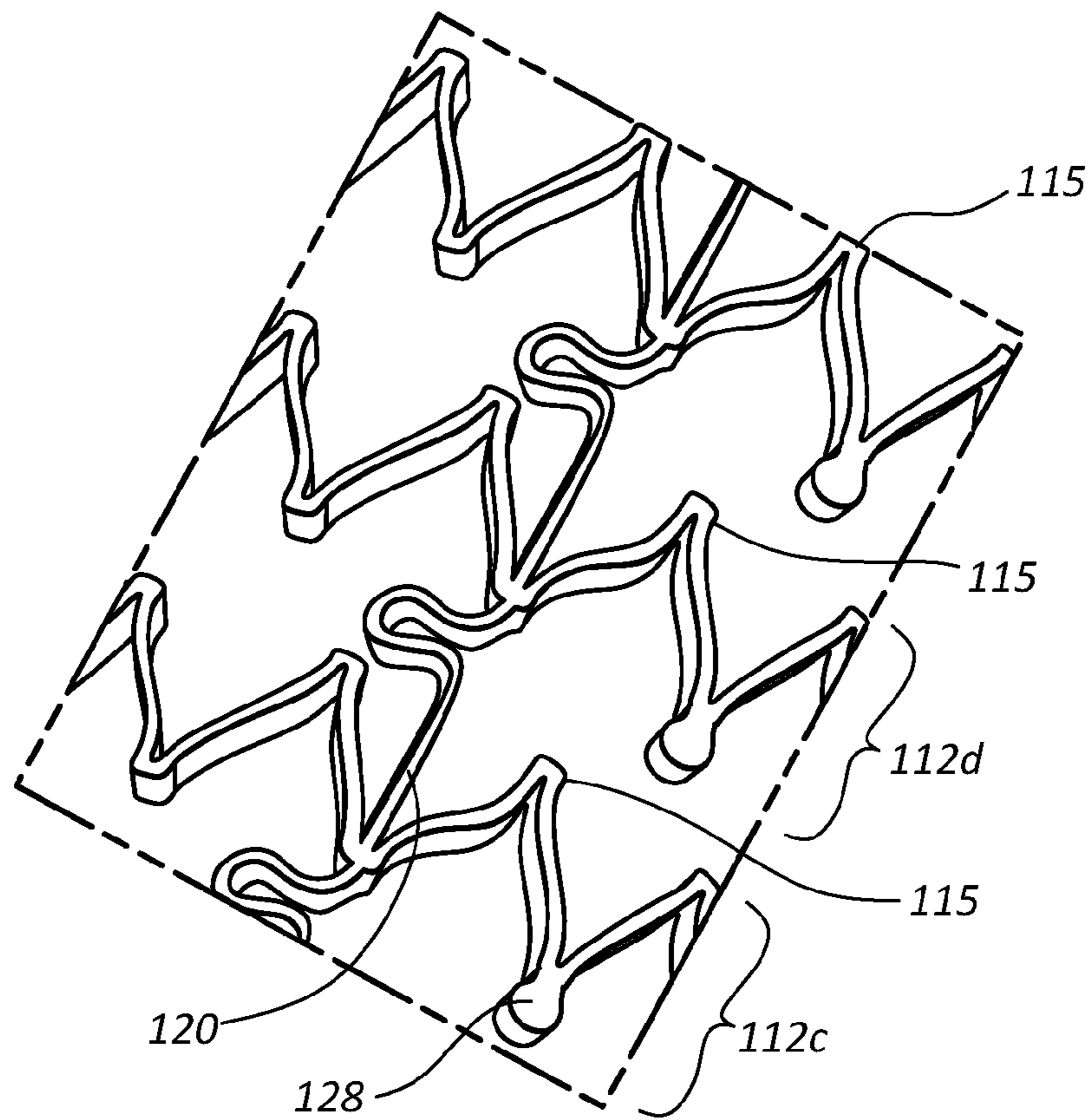
FIG. 1B
