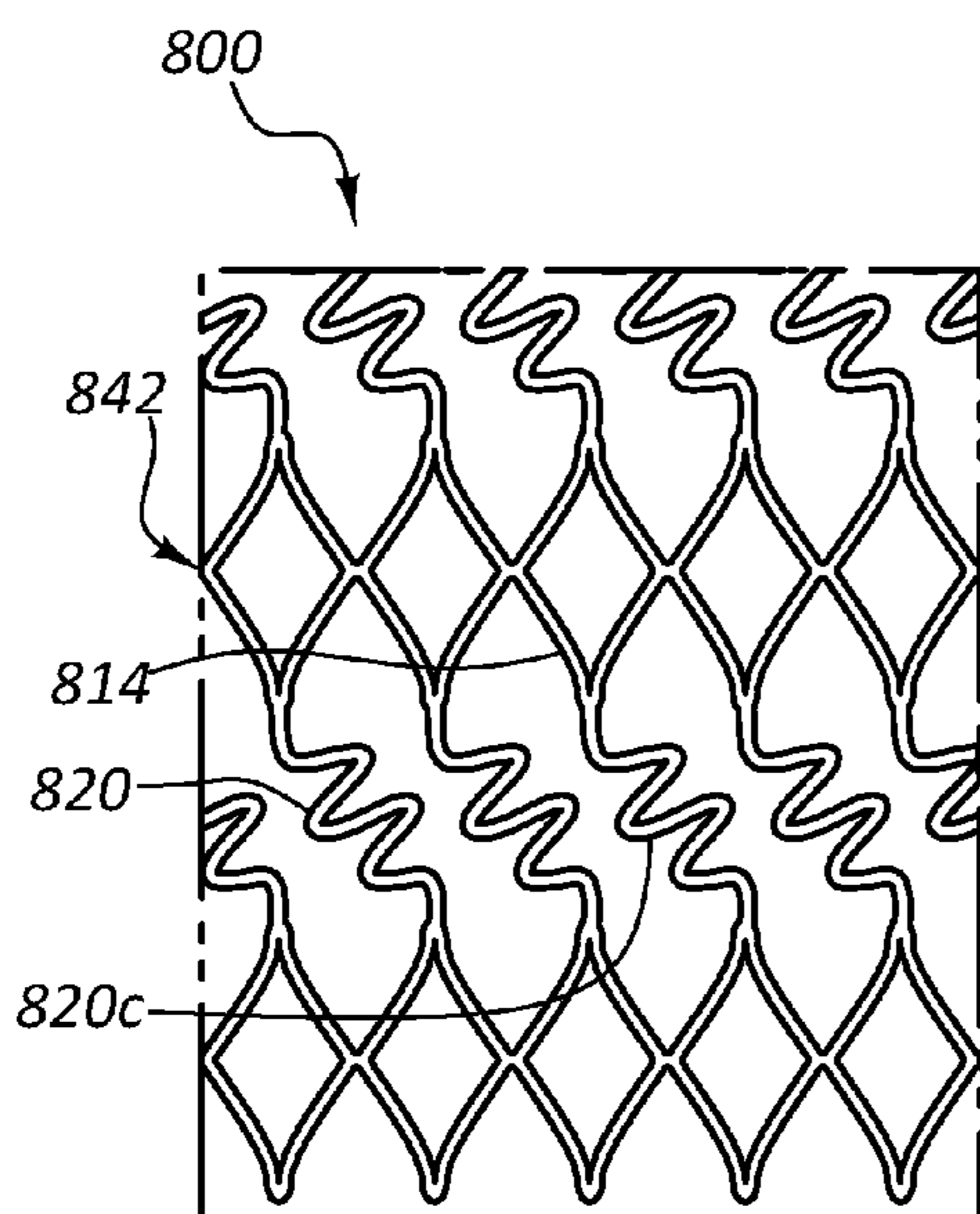
FIG. 8A
