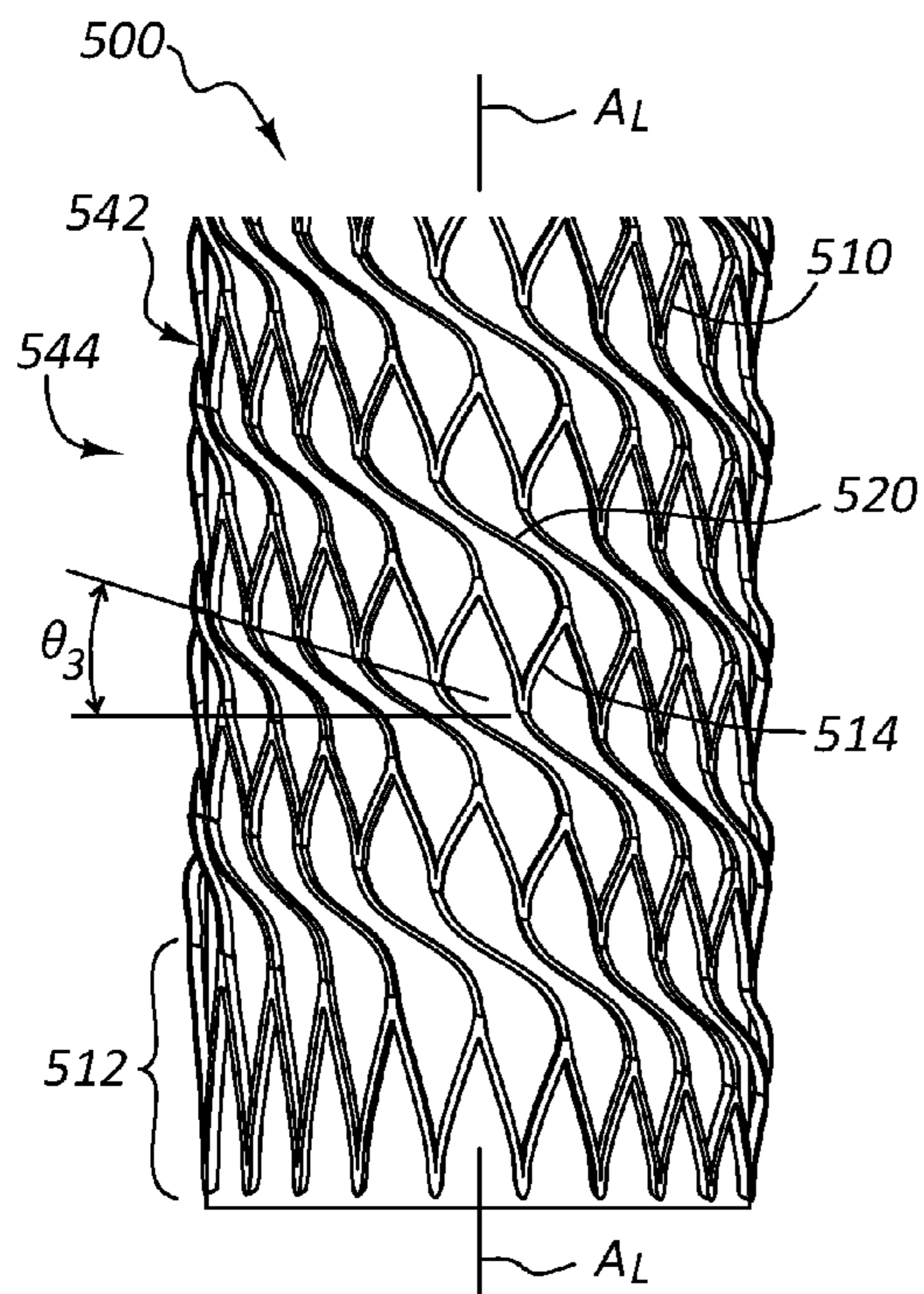
FIG. 5A
