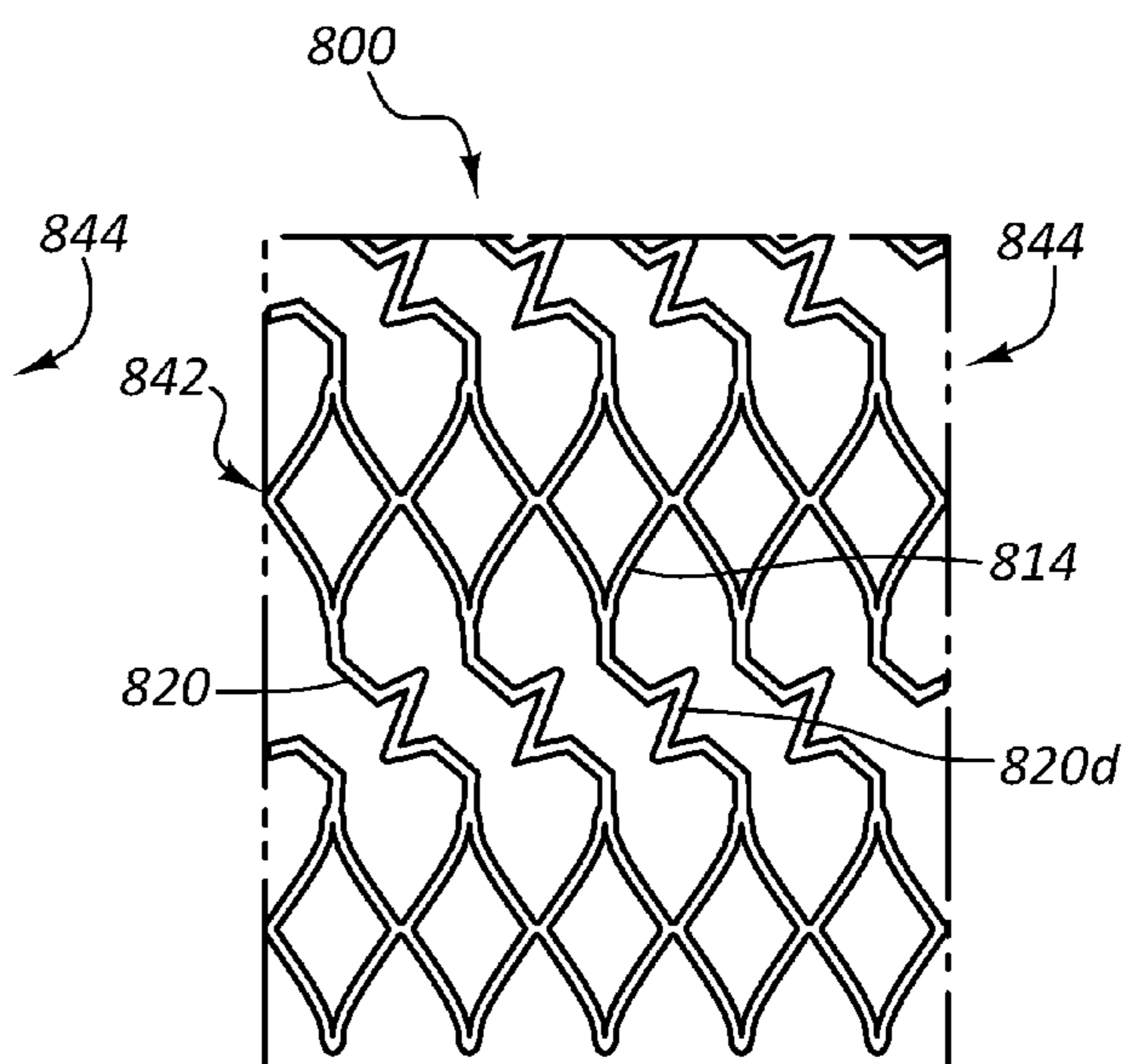
FIG. 8B
