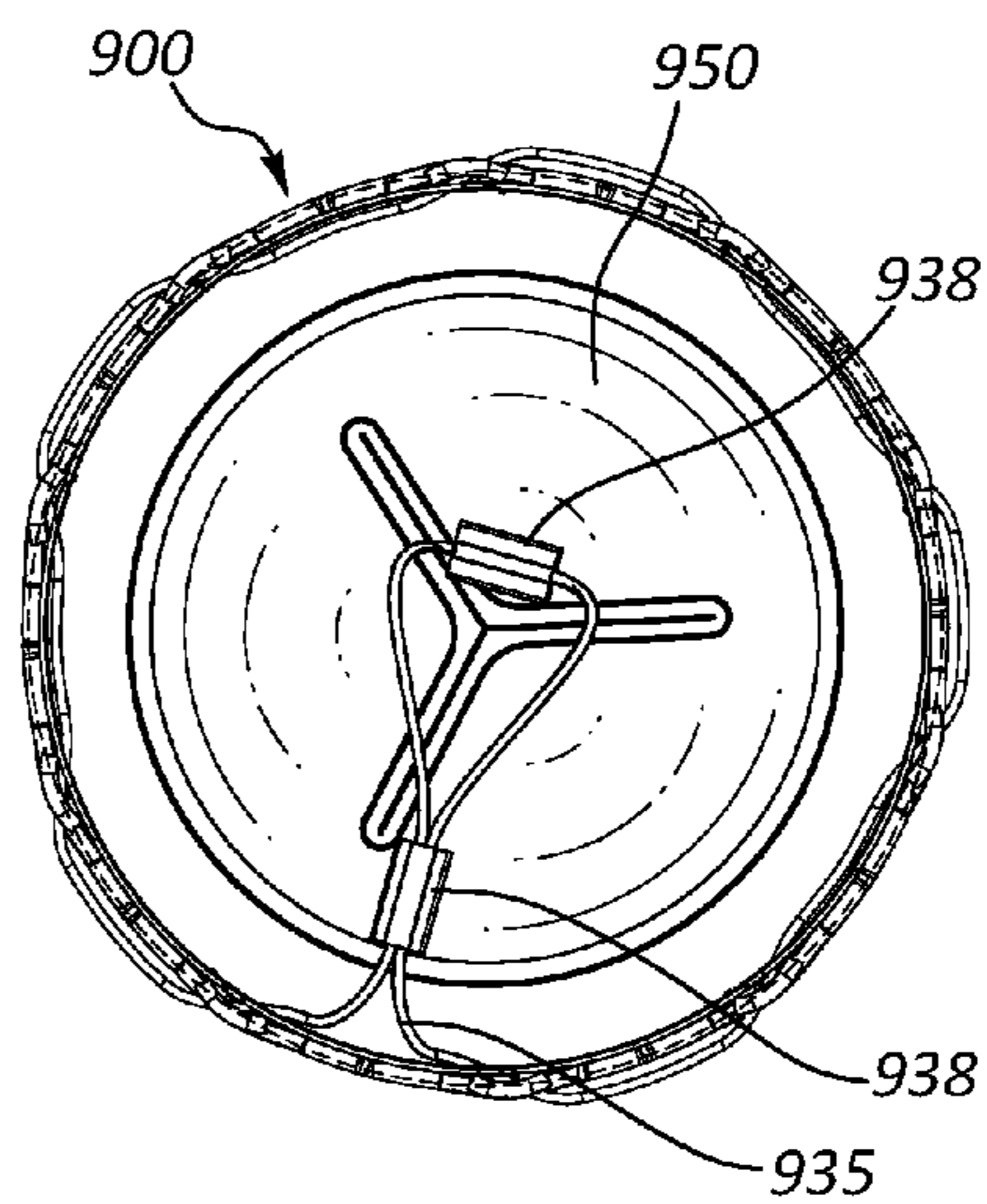
FIG. 9A
