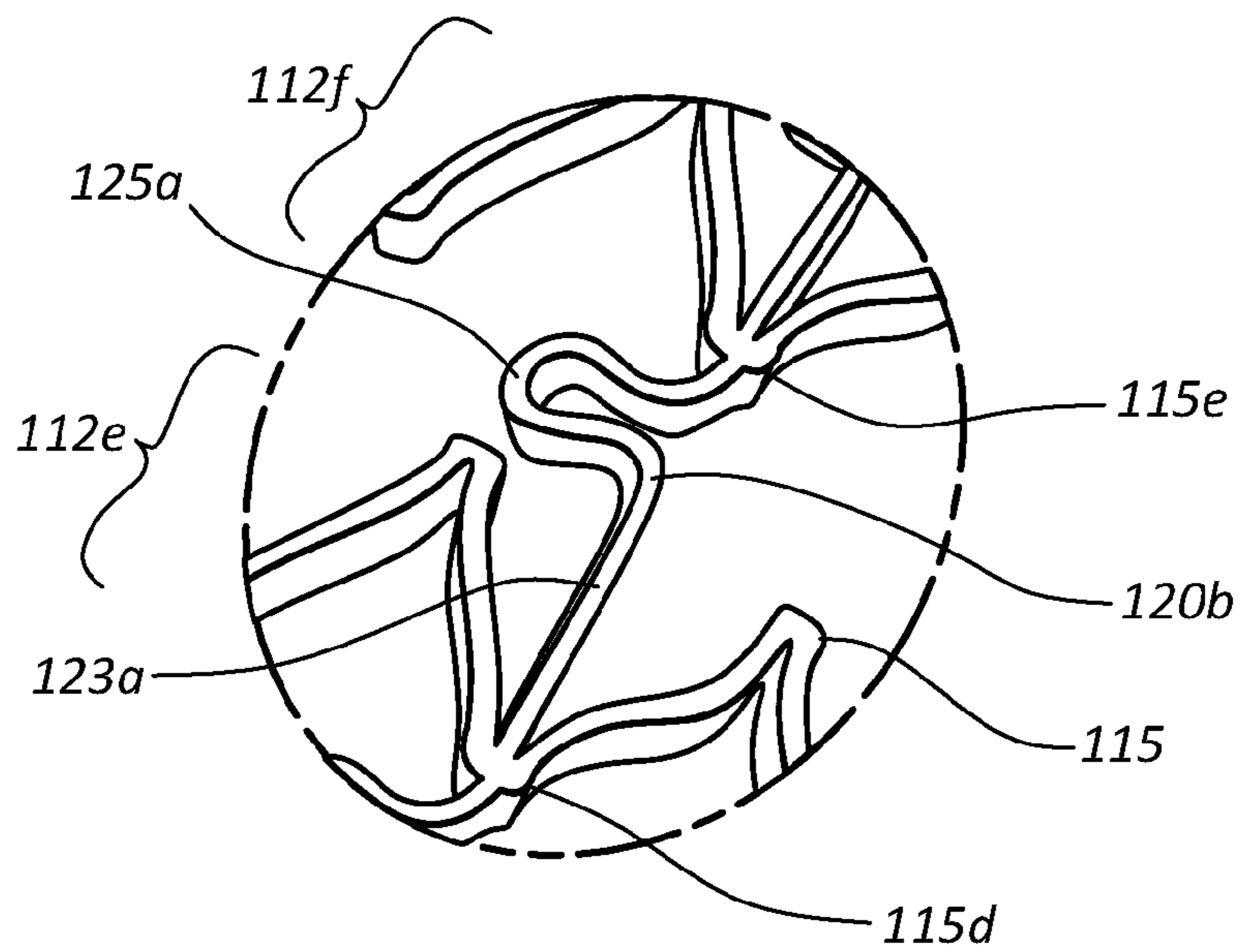
FIG. 1C
