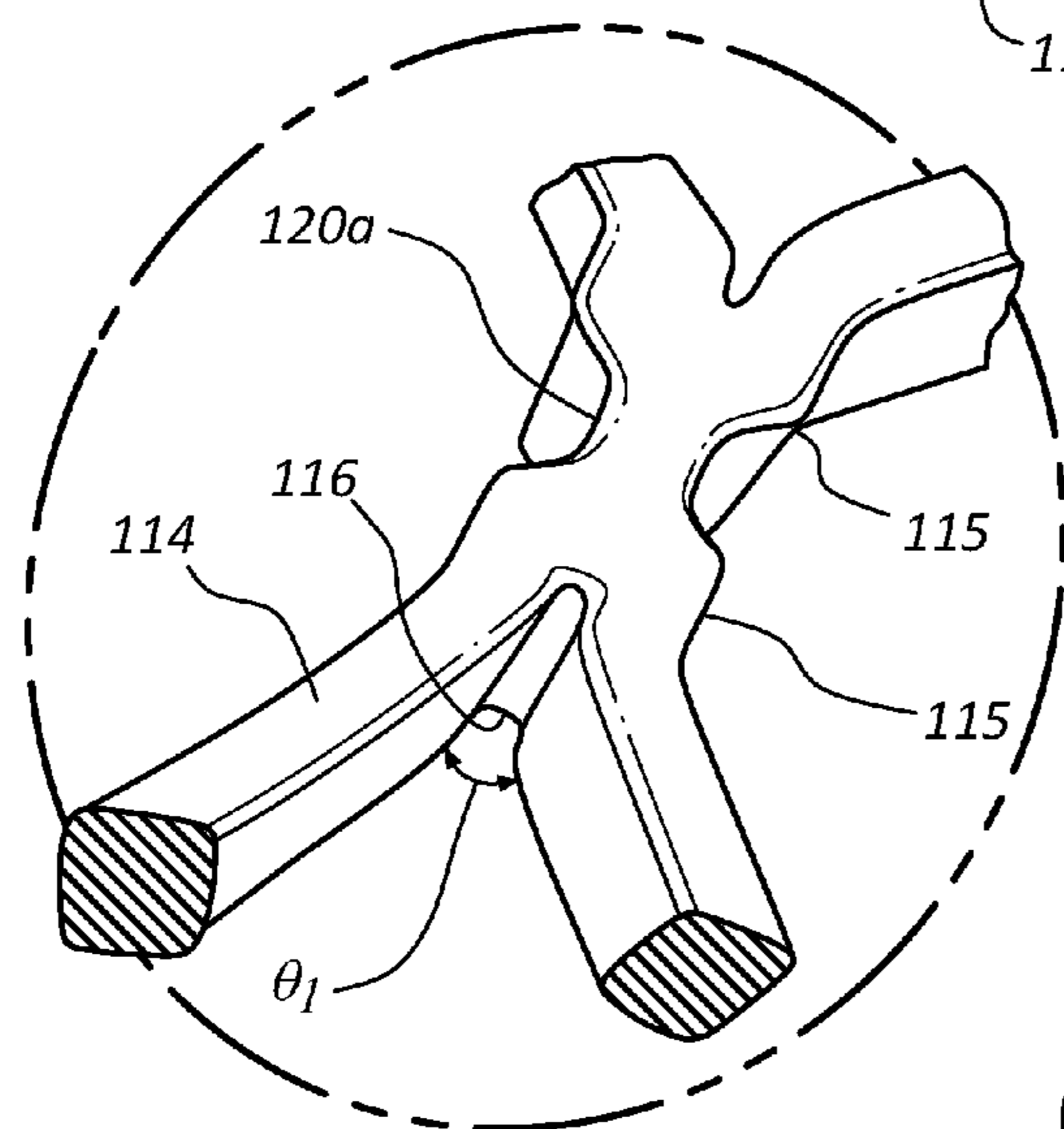
FIG. 1AB
