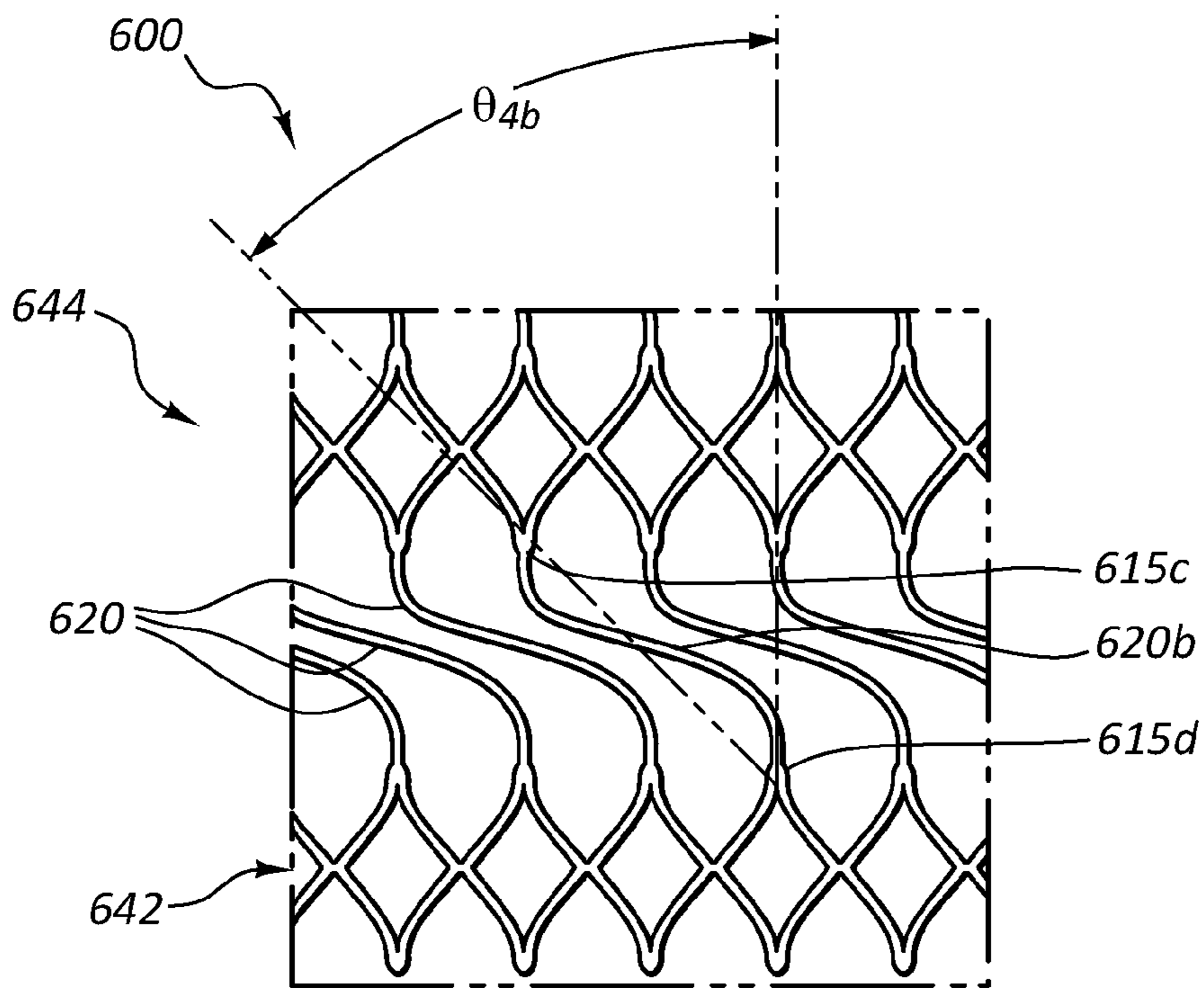
FIG. 6B
