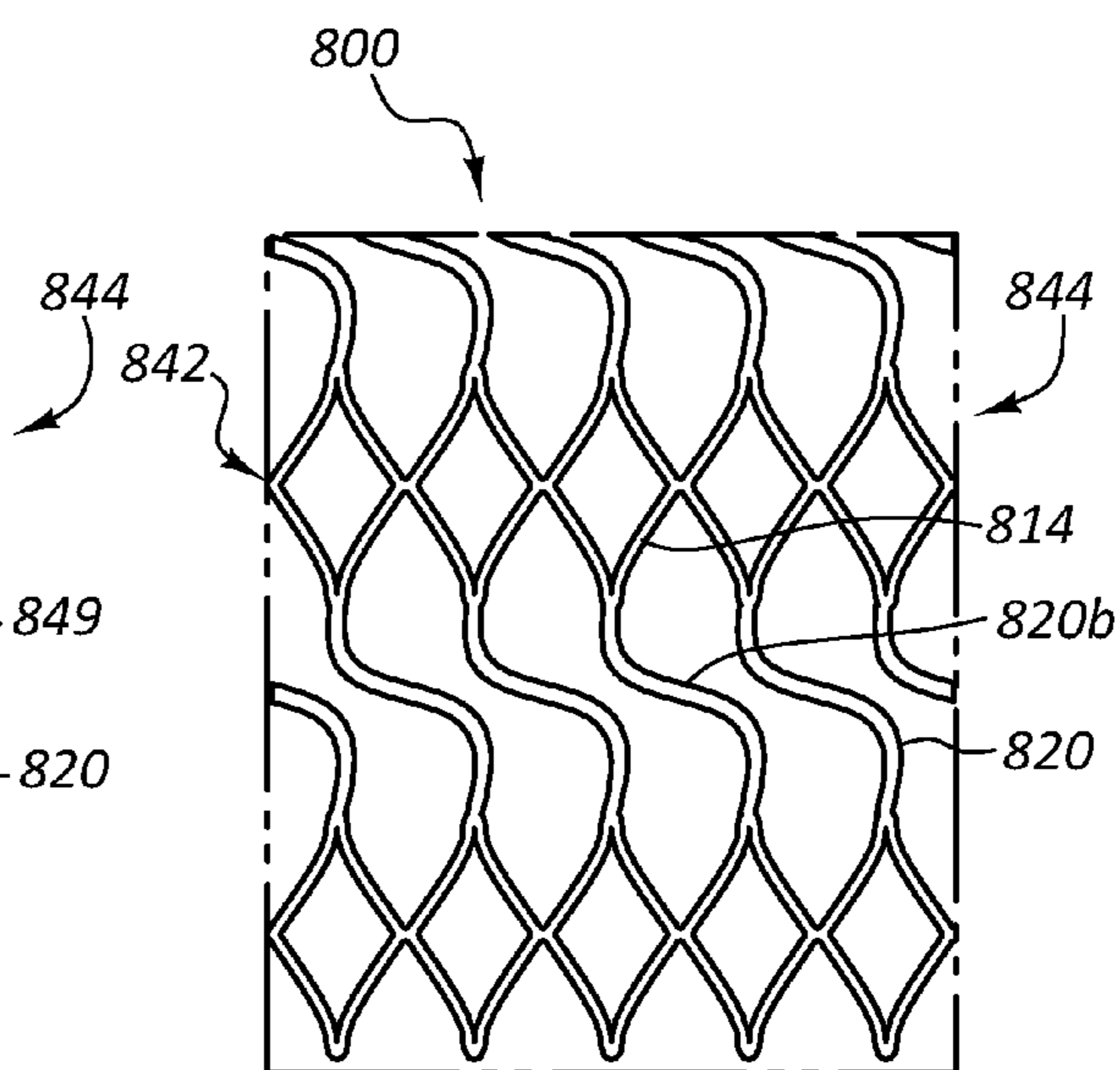
FIG. 8B
