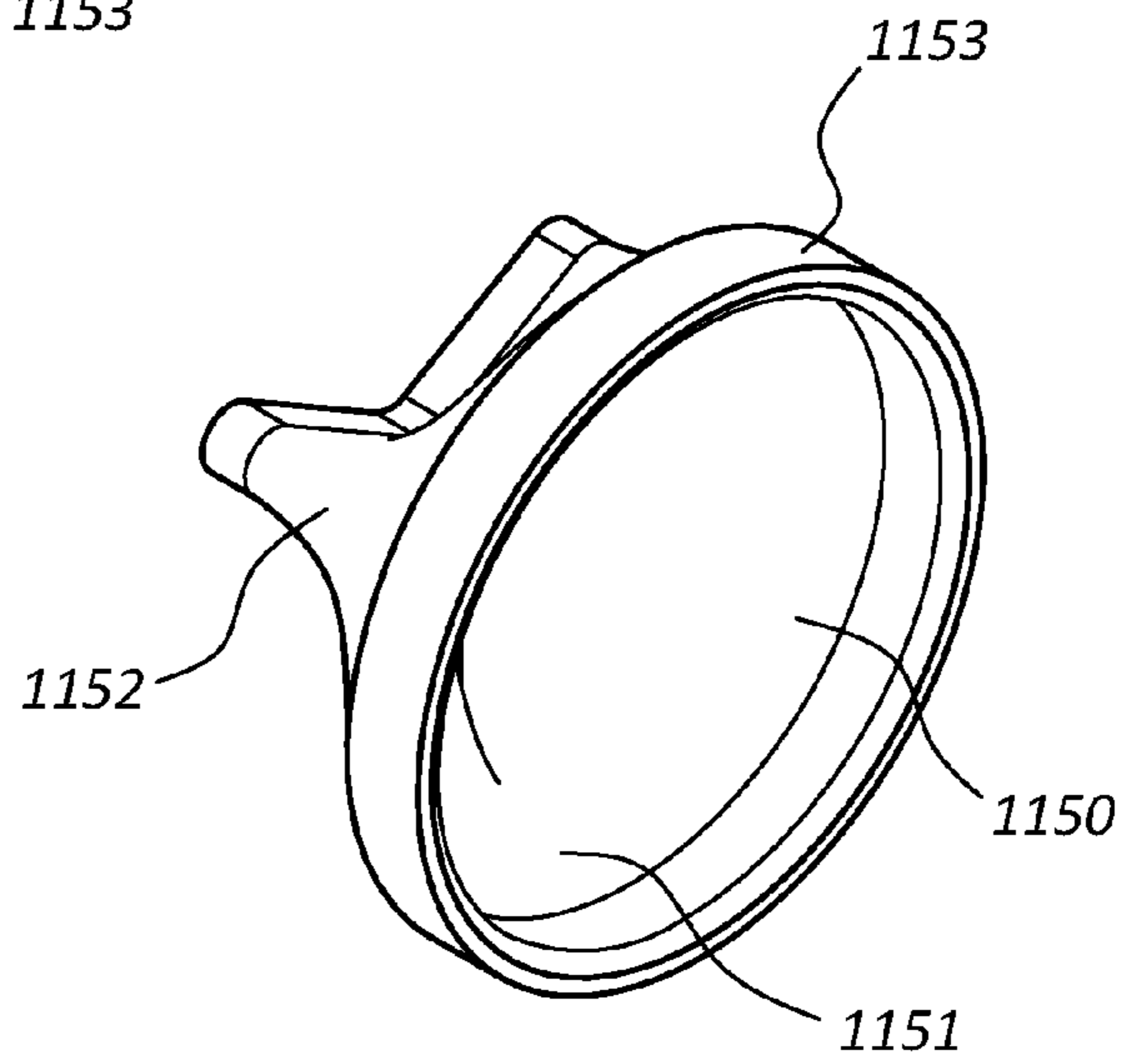
FIG. 11B
