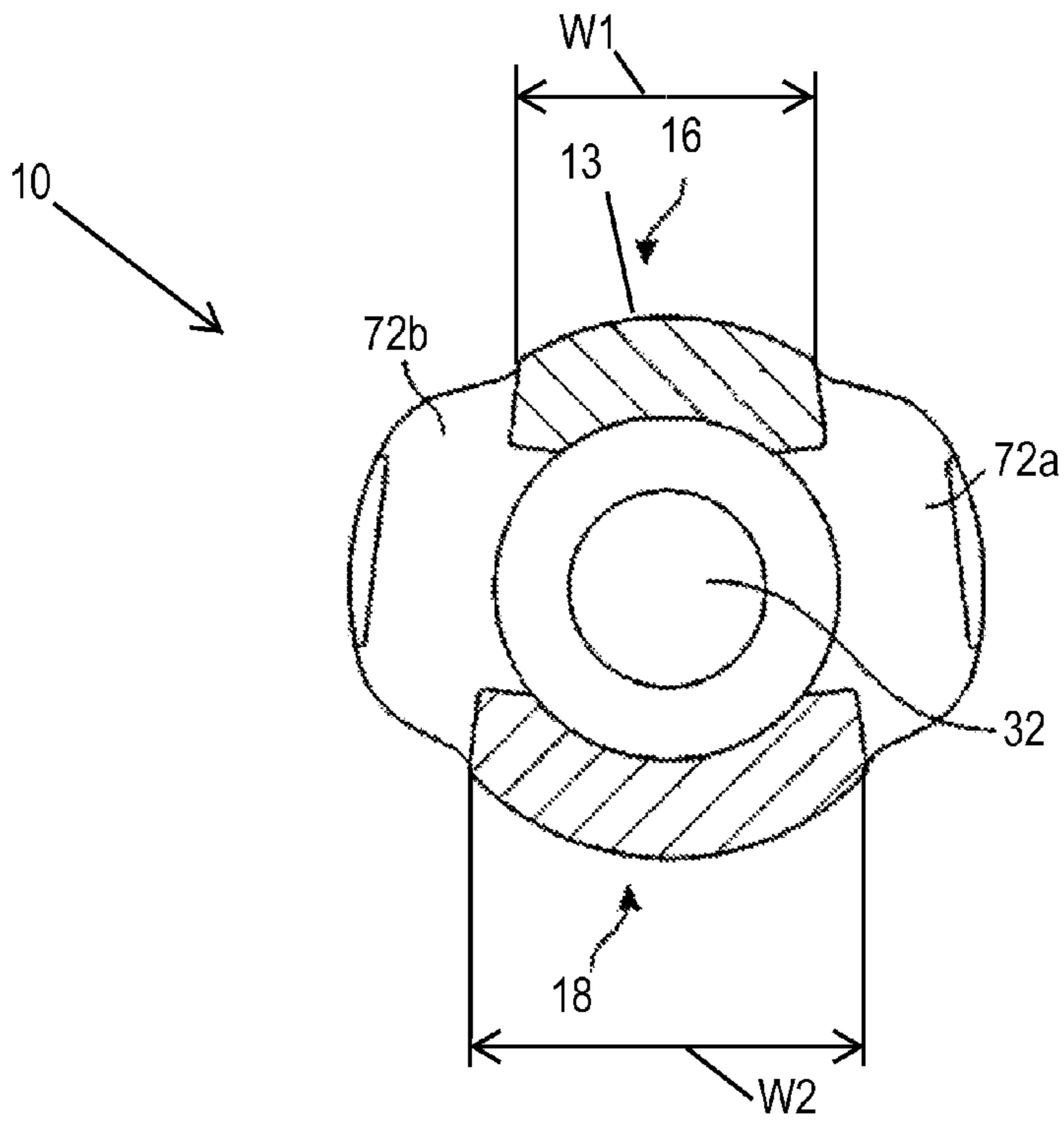
FIG. 8
