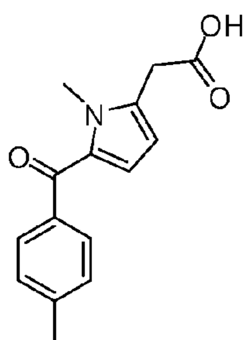
Tolmetin
