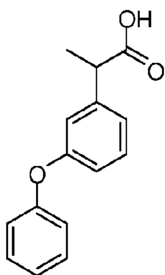
Fenopropfen
