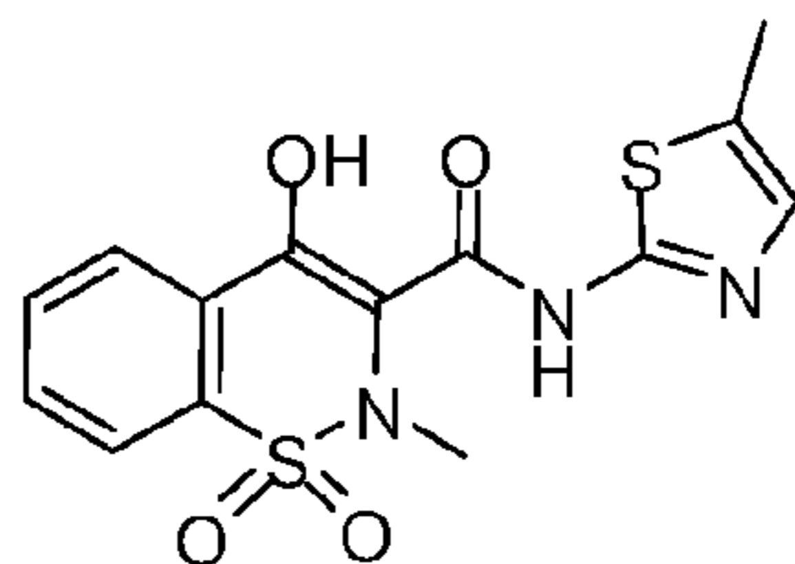
Meloxicam
