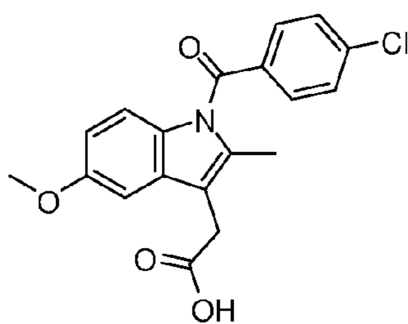
Indomethacin
