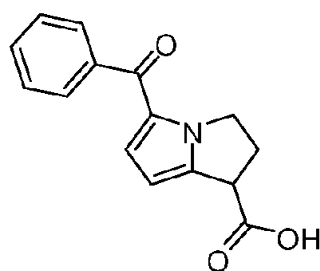
Ketorolac
