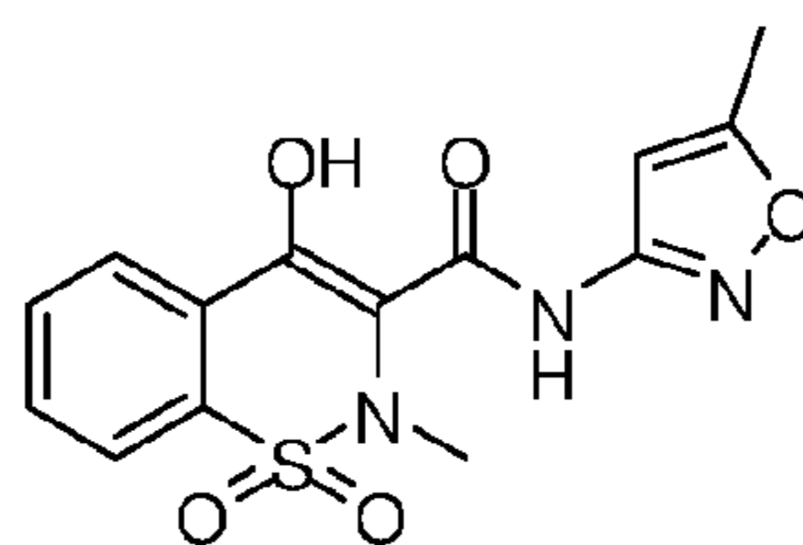
Isoxicam
