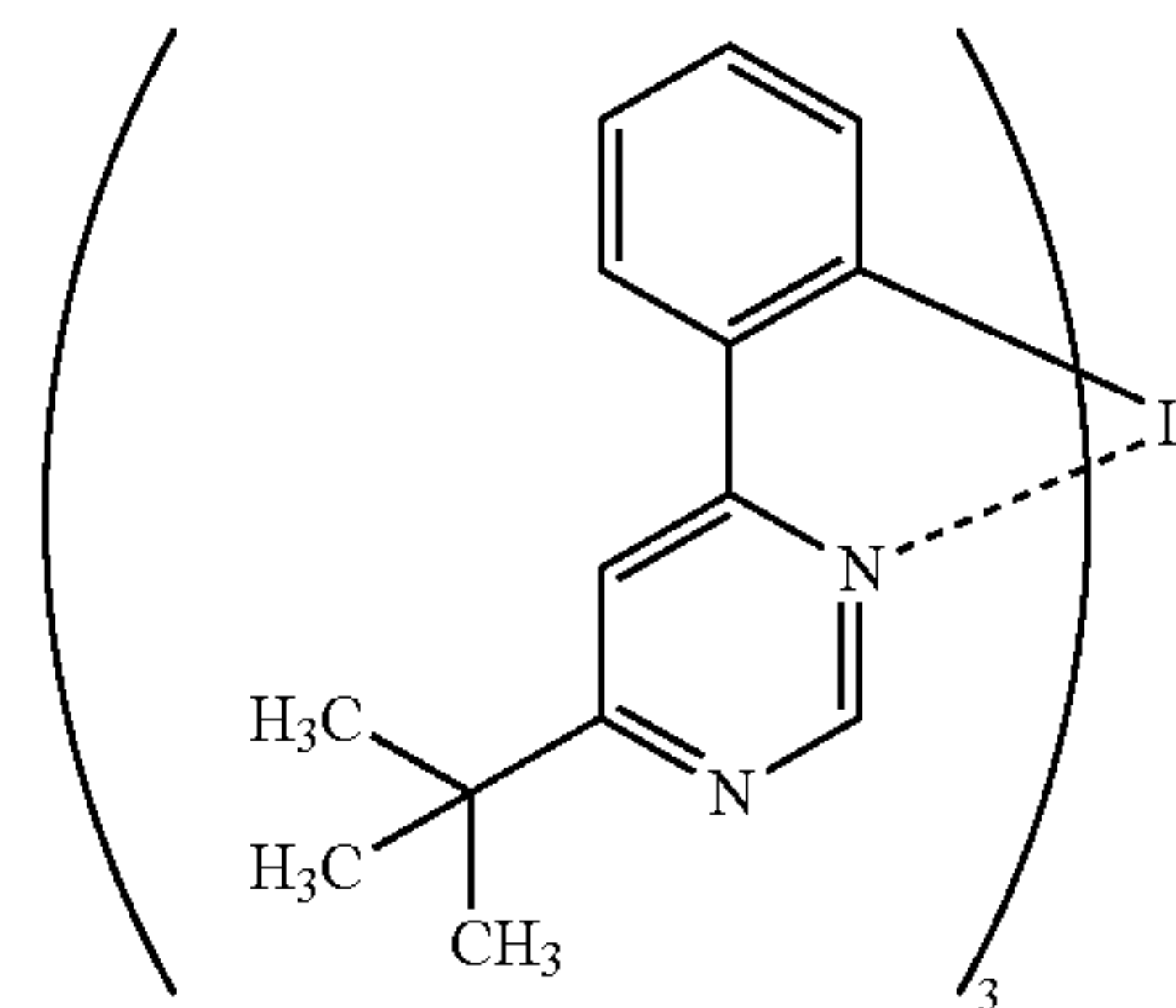
Ir(tBuppm) 3
