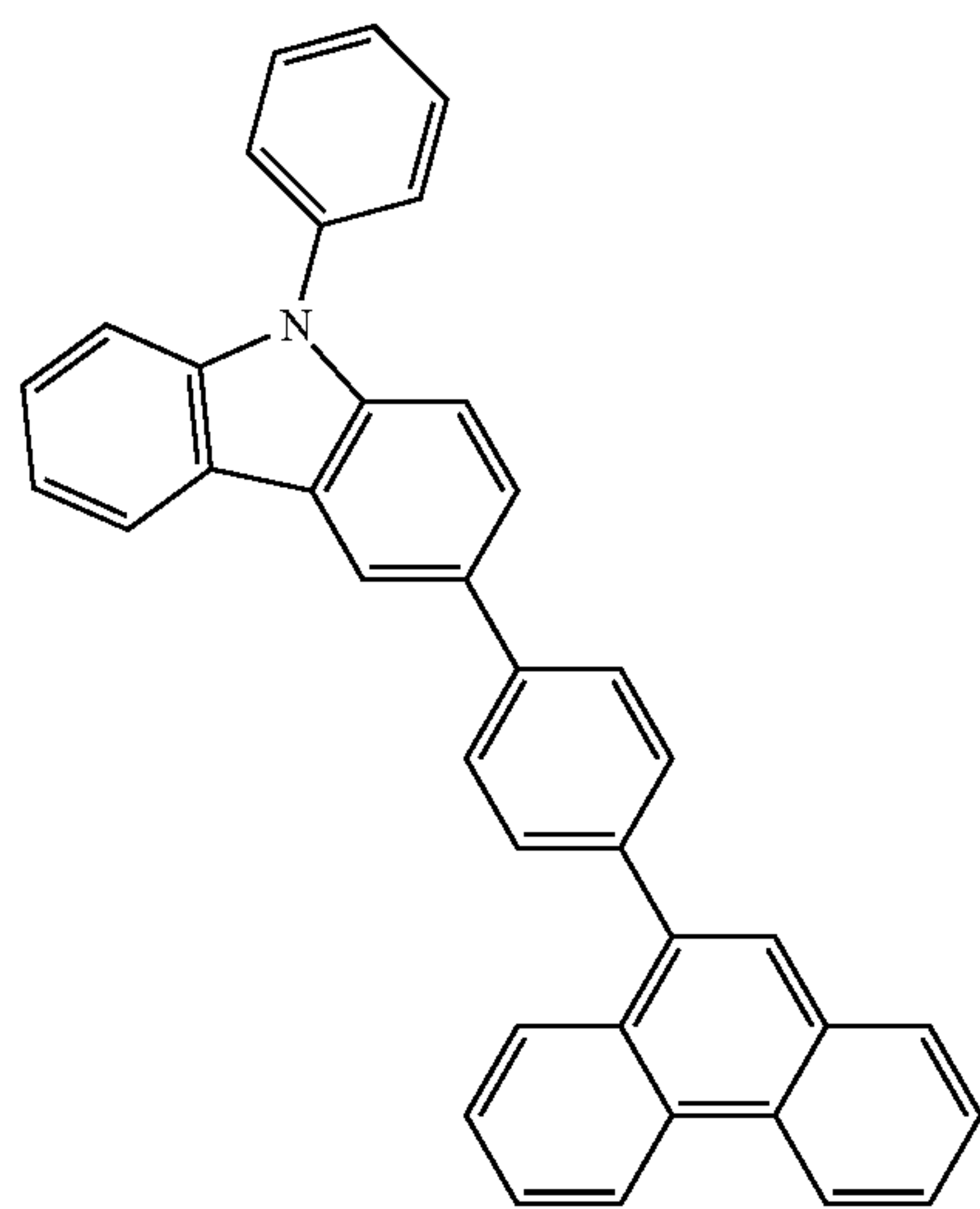
PCPPn
