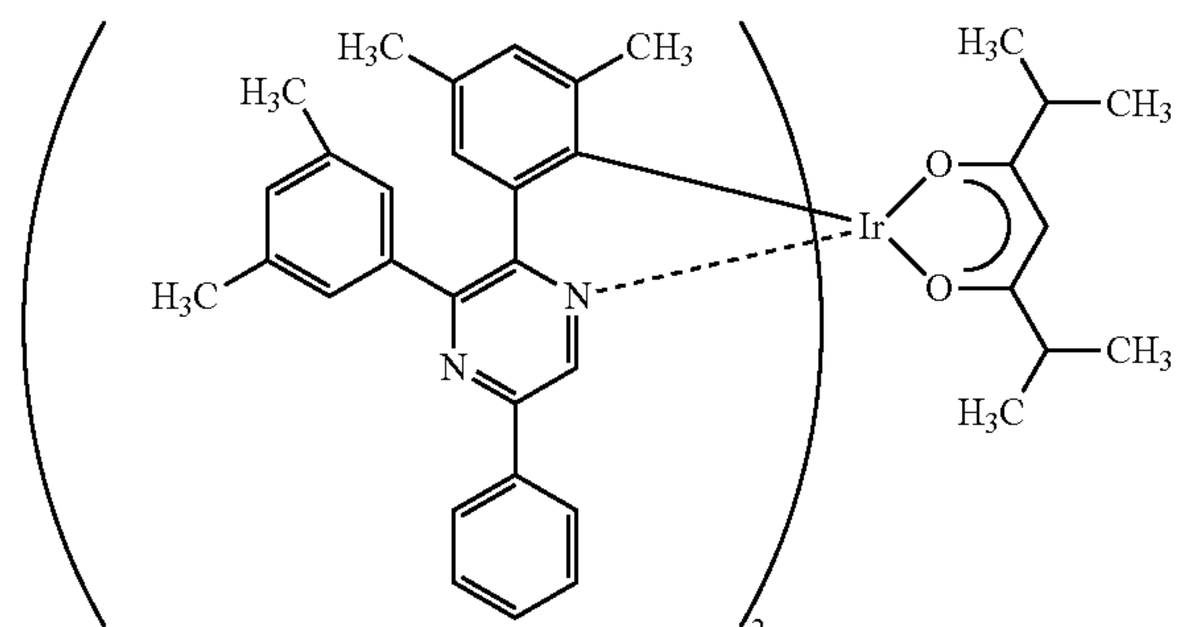
Ir(dmdppr-P) 2 (dibm)
