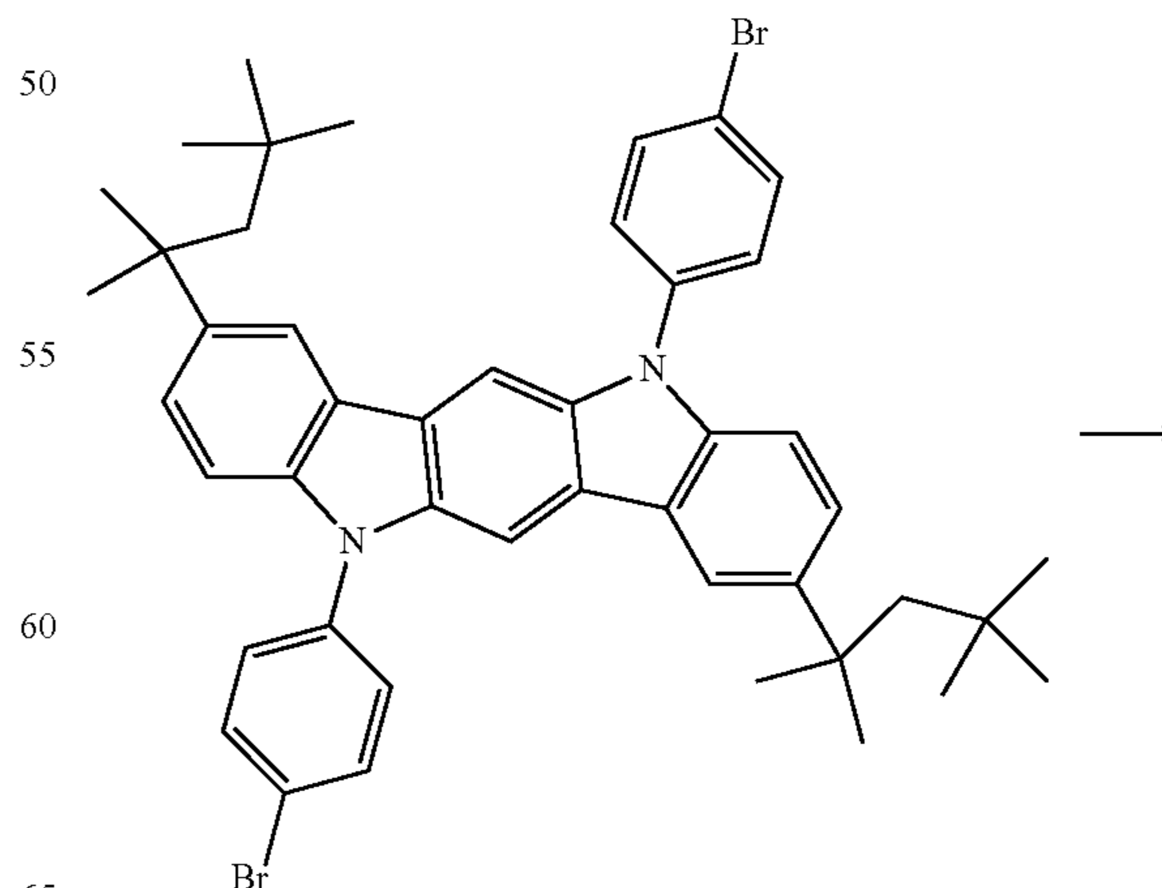
Monomer A
