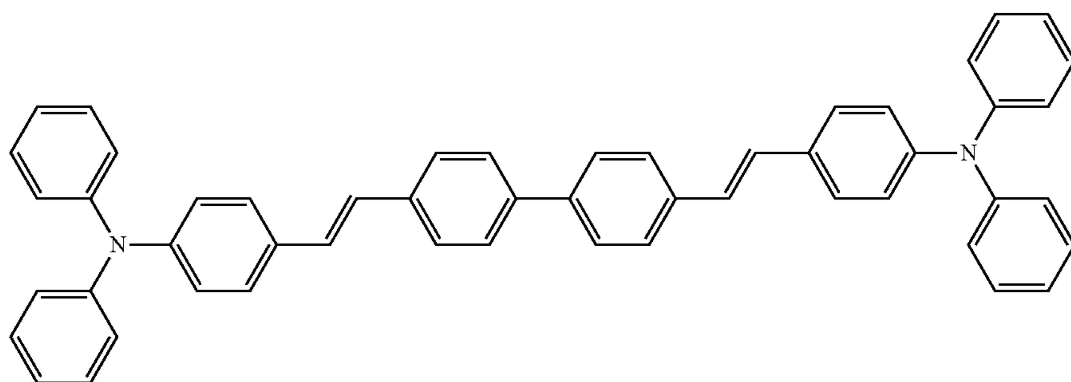
BDAVBi
