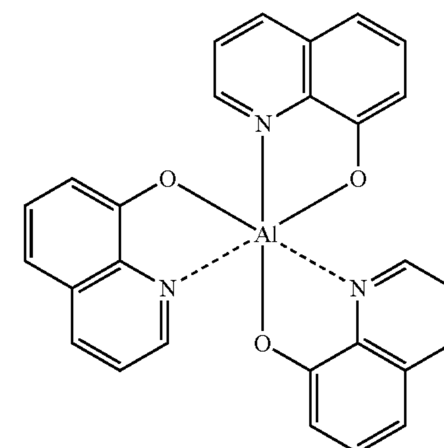
Alq 3
