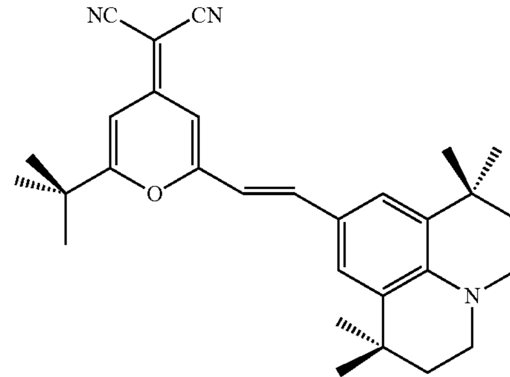
DCJTb
