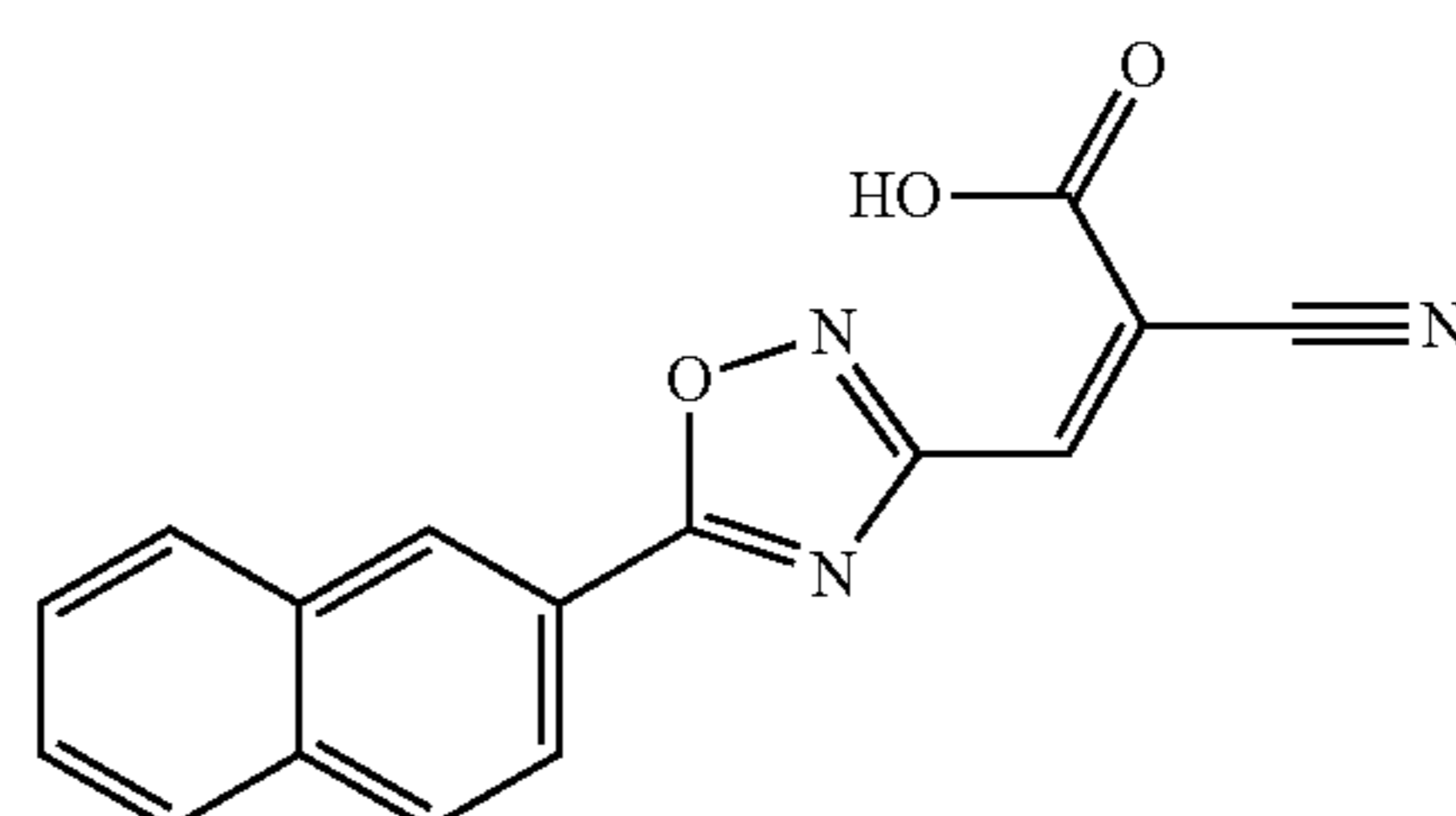
(Z)-2-cyano-3-(5-(naphthalen-2-yl)-1,2,4-oxadiazol-3-yl)acrylic acid
