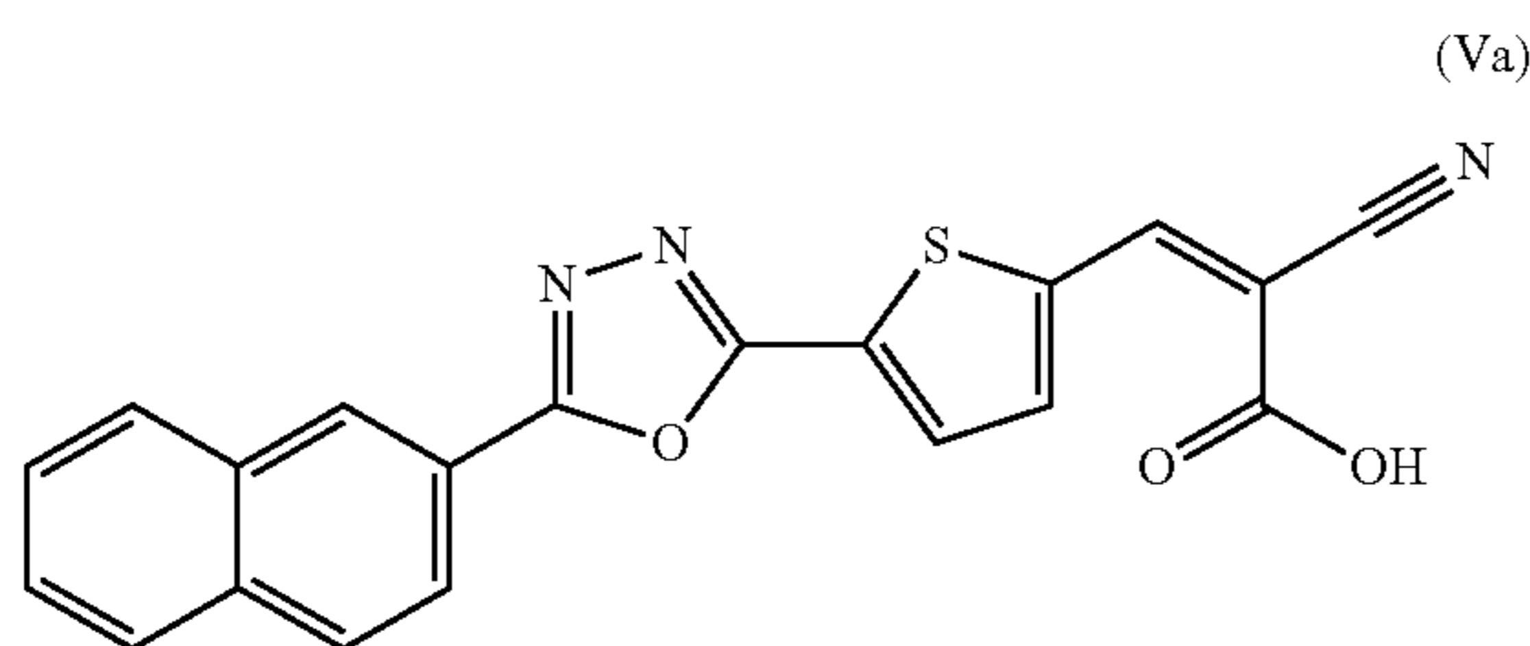
(Z)-2-cyano-3-(5-(5-(naphthalen-2-yl)-1,3,4-oxadiazol-2-yl)thiophen-2-yl)acrylic acid
