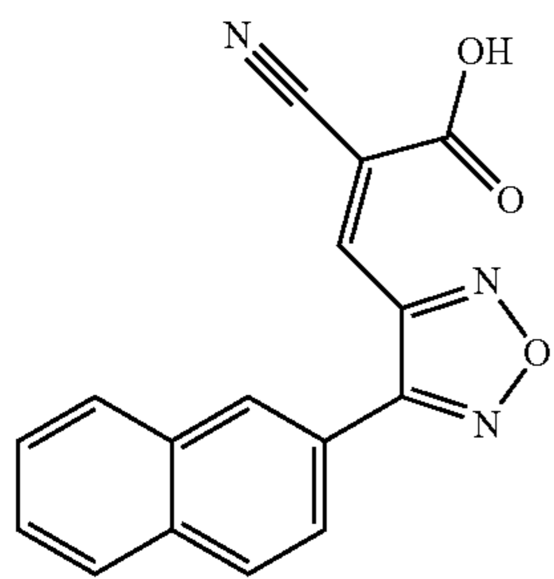
(Z)-2-cyano-3-(4-(naphthalen-2-yl)-1,2,5-oxadiazol-3-yl)acrylic acid
