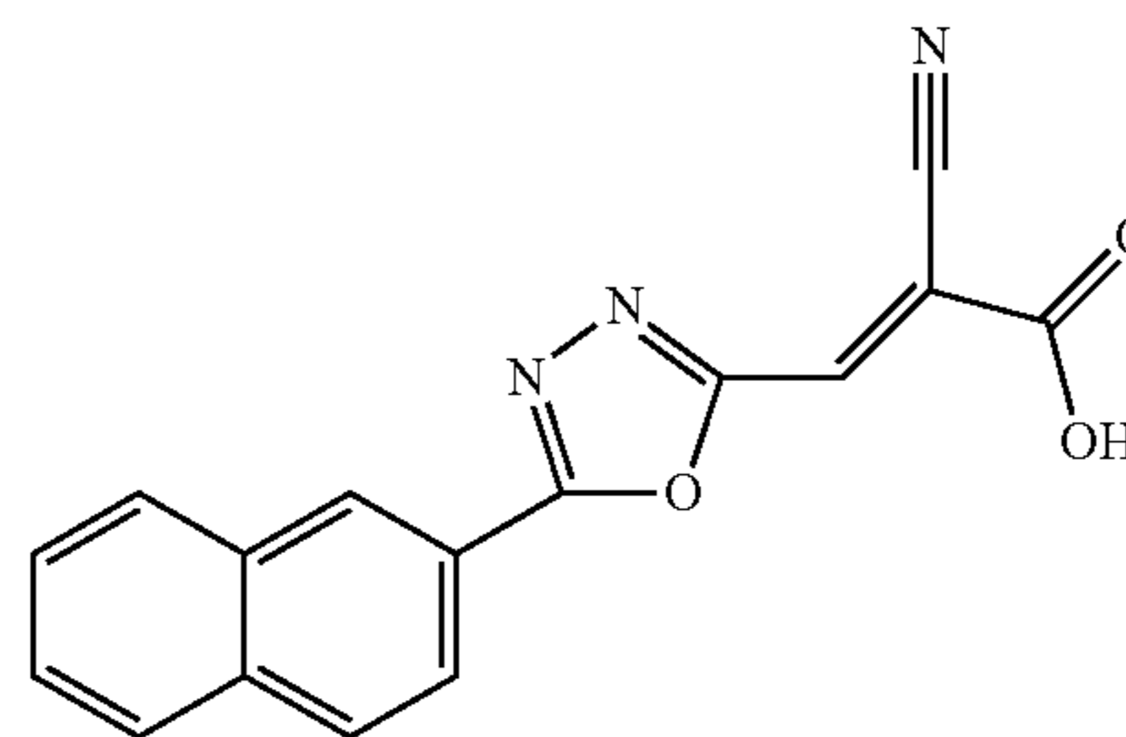
(E)-2-cyano-3-(5-(naphthalen-2-yl)-1,3,4-oxadiazol-2-yl)acrylic acid
