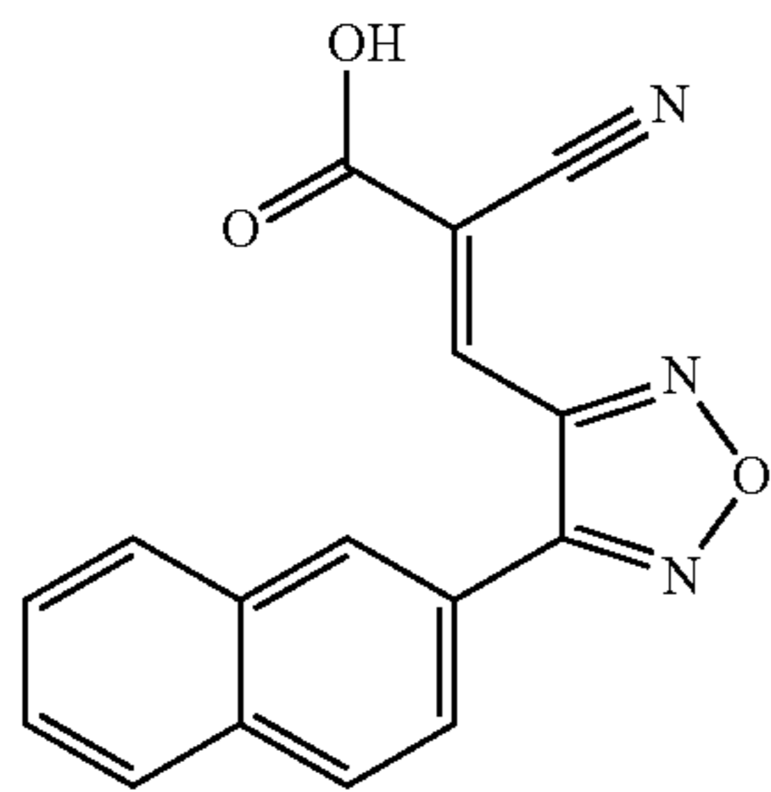
(E)-2-cyano-3-(4-(naphthalen-2-yl)-1,2,5-oxadiazol-3-yl)acrylic acid
