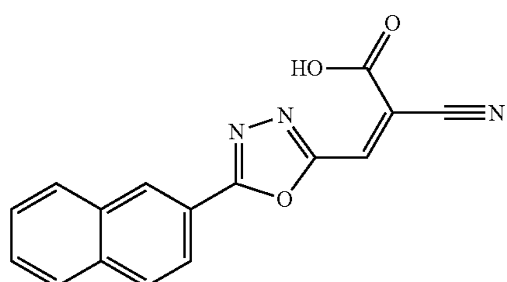
(Z)-2-cyano-3-(5-(naphthalen-2-yl)-1,3,4-oxadiazol-2-yl)acrylic acid
