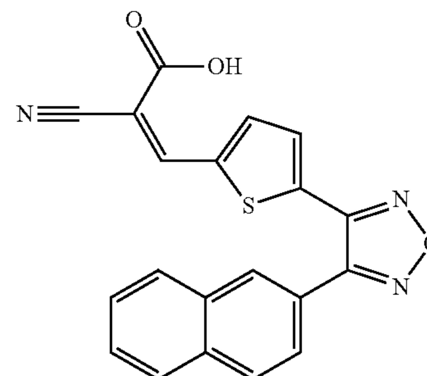
(Z)-2-cyano-3-(5-(4-(naphthalen-2-yl)-1,2,5-oxadiazol-3-yl)thiophen-2-yl)acrylic acid
