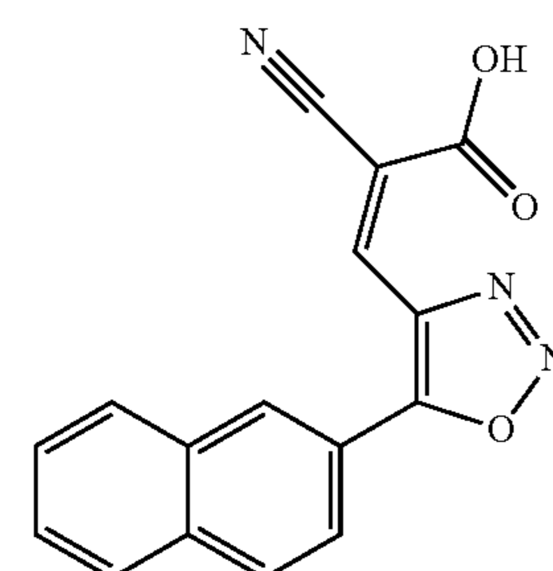
(Z)-2-cyano-3-(5-(naphthalen-2-yl)-1,2,3-oxadiazol-4-yl)acrylic acid
