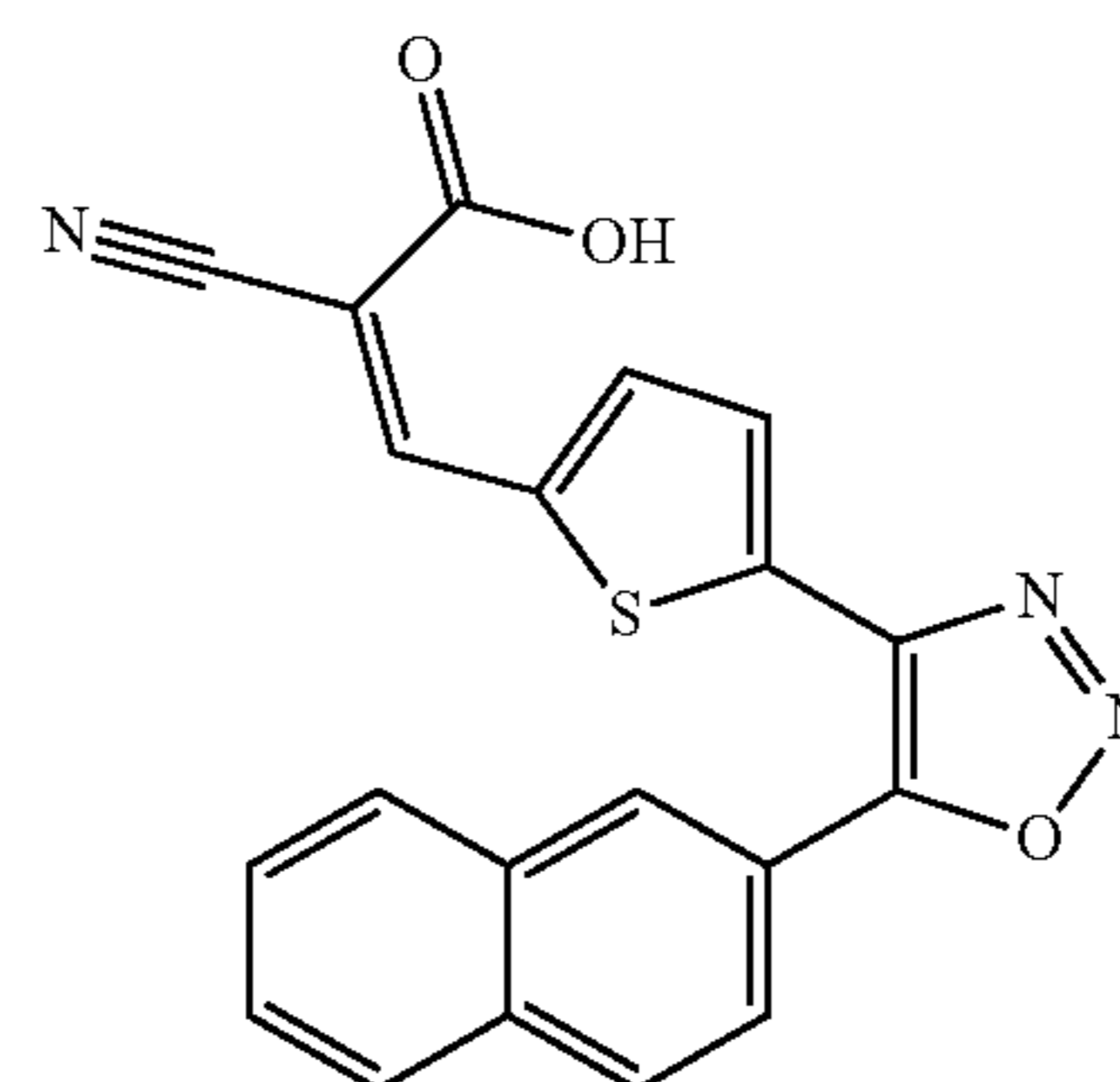
(Z)-2-cyano-3-(5-(5-(naphthalen-2-yl)-1,2,3-oxadiazol-4-yl)thiophen-2-yl)acrylic acid
