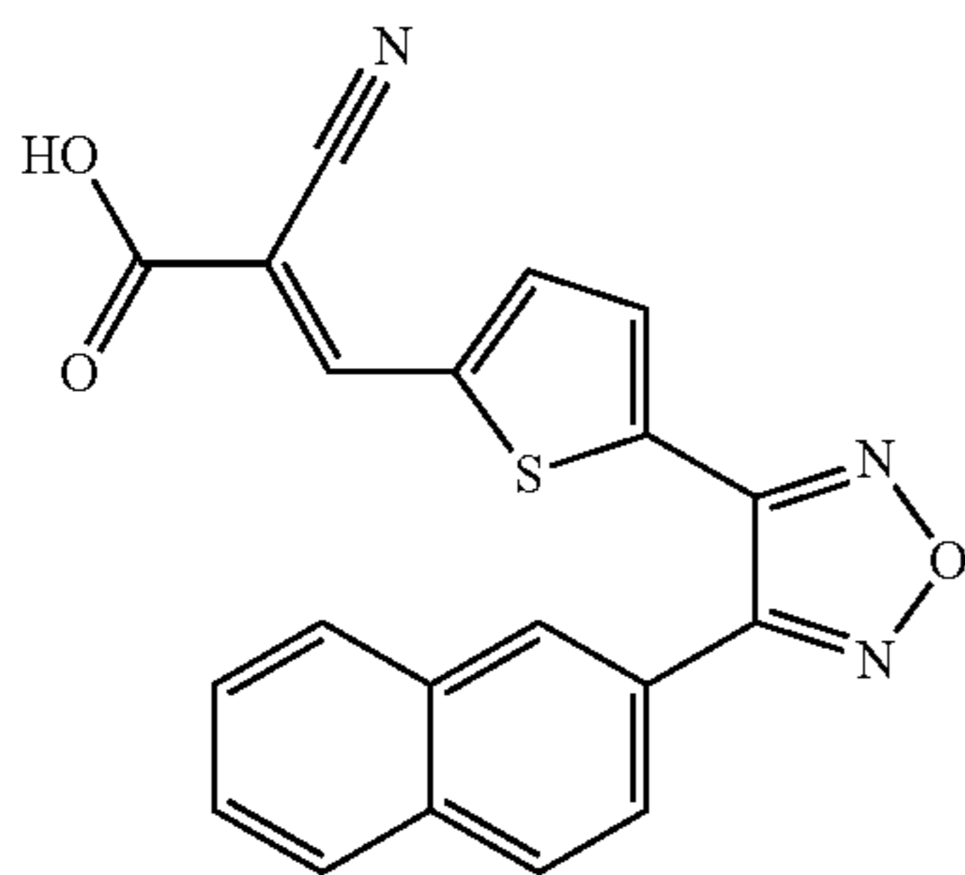
(E)-2-cyano-3-(5-(4-(naphthalen-2-yl)-1,2,5-oxadiazol-3-yl)thiophen-2-yl)acrylic acid
