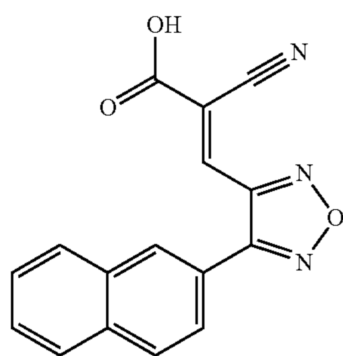
(E)-2-cyano-3-(4-(naphthalen-2-yl)-1,2,5-oxadiazol-3-yl)acrylic acid
