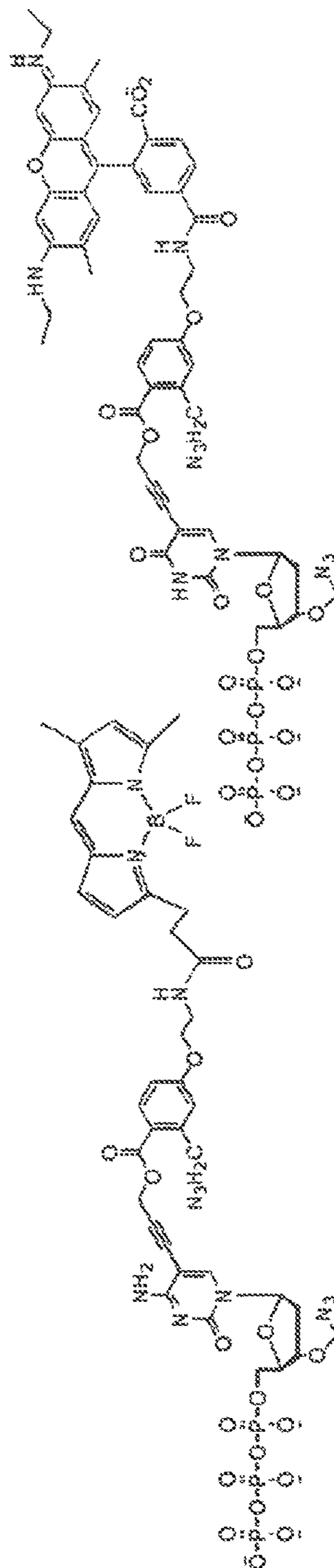
3'-O-Azido-dUTP-Azido-R6G
