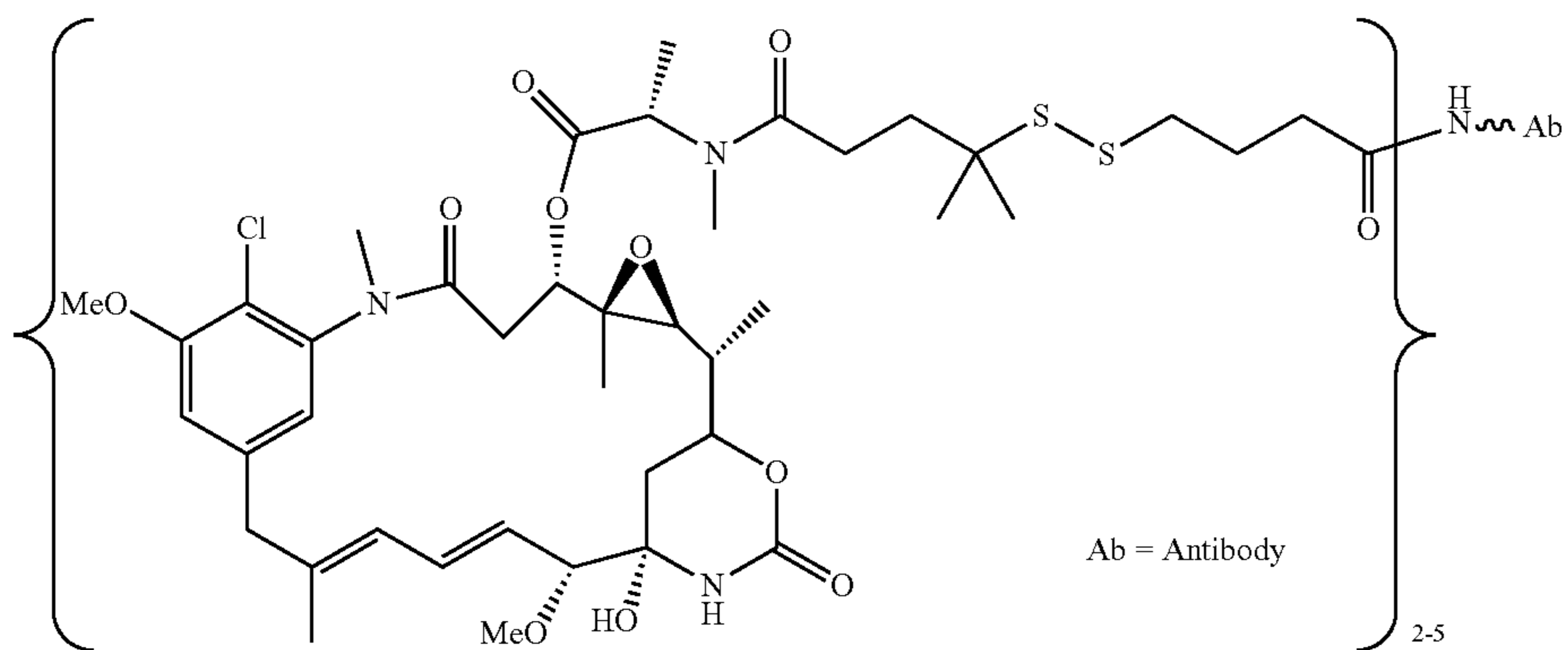
Ab-SPDB-DM4
