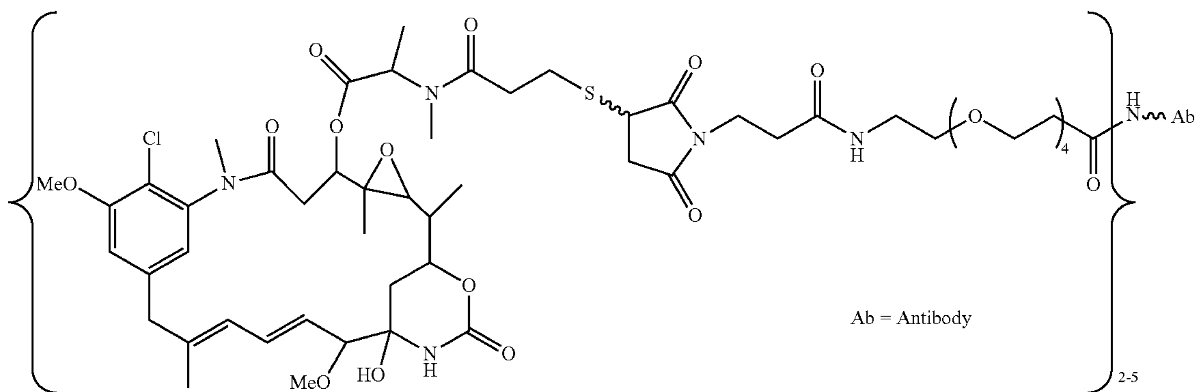
Ab-PEG4-Mal-DM1
