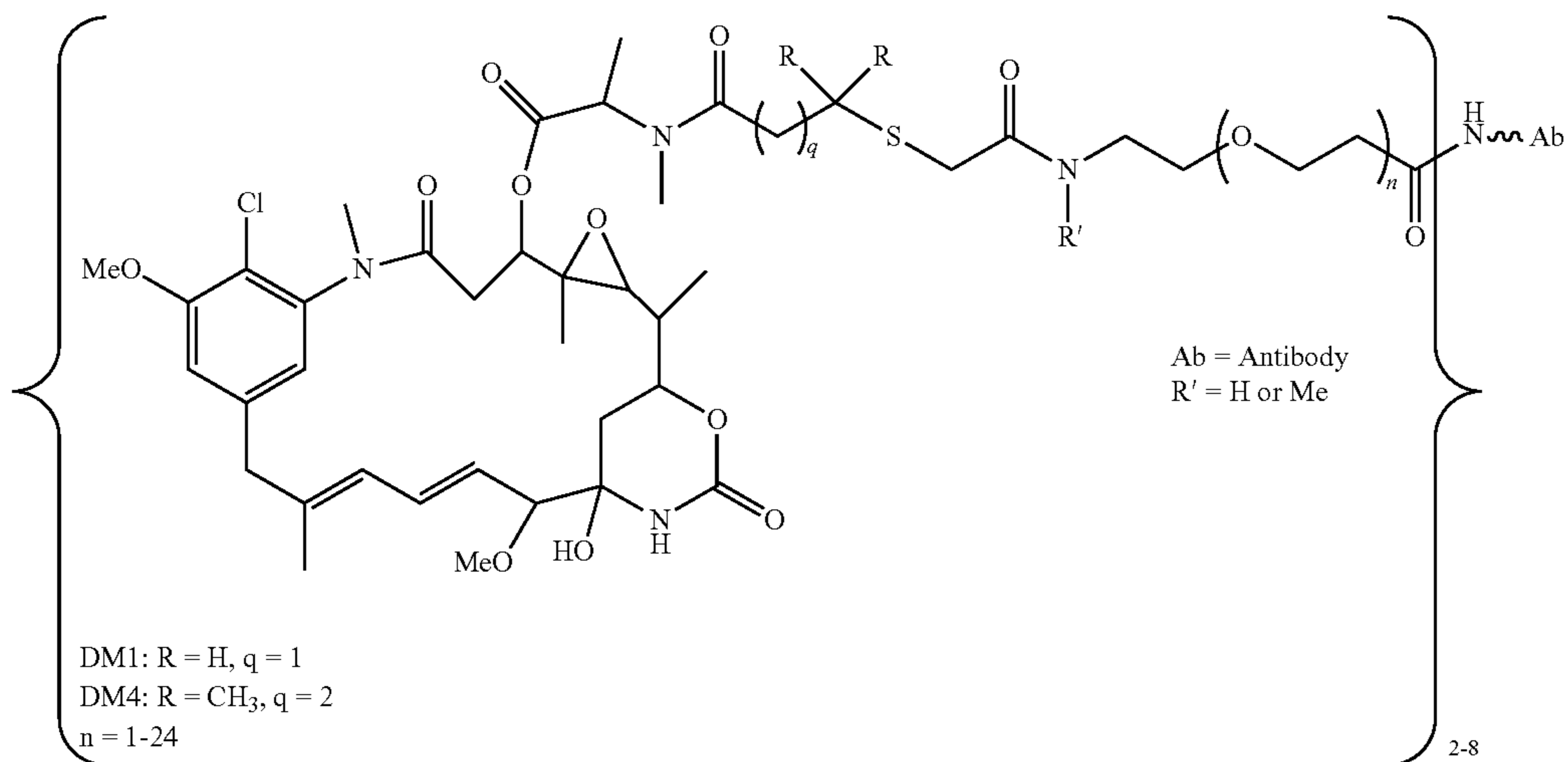
Ab-PEG-SIA-DM1/DM4
