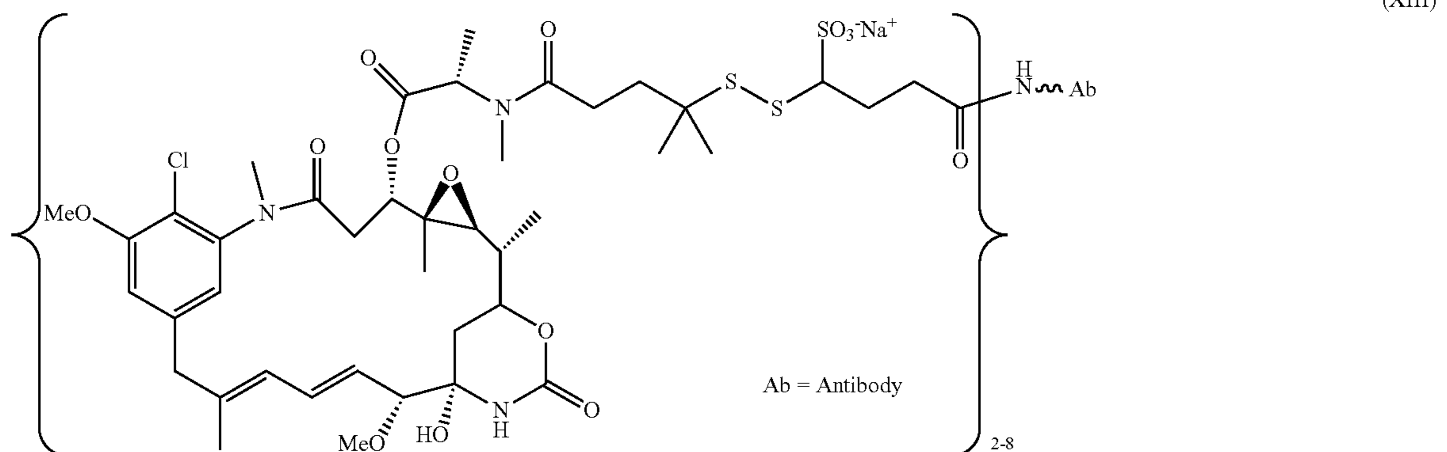
Ab-sulfo-SPDB-DM4
