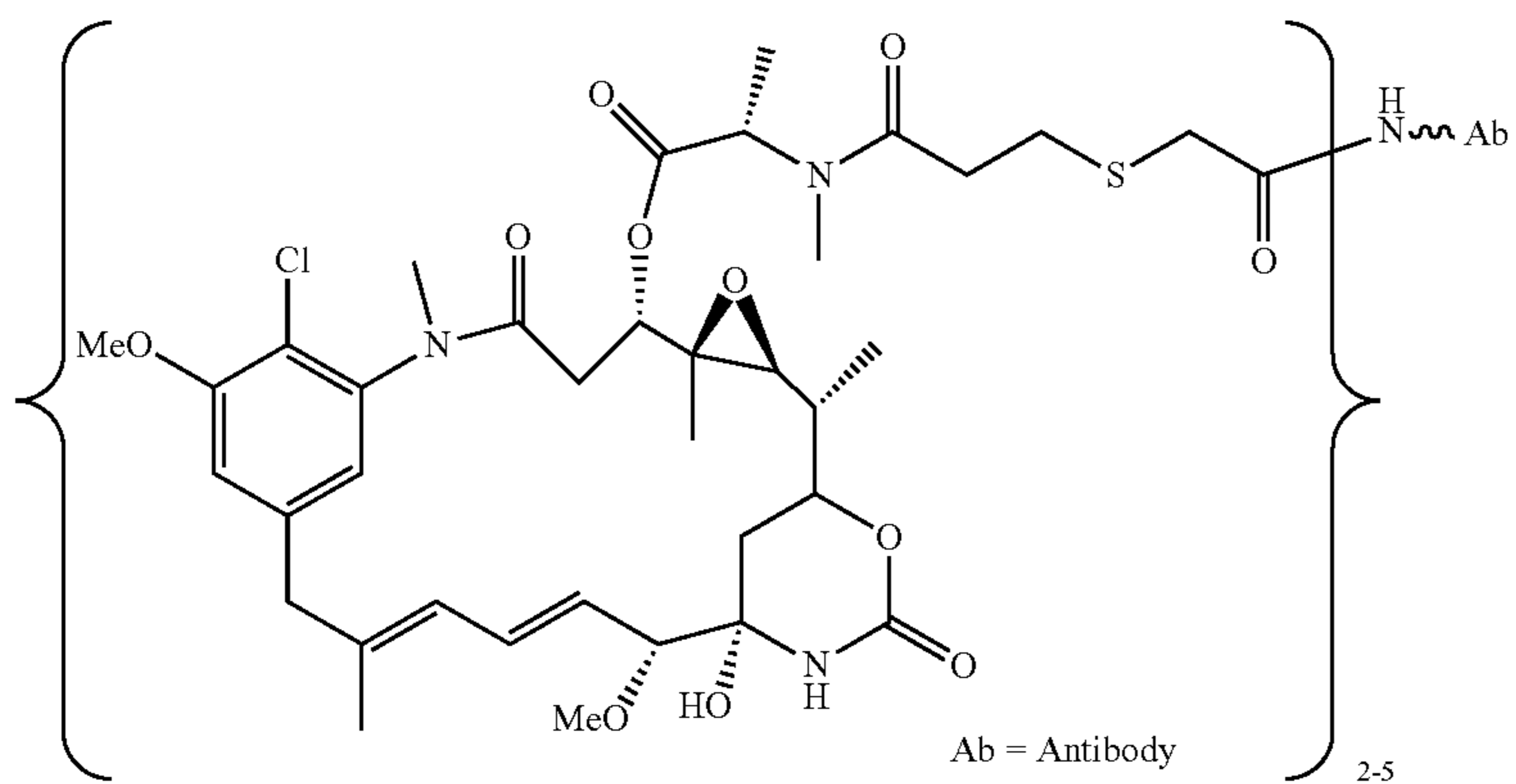
Ab-SIA-DM1
