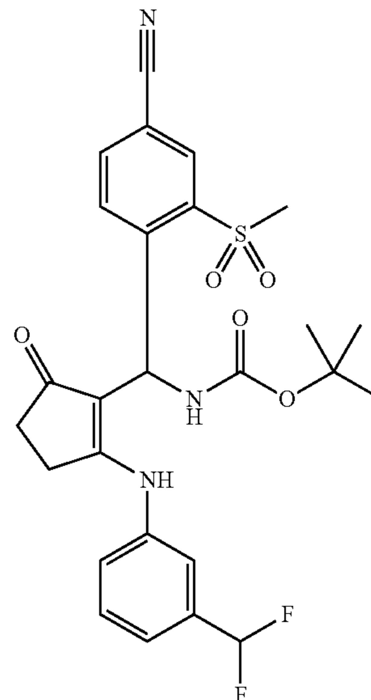
tert-Butyl(4-Cyano-2-(methylsulfonyl)phenyl)(2-(3-(difluoromethyl)phenylamino)cyclopent-2-en-1-yl)methylcarbamate
