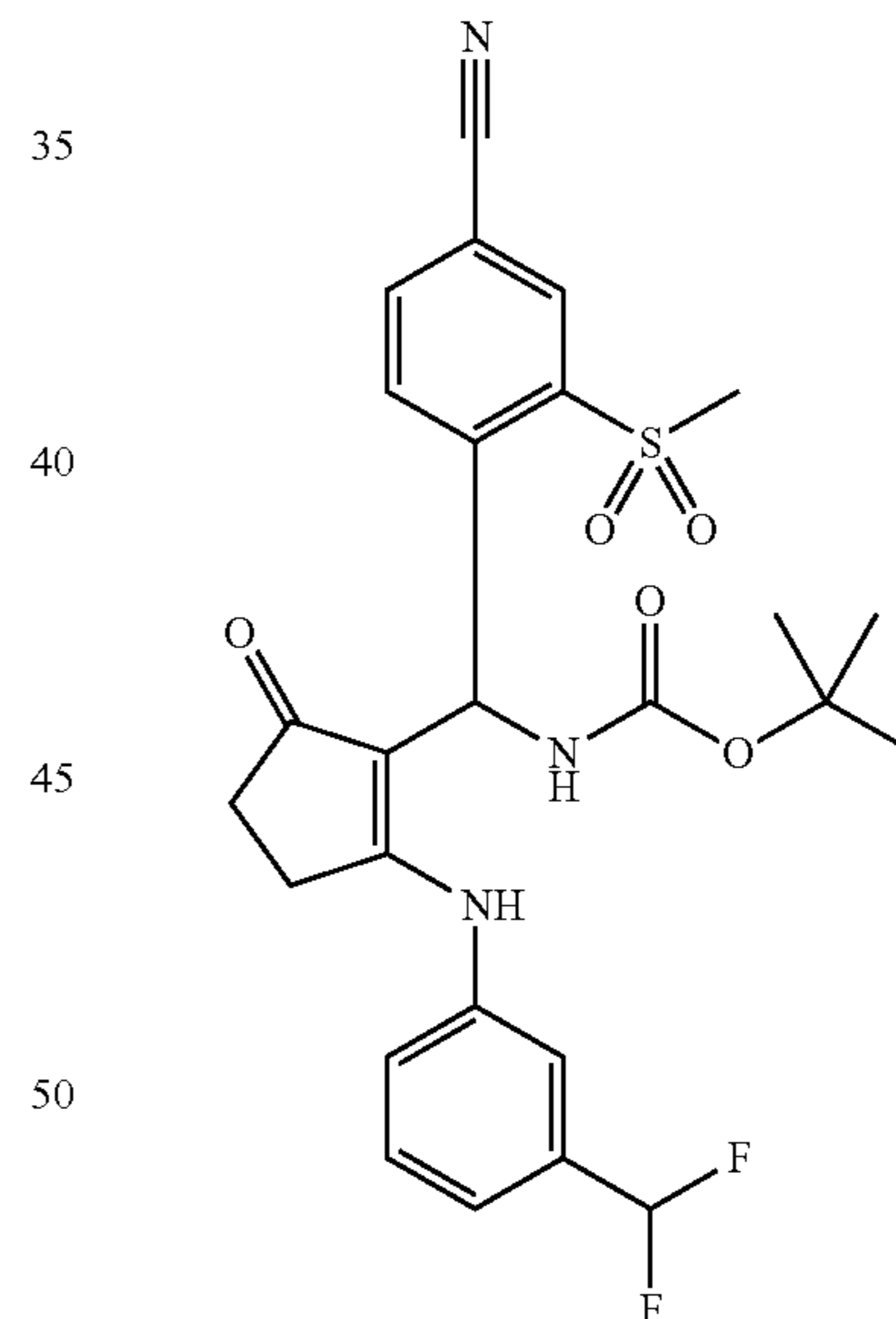
tert-Butyl(4-Cyano-2-(methylsulfonyl)phenyl)(2-(3-(difluoromethyl)phenylamino)cyclopent-2-en-1-yl)methylcarbamate
