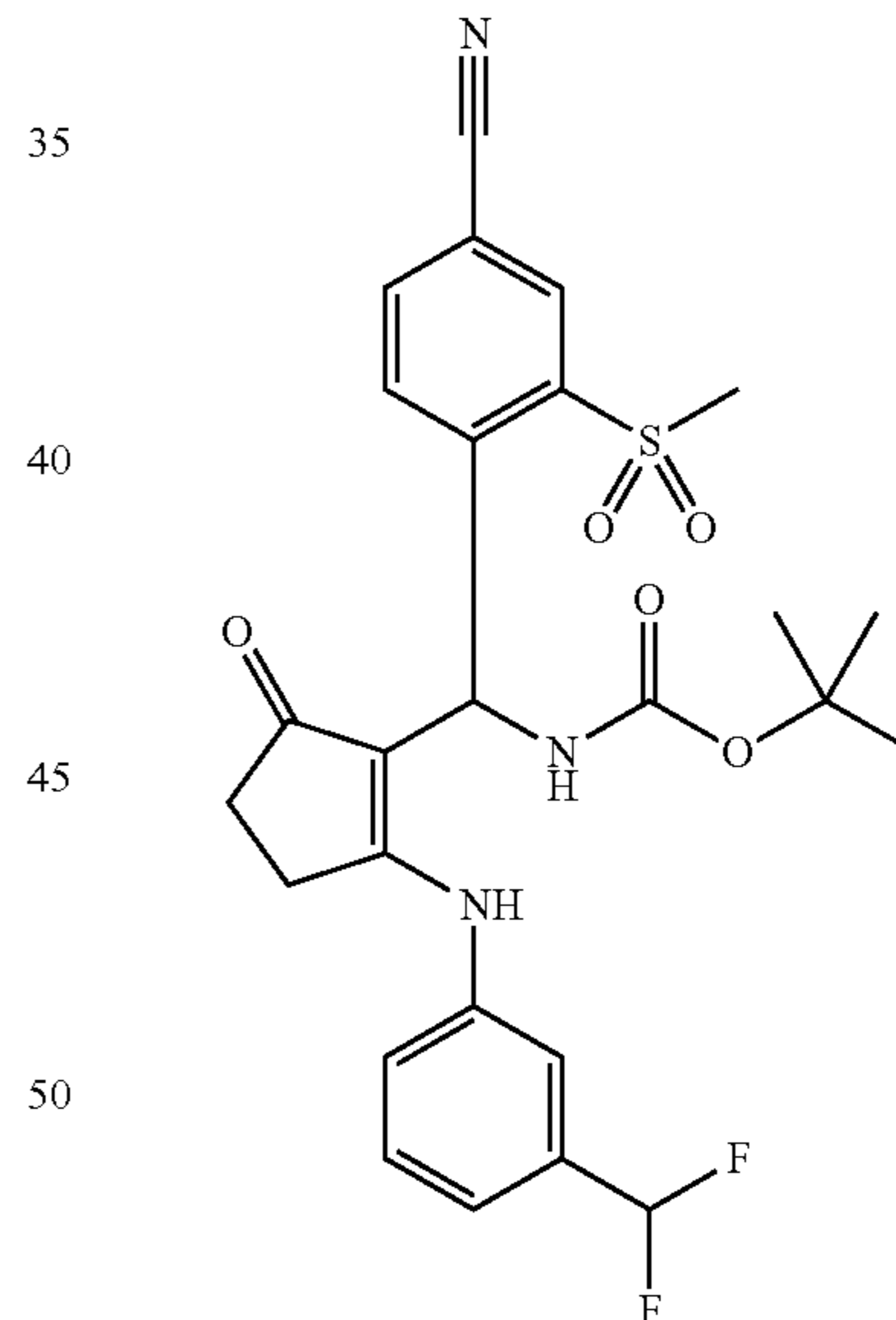
tert-Butyl(4-Cyano-2-(methylsulfonyl)phenyl)(2-(3-(difluoromethyl)phenylamino)cyclopent-2-en-1-yl)methylcarbamate
