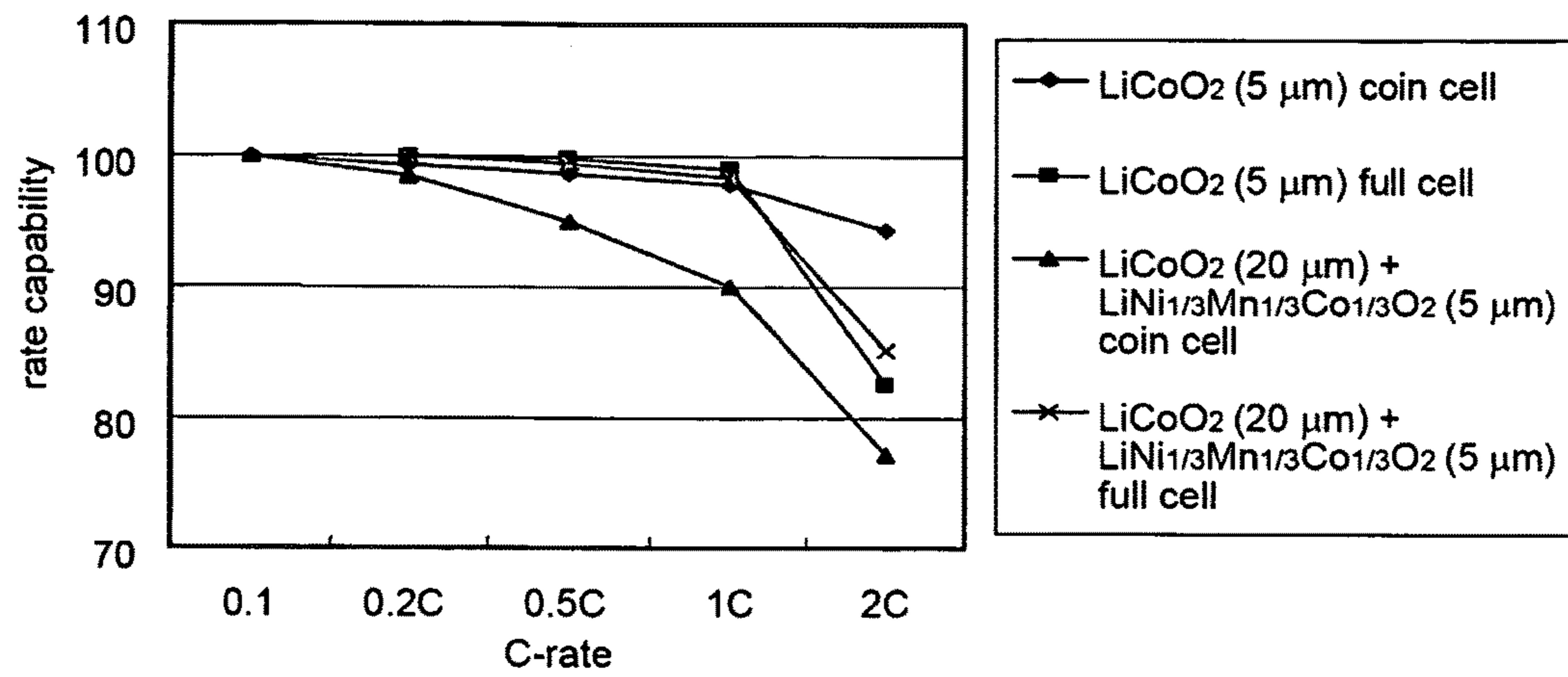
FIG. 12
