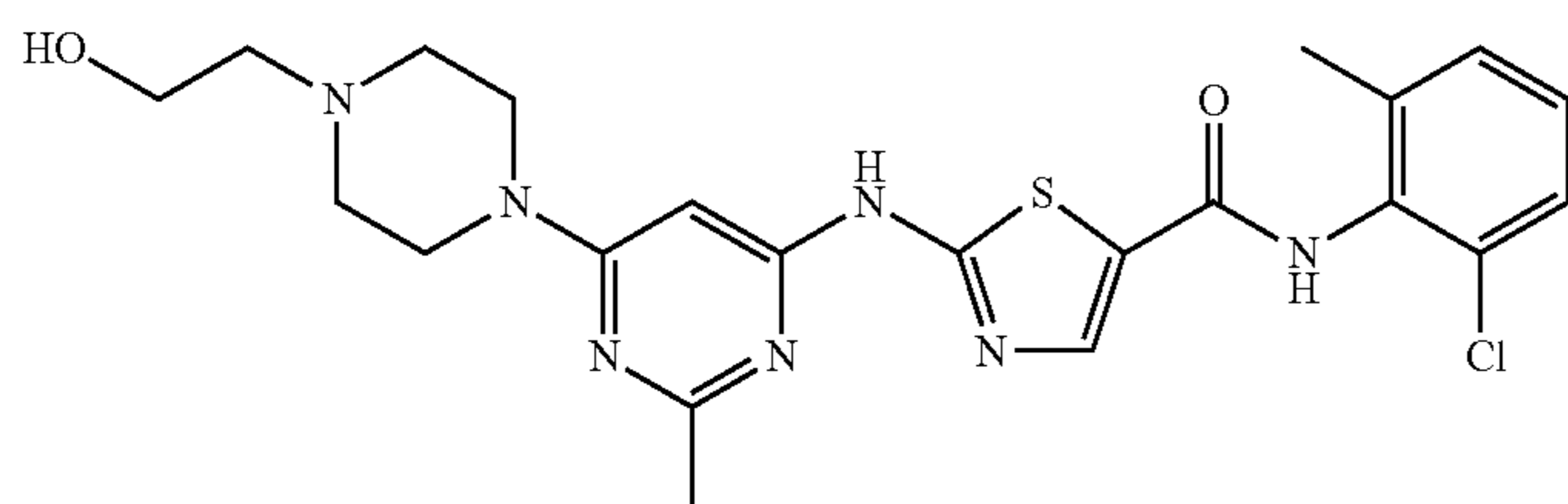
Dasatinib
