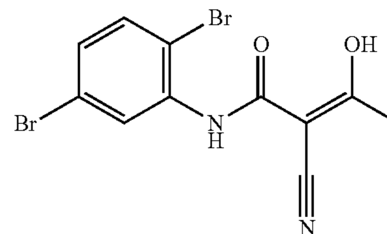
LFM-A13
