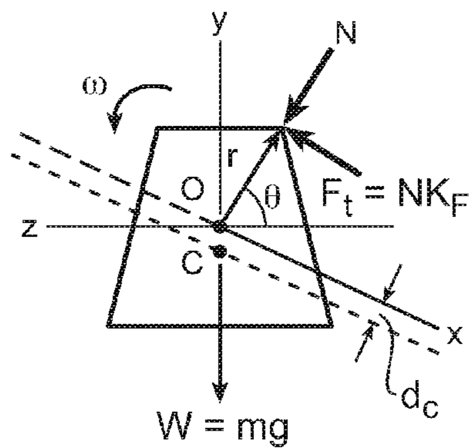
Free Body
