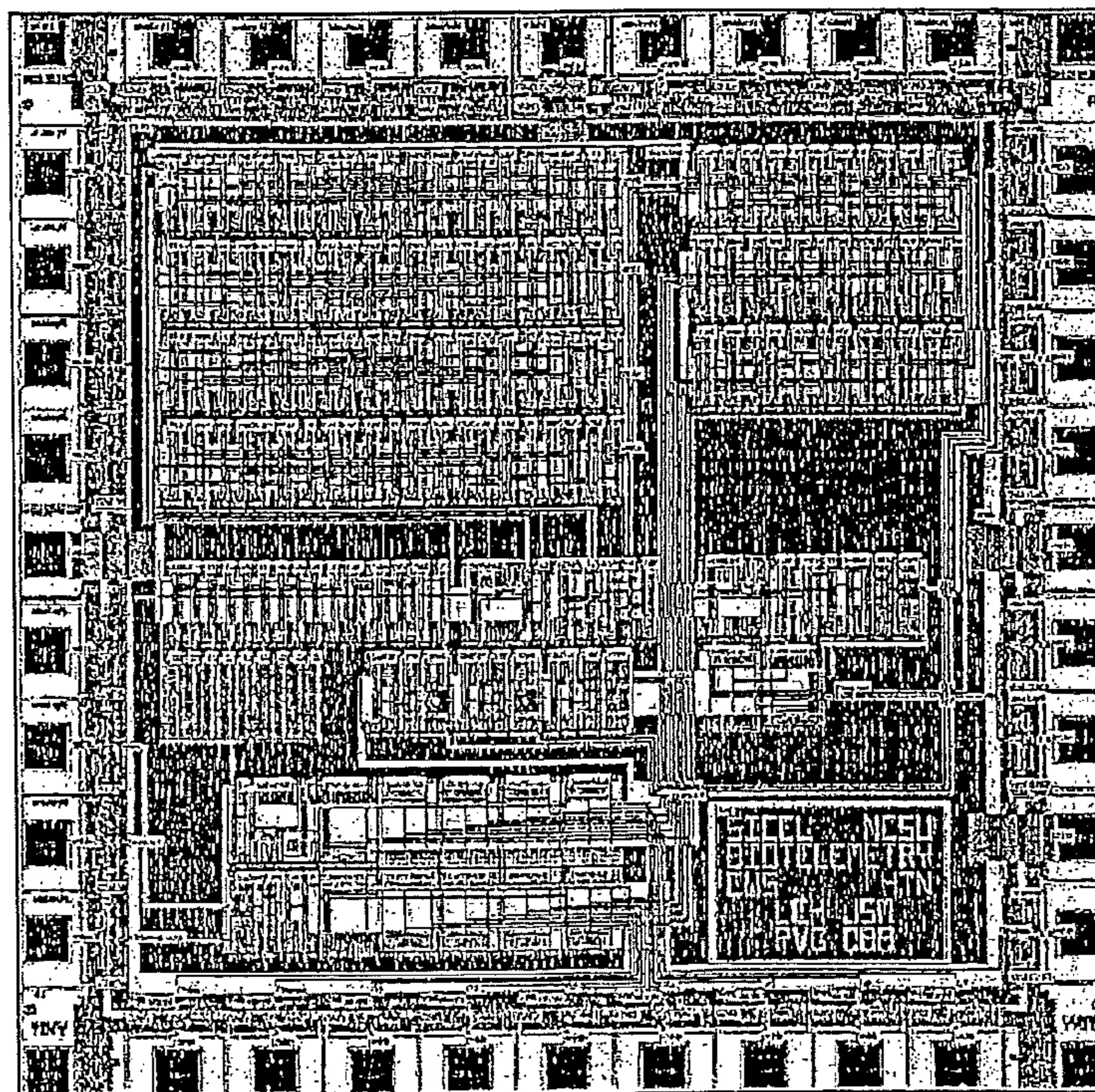
IC LAYOUT
