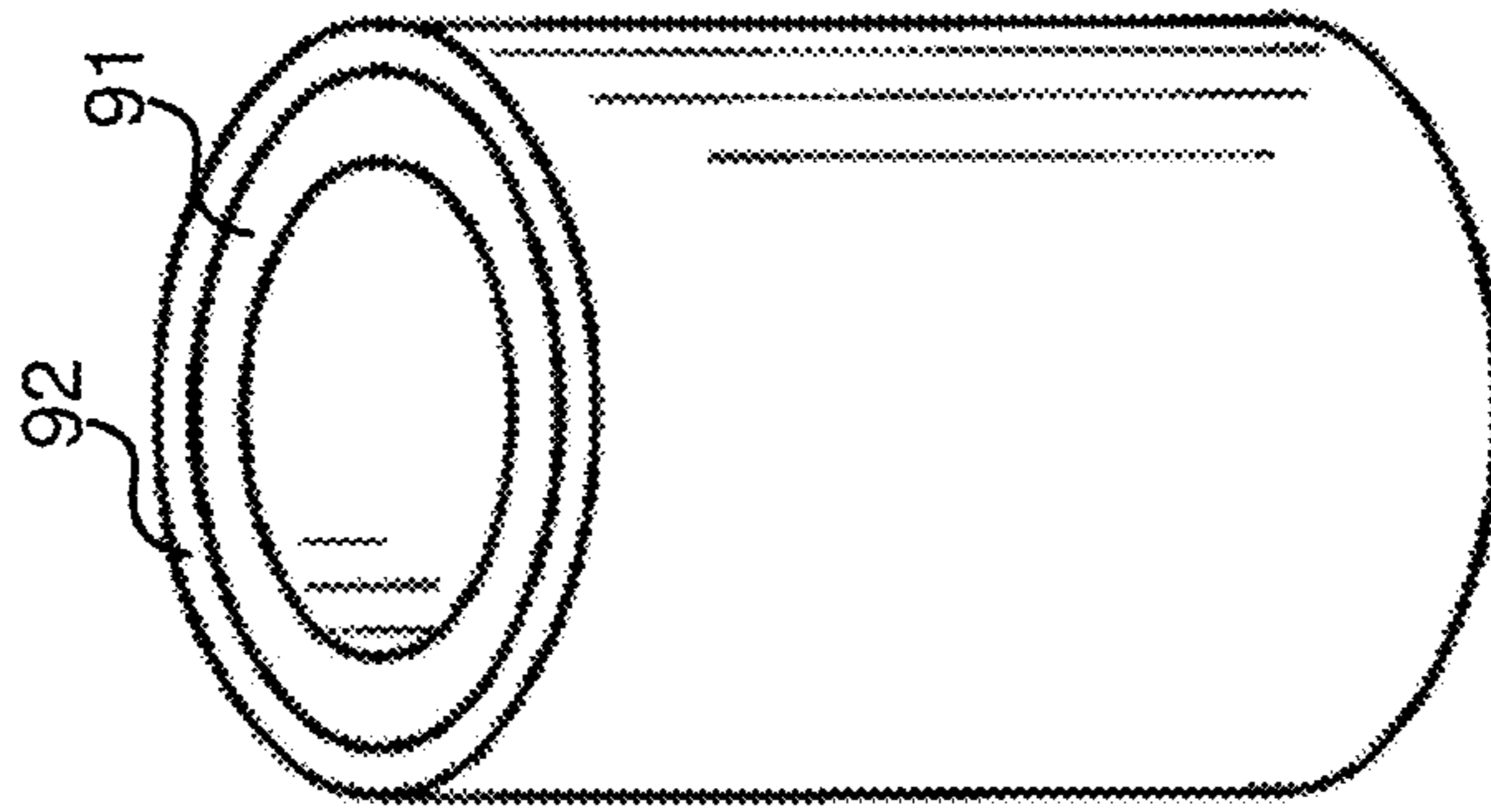
Fig. 15B
