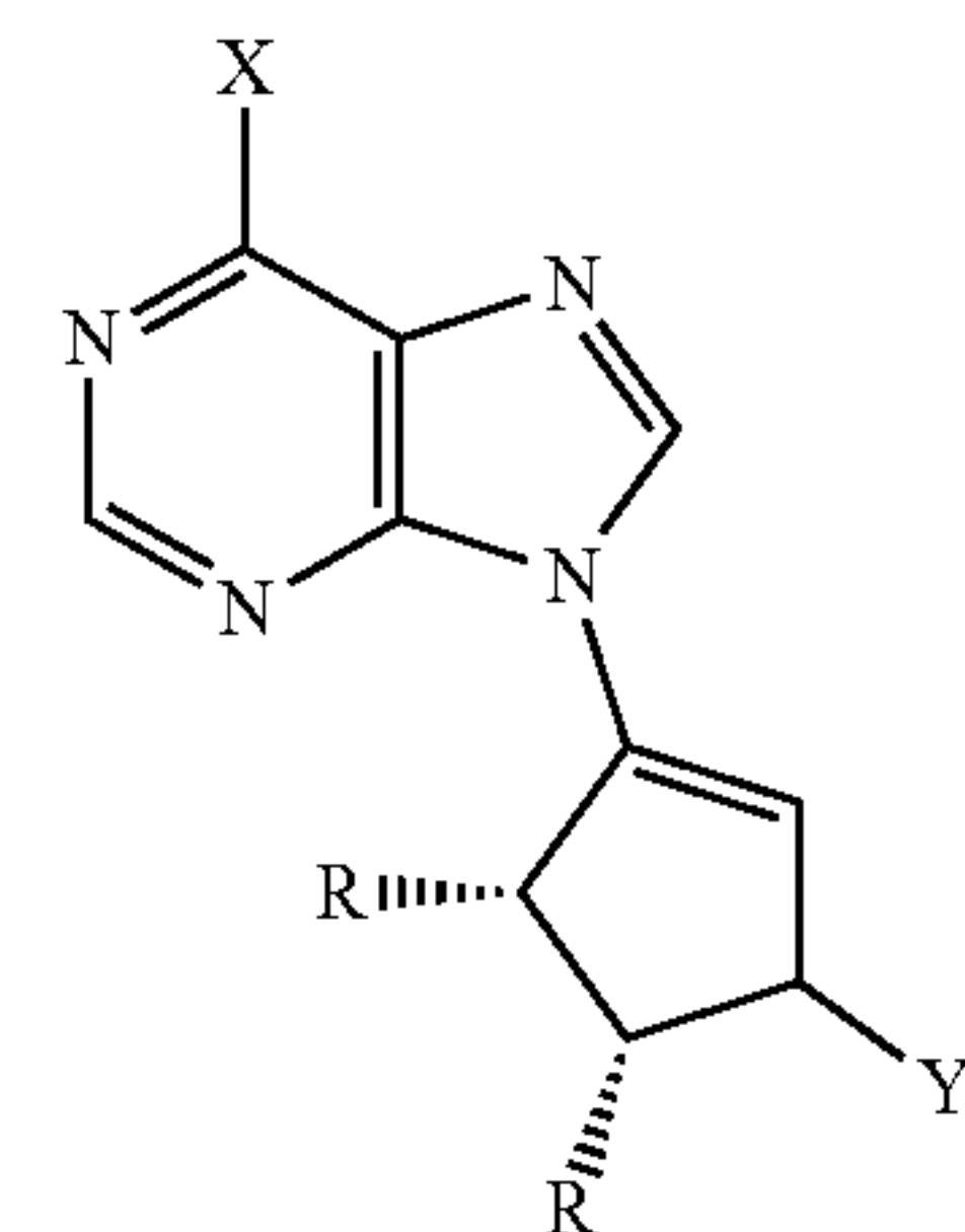
L-isoneplanocin analogue,
