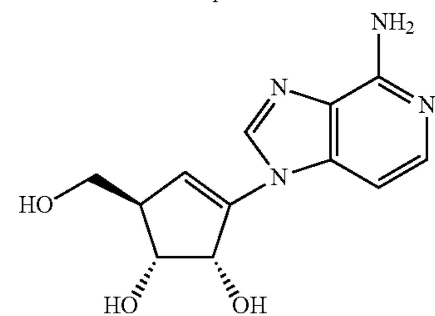
D-3-deazaisoneplanocin
