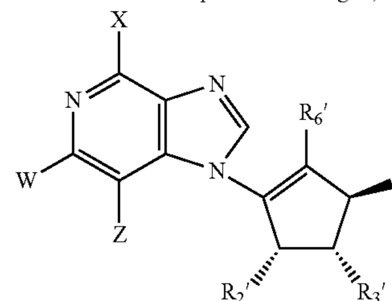
D-3-Deazaisoneplanocin analogue,
