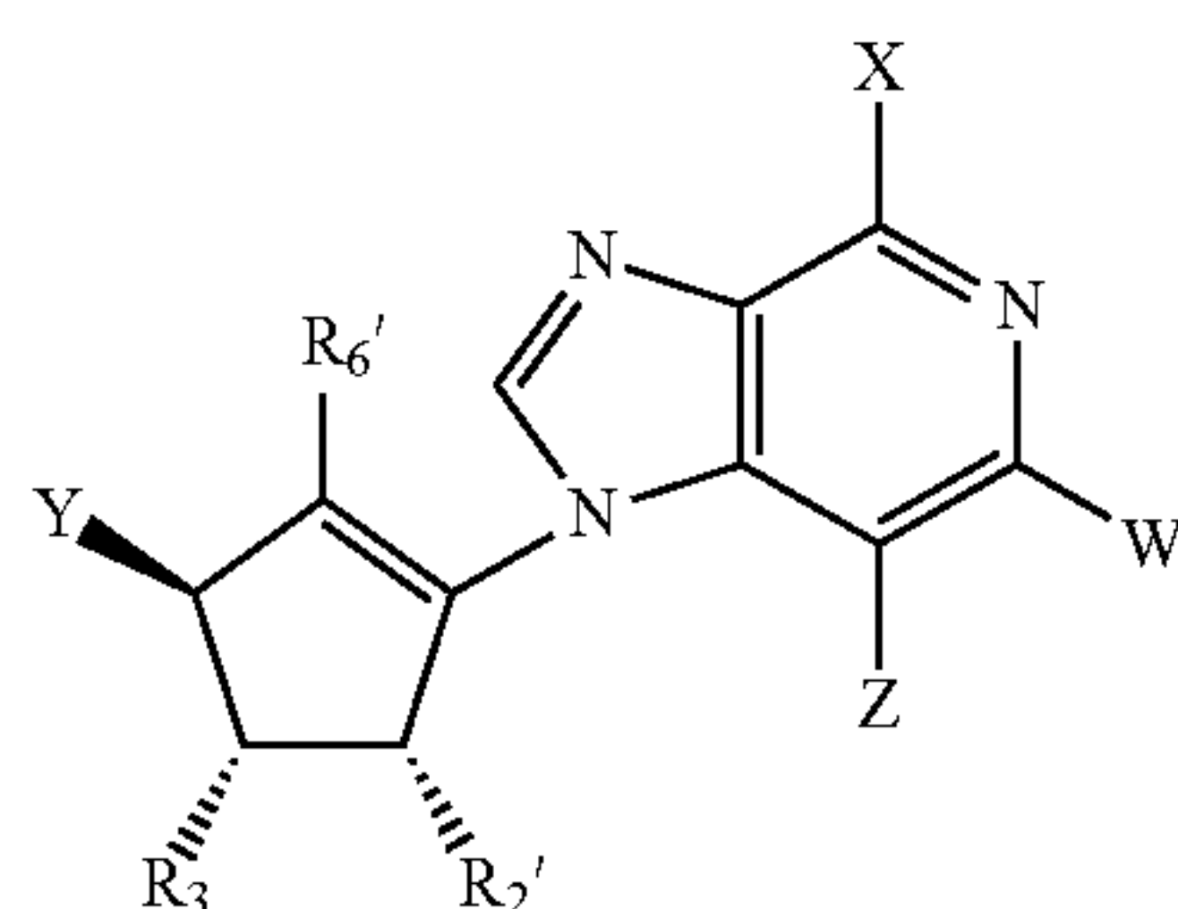
D-3-Deazaisoneplanocin analogue
