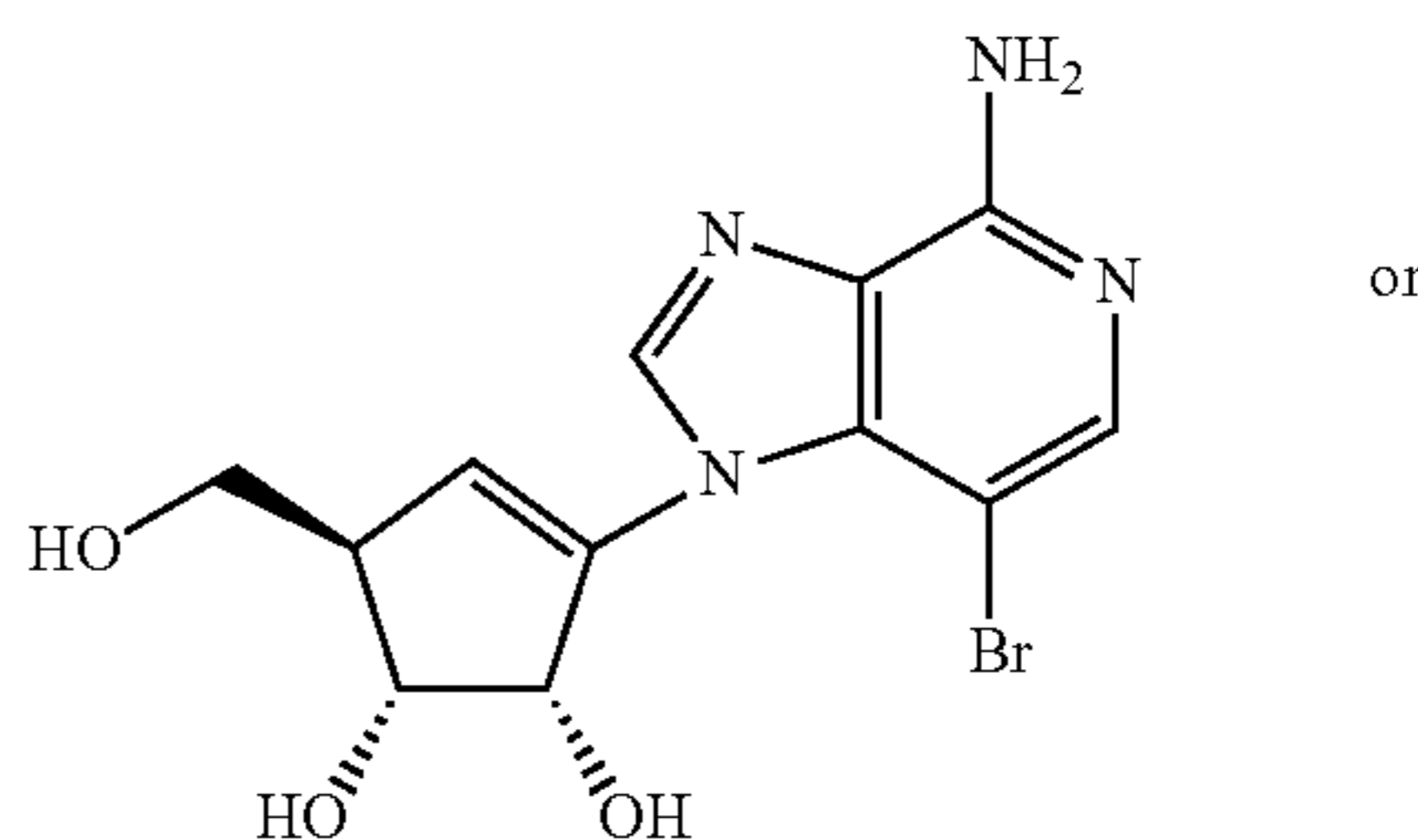
D-3-bromo-3-deazaisoneplanocin
