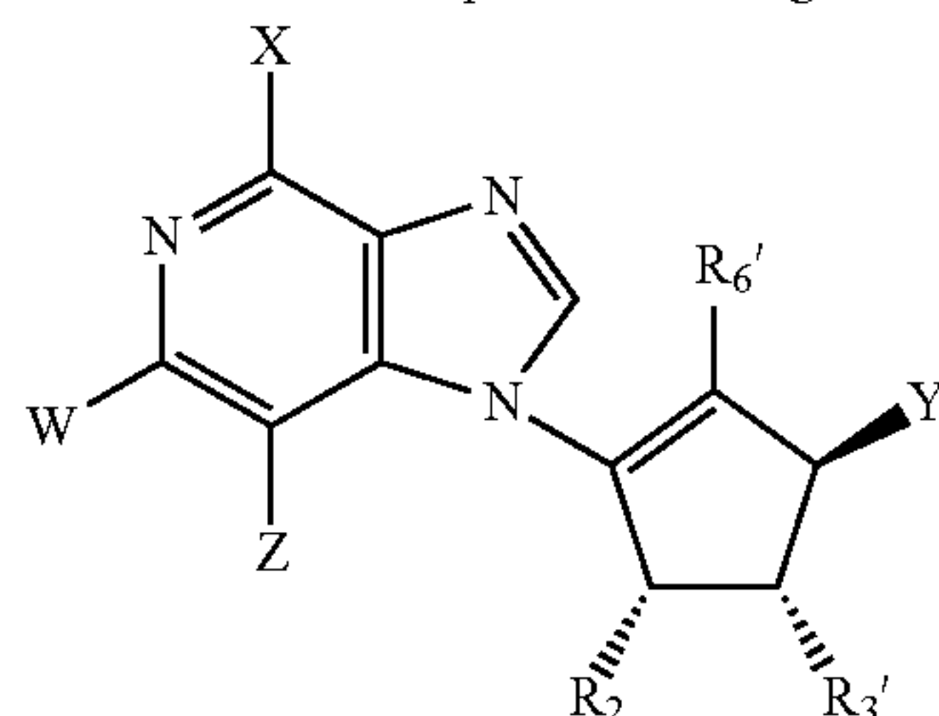
D-3-Deazaisoneplanocin analogue
