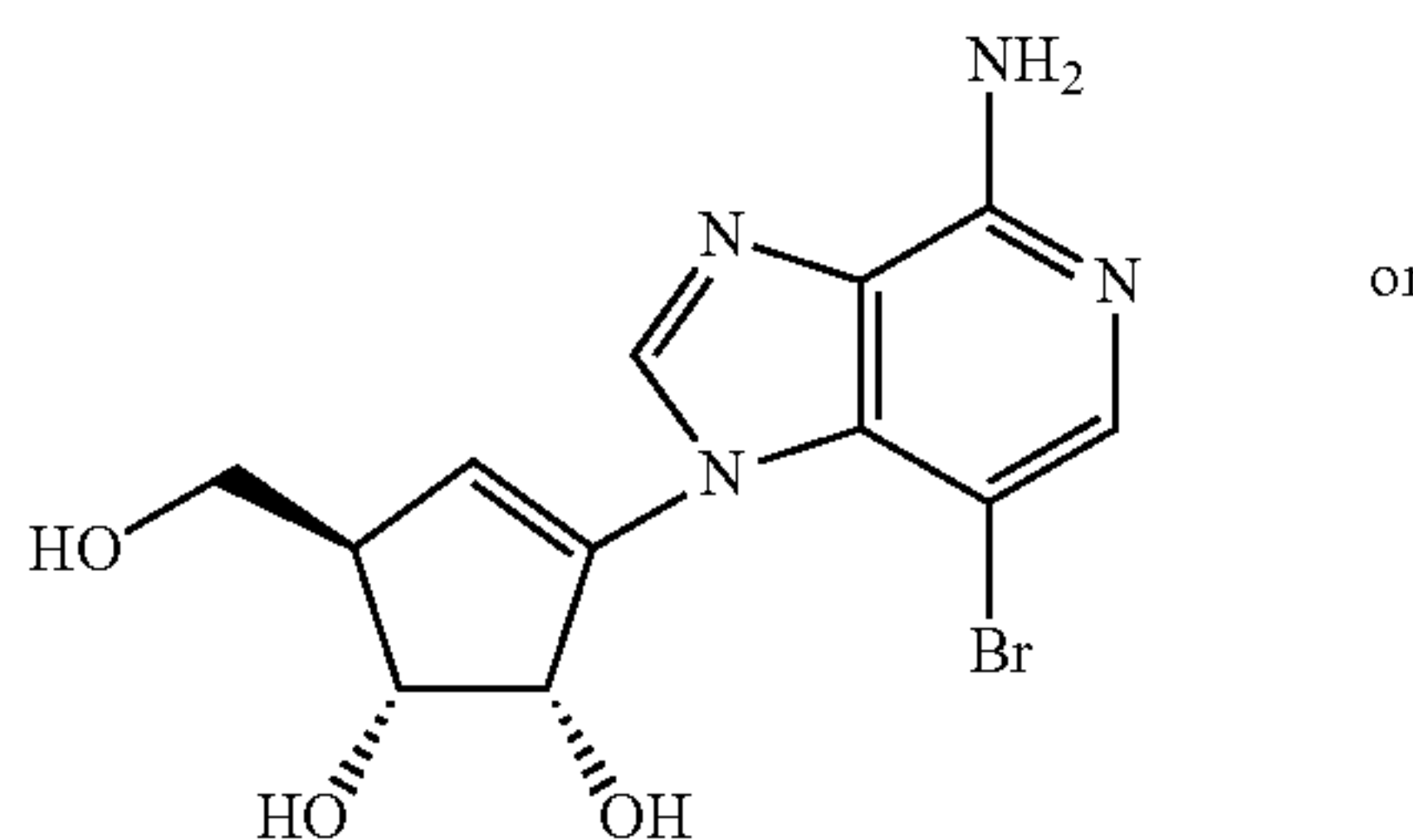
D-3-bromo-3-deazaisoneplanocin
