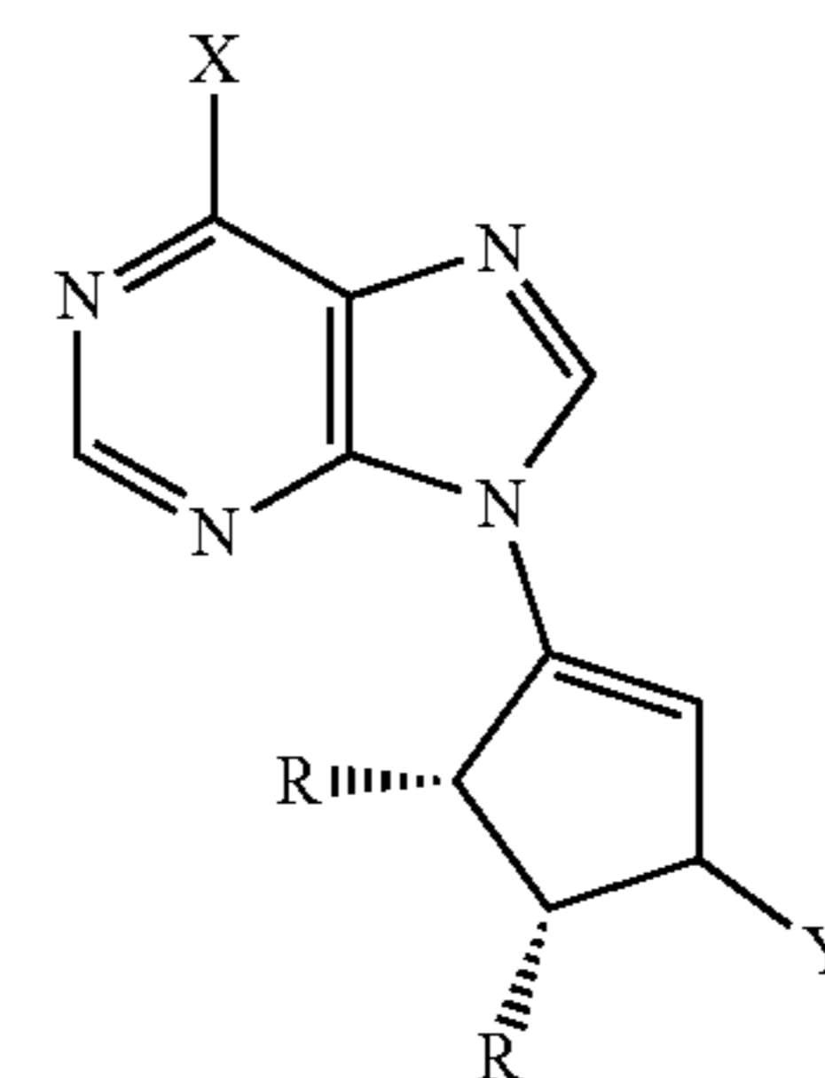
L-isoneplanocin analogue,
