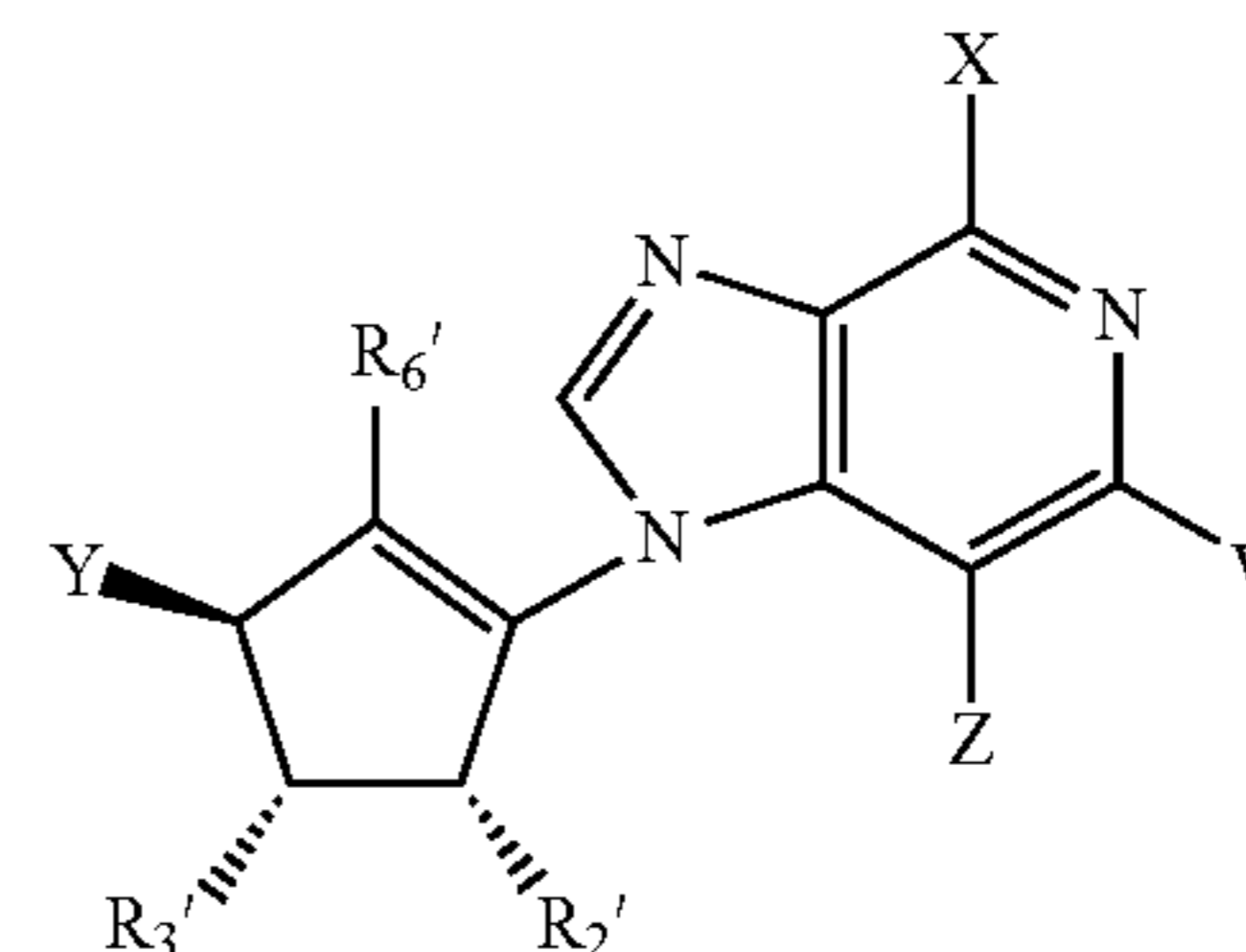
L-isoneplanocin analogue,
