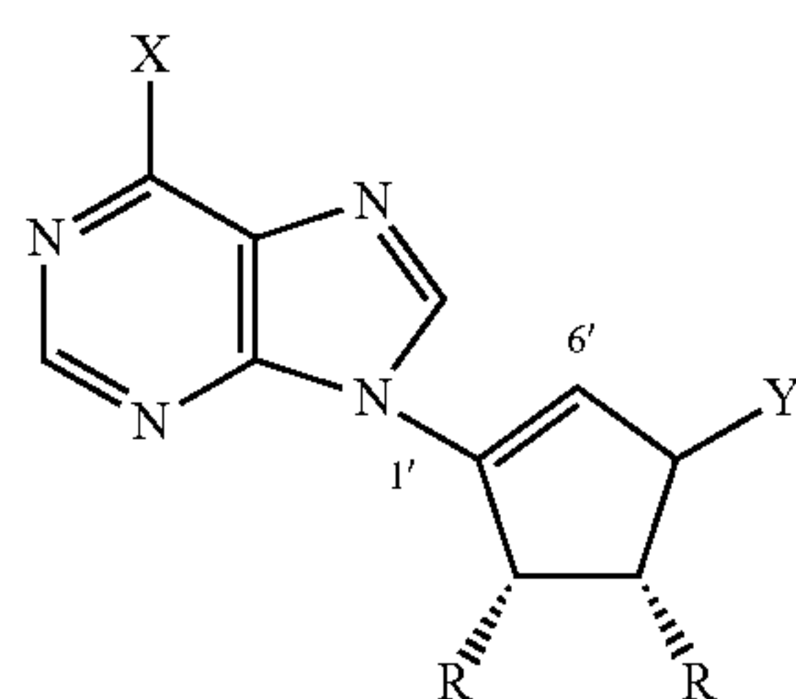
L-isononeplanocin analogue
