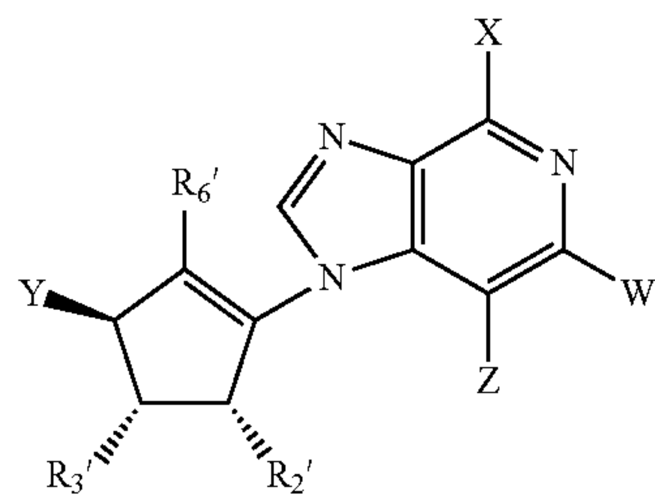
D-3-Deazaisoneplanocin analogue,
