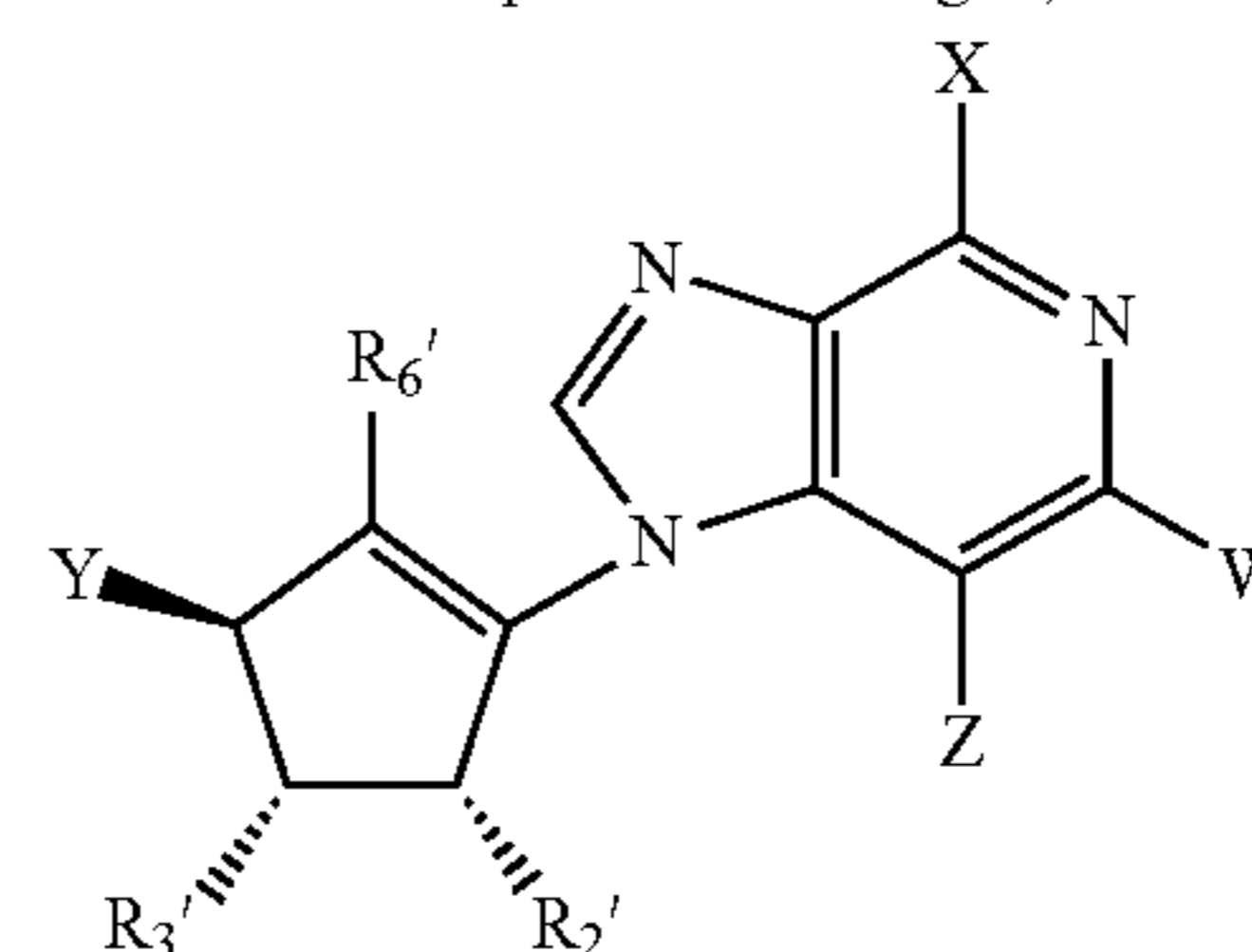
L-isoneplanocin analogue,
