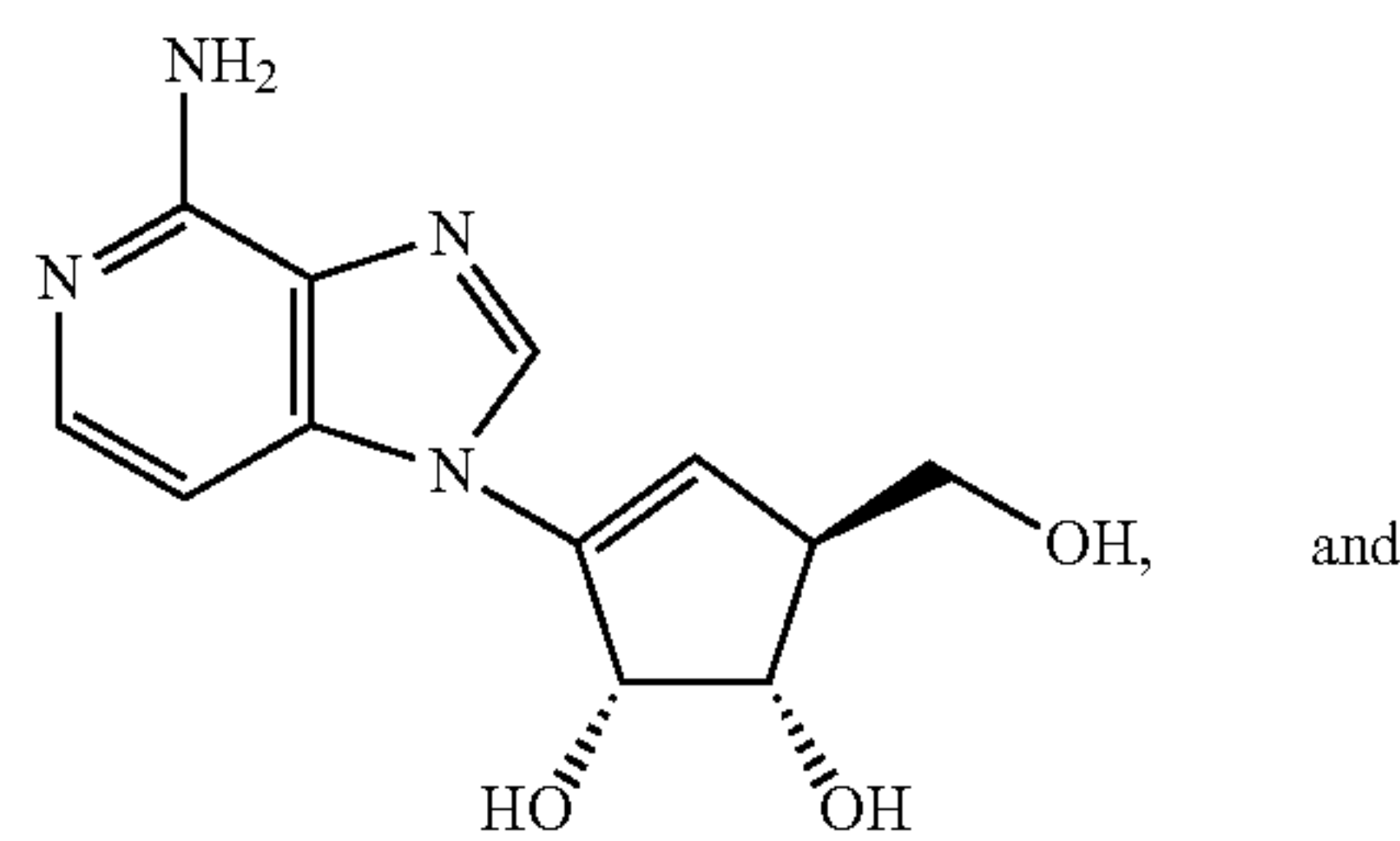
L-3-deazaisoneplanocin
