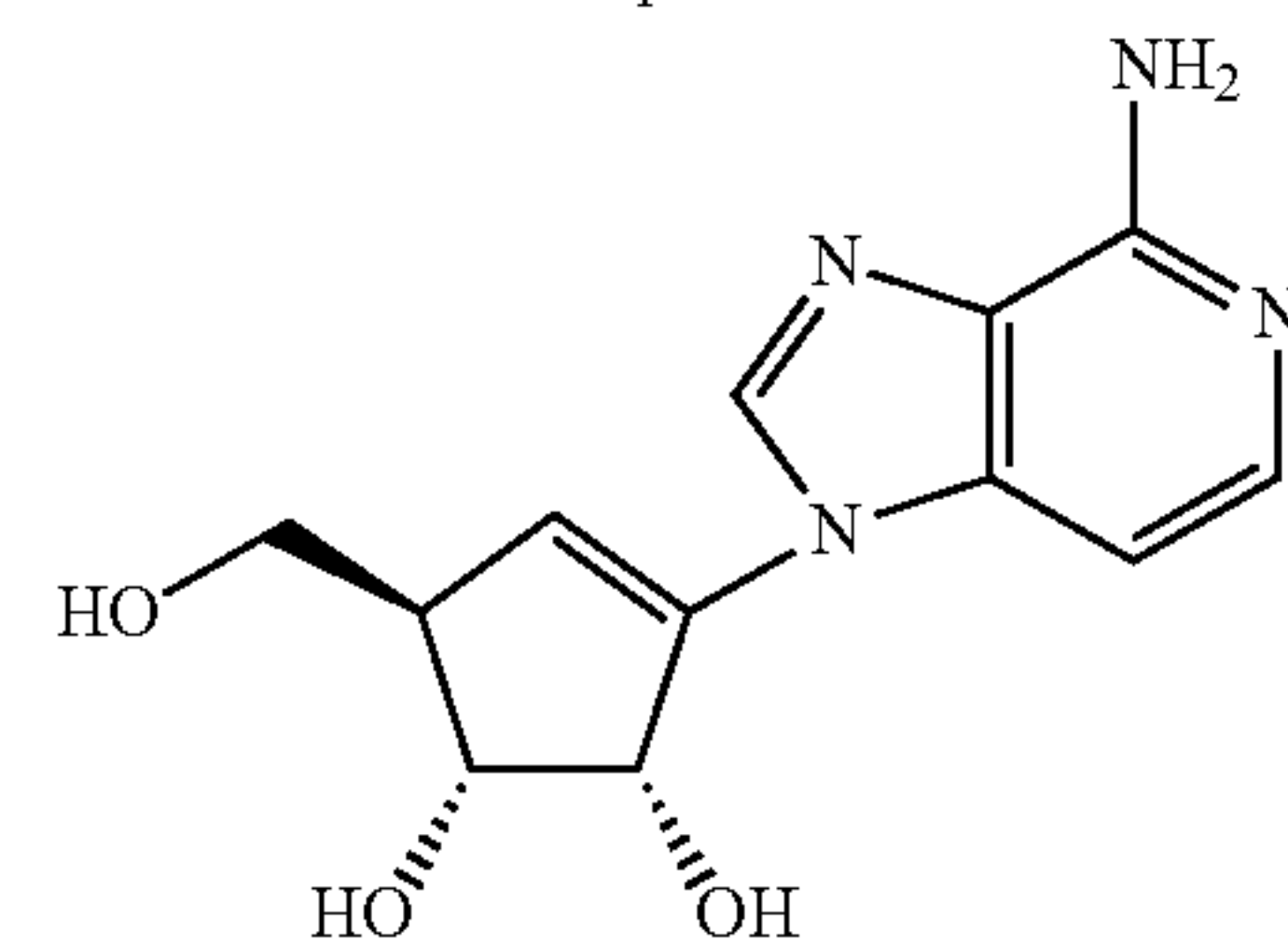
D-3-deazaisoneplanocin
